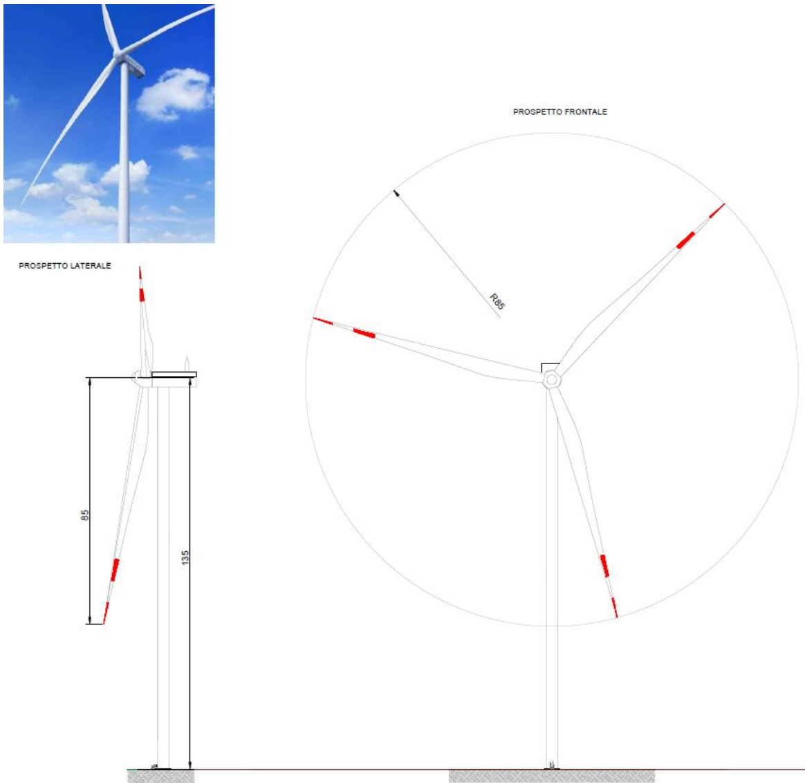
Figura c-1: Struttura aerogeneratore
