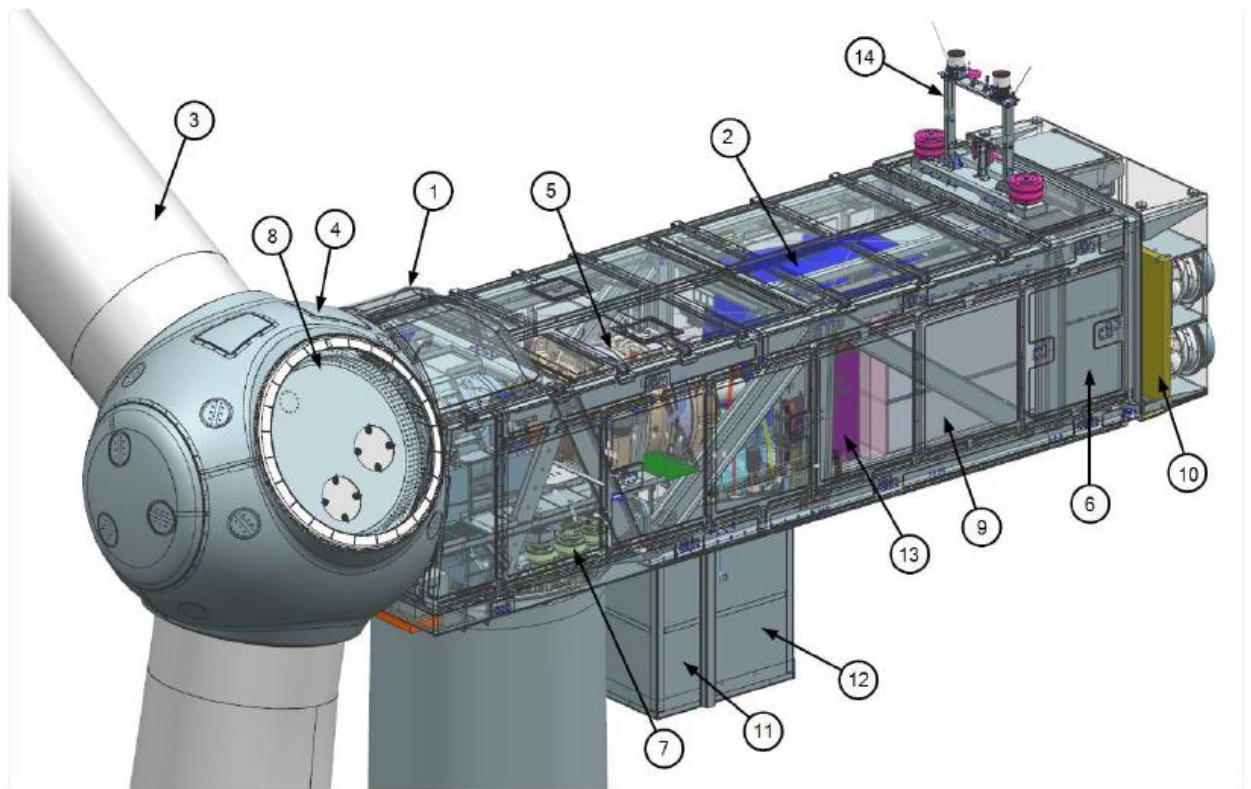
Figura 1 schema descrittivo della navicella Siemens Gamesa SG 6.0-170
