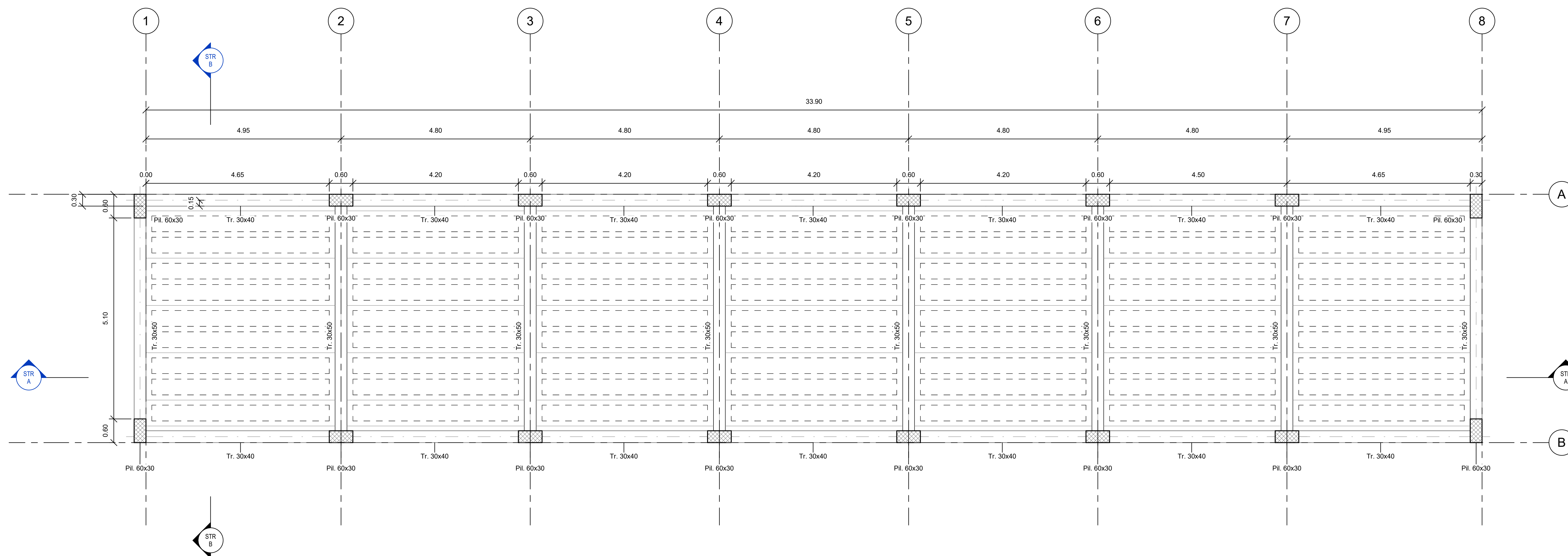
Carpenteria Copertura 1 : 50
