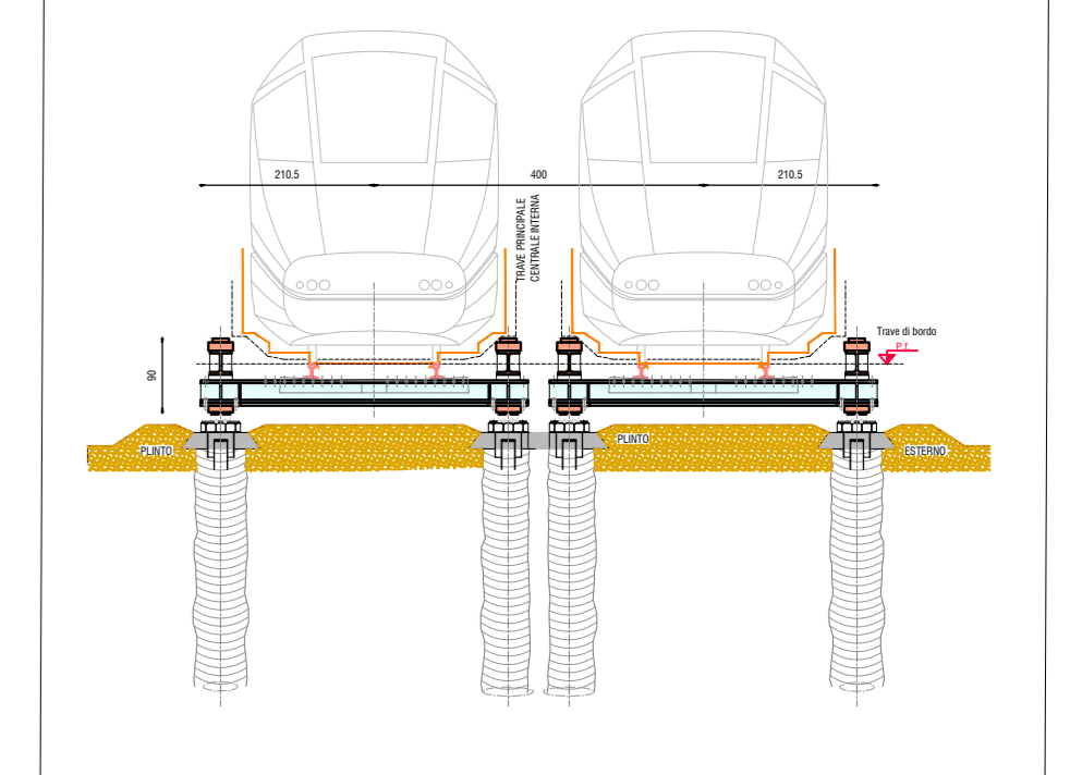
SEZIONE TRASVERSALE - PONTE GUIDO Lc=20,40m (in prossimità appoggi)
