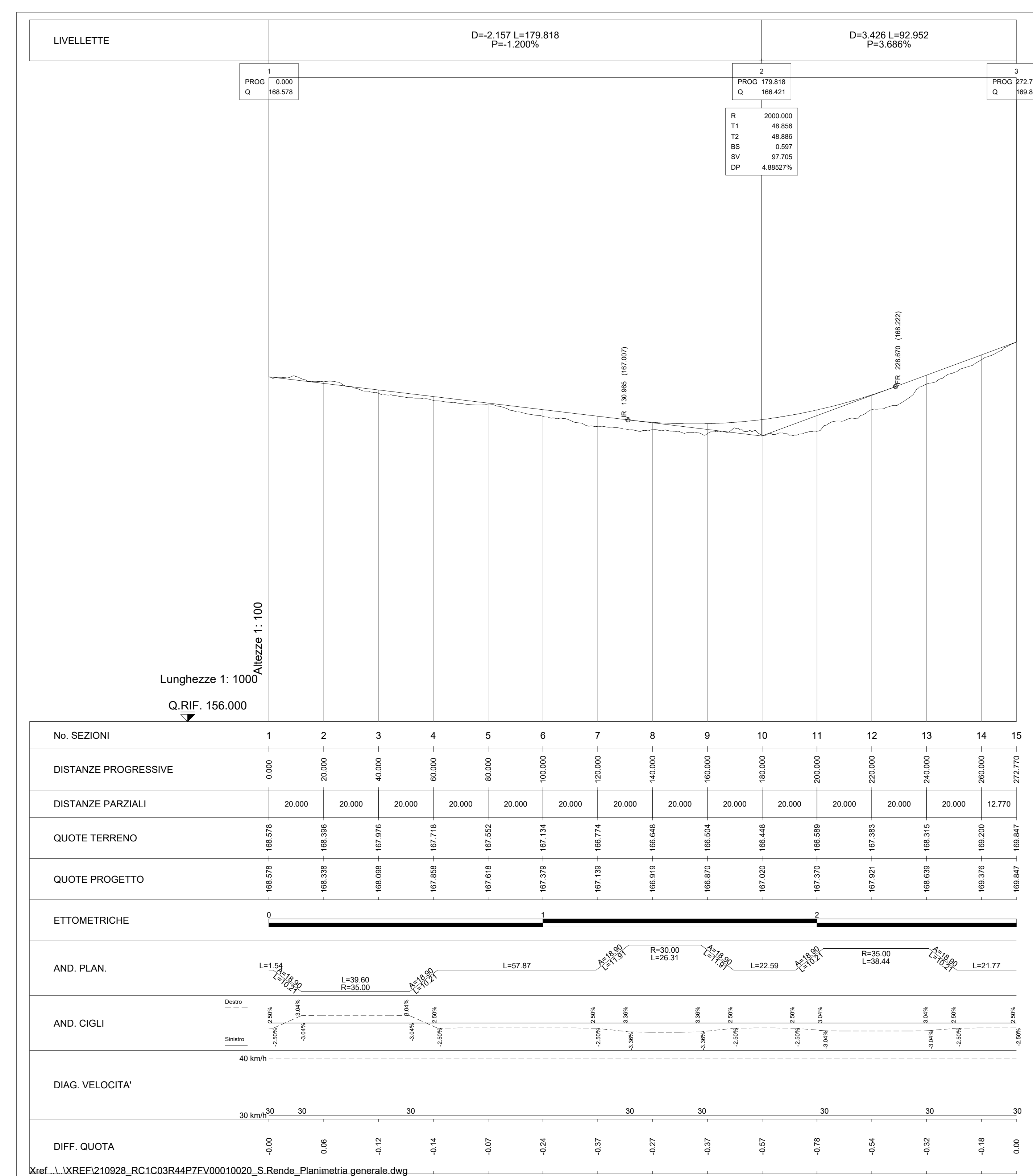
PROFILO NV01 - Scala 1:1000 1:1000
