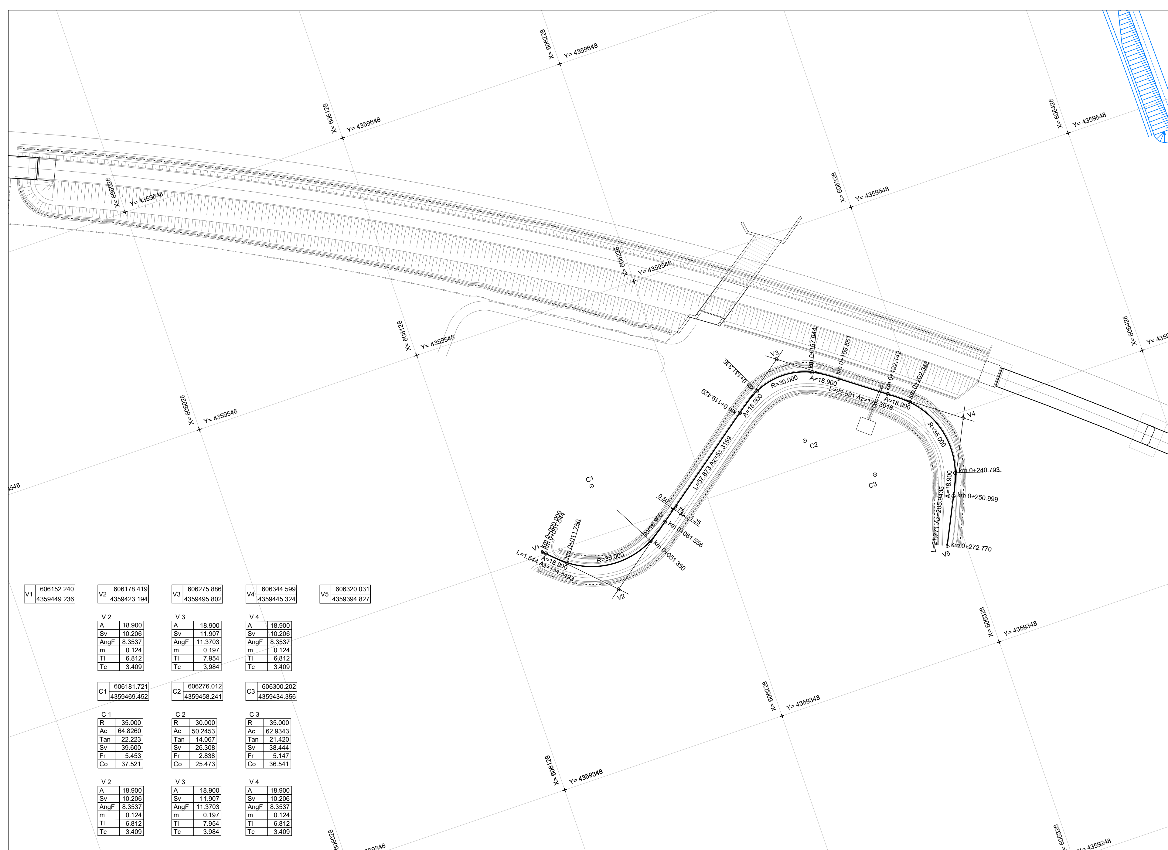
PLANIMETRIA DI TRACCIAMENTO NV01 - Scala 1:1000
