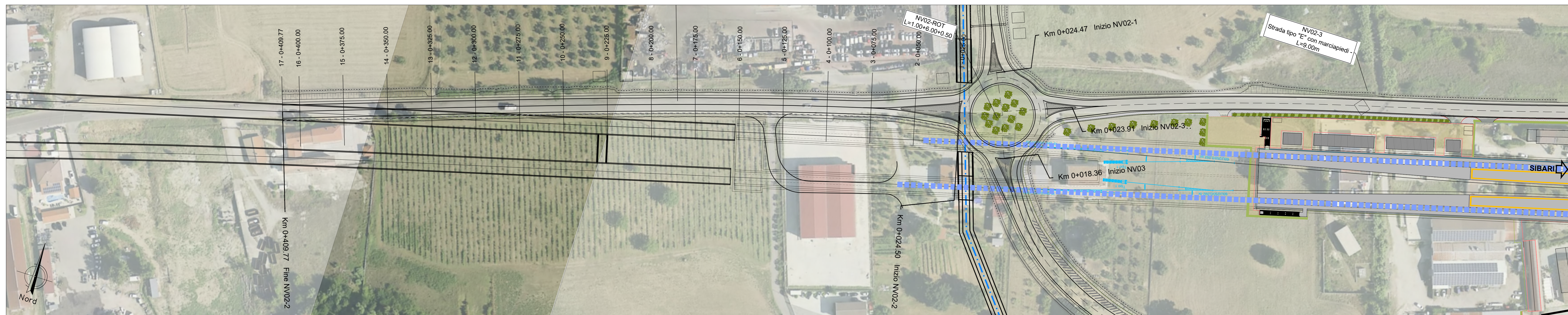
PLANIMETRIA DI PROGETTO NV02-2 - Scala 1:1000
