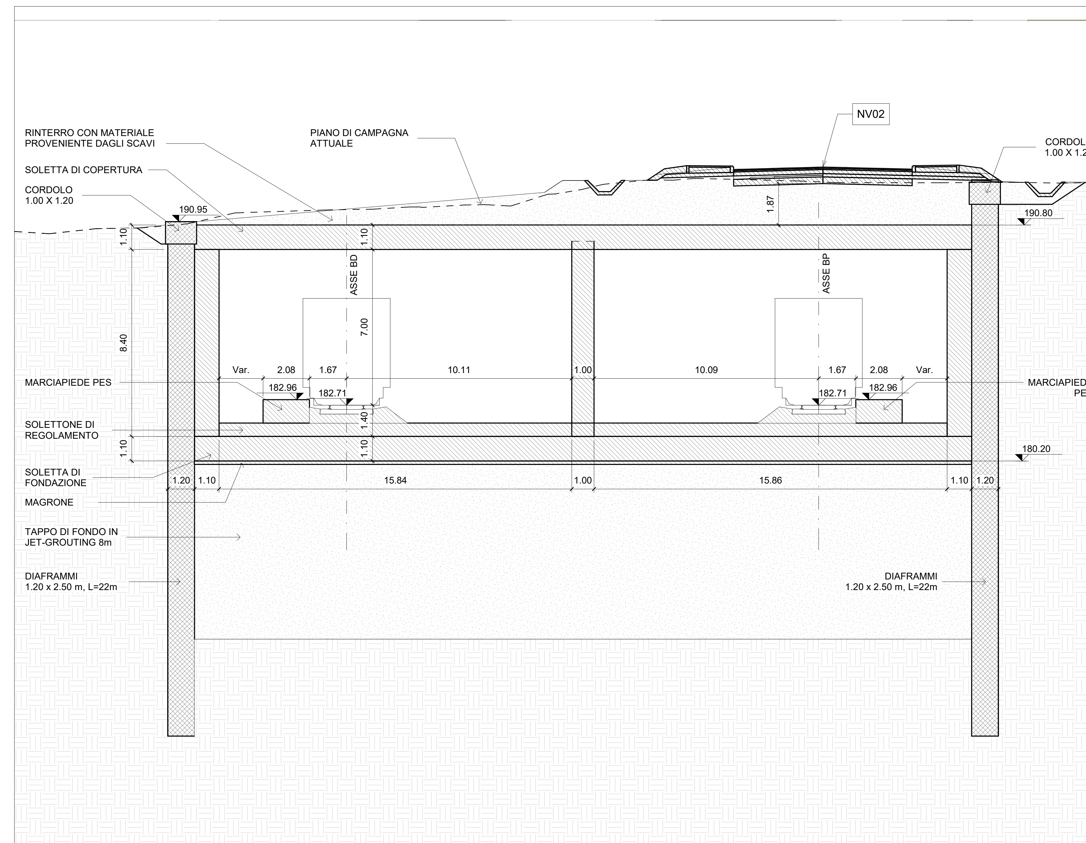
S2 - Sezione Trasversale 1 : 100
