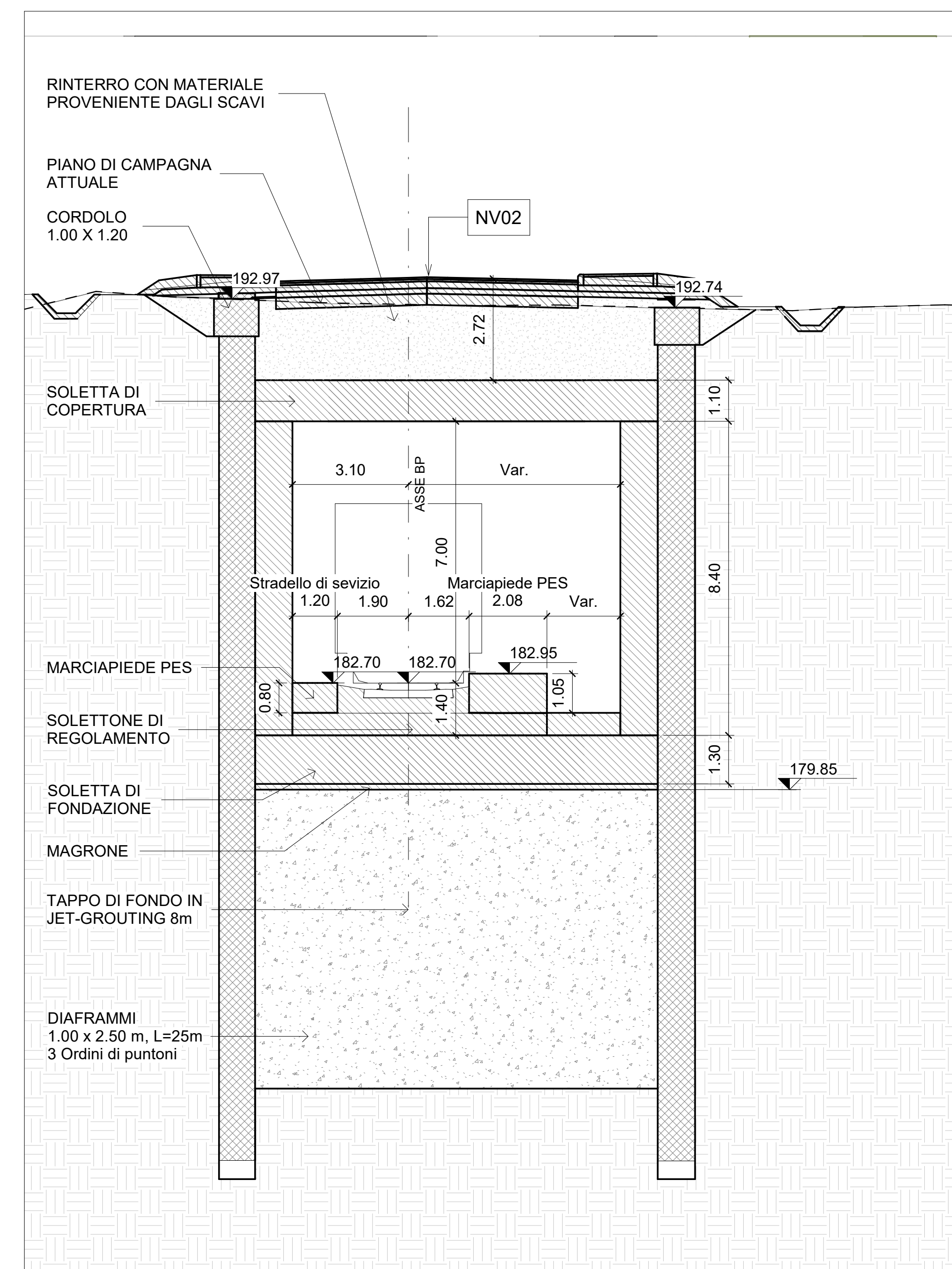
S3 - Sezione Trasversale 1 : 100
