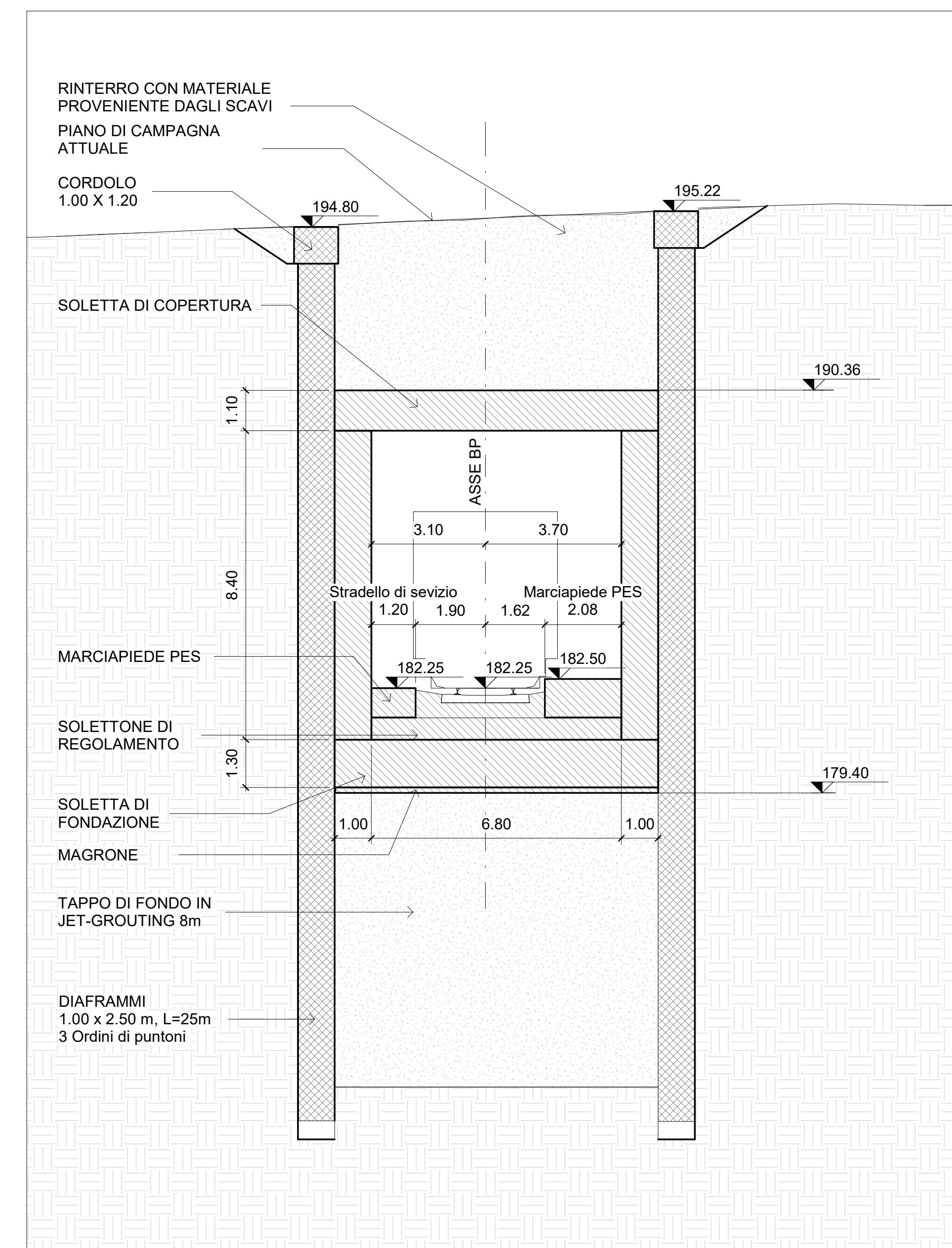
S2 - Sezione Trasversale 1 : 100
