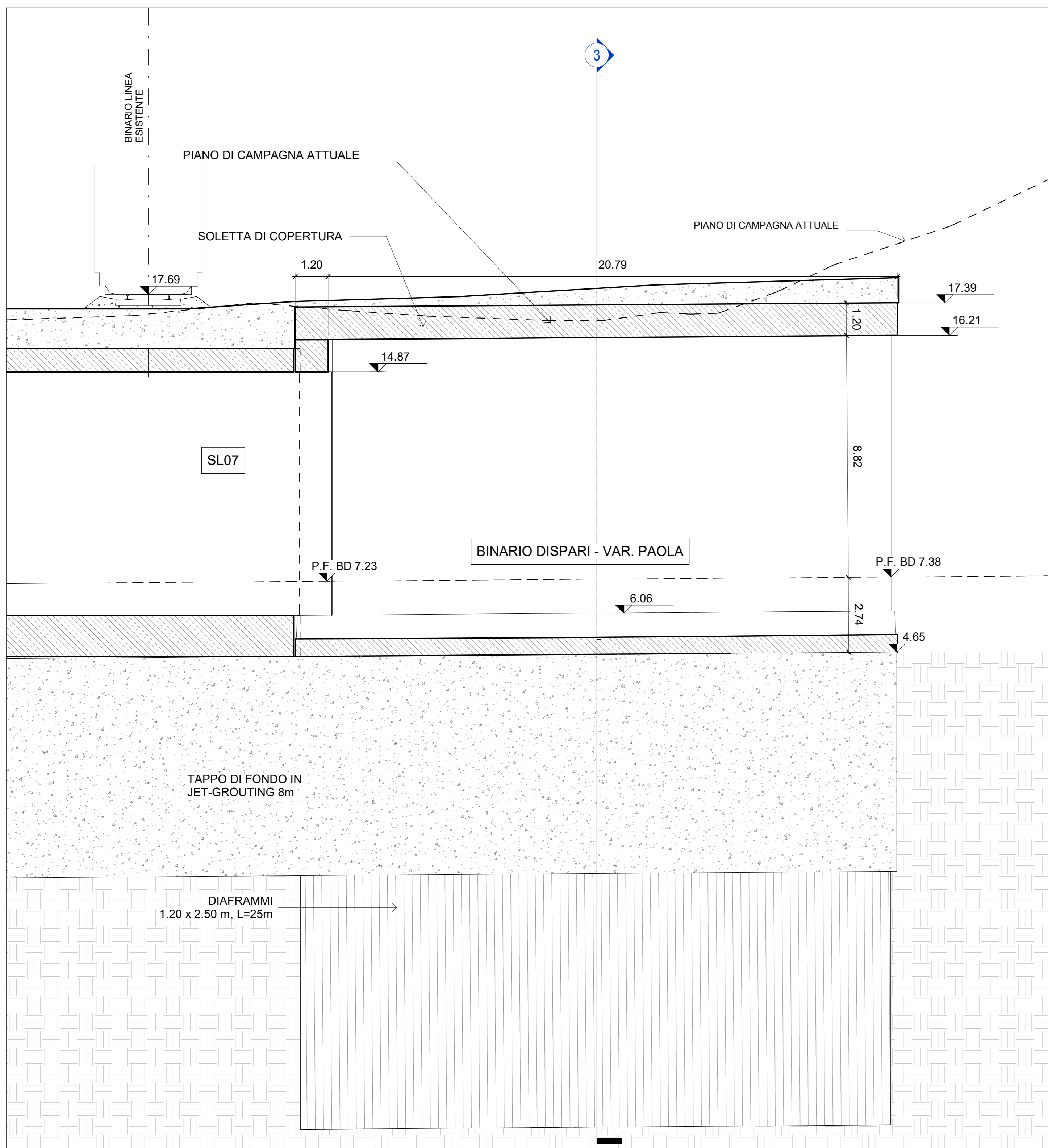
S1 - Sezione Longitudinale 1: 100
