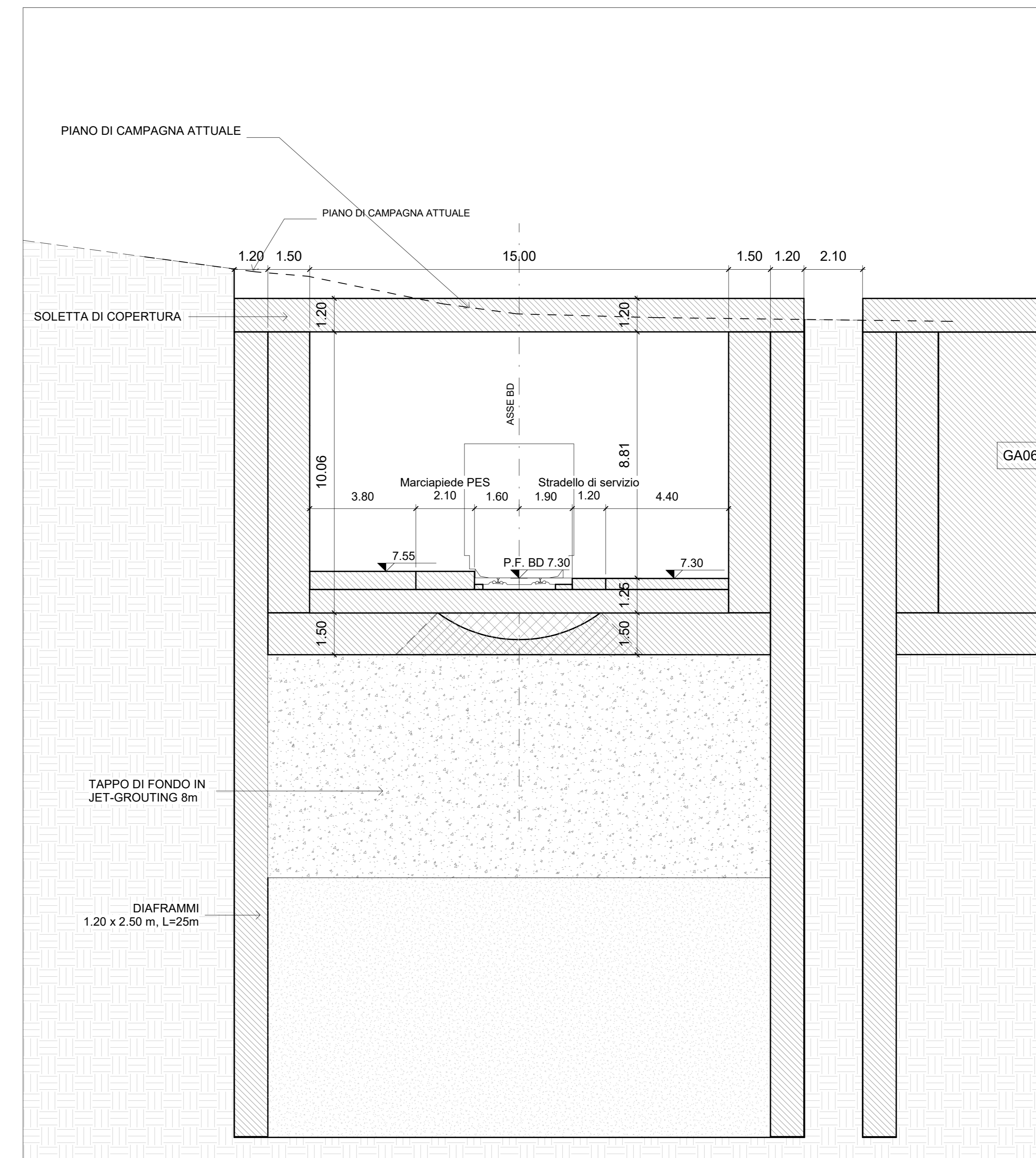
S2 - Sezione Trasversale 1: 100
