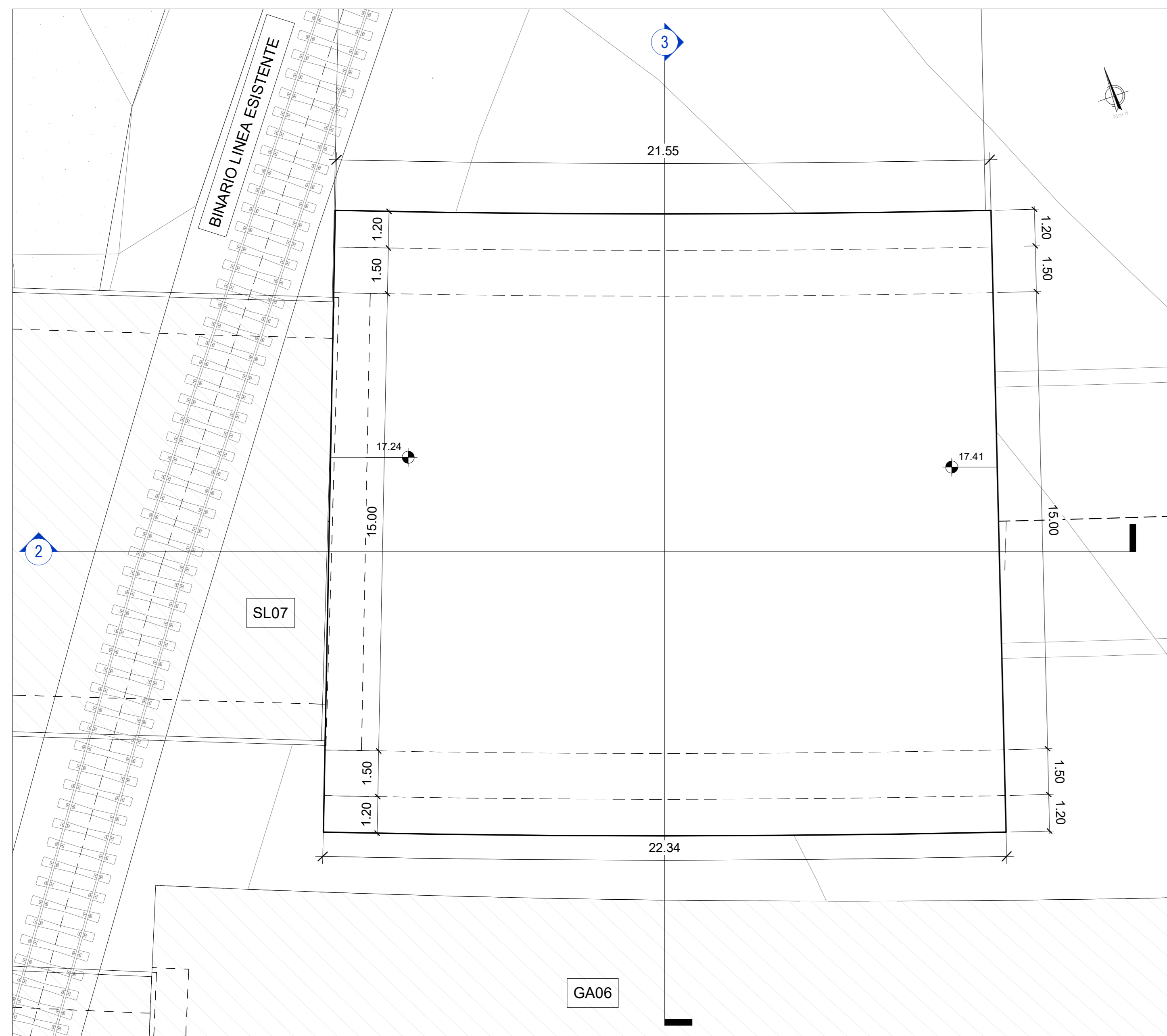
Pianta spiccato 1: 100
