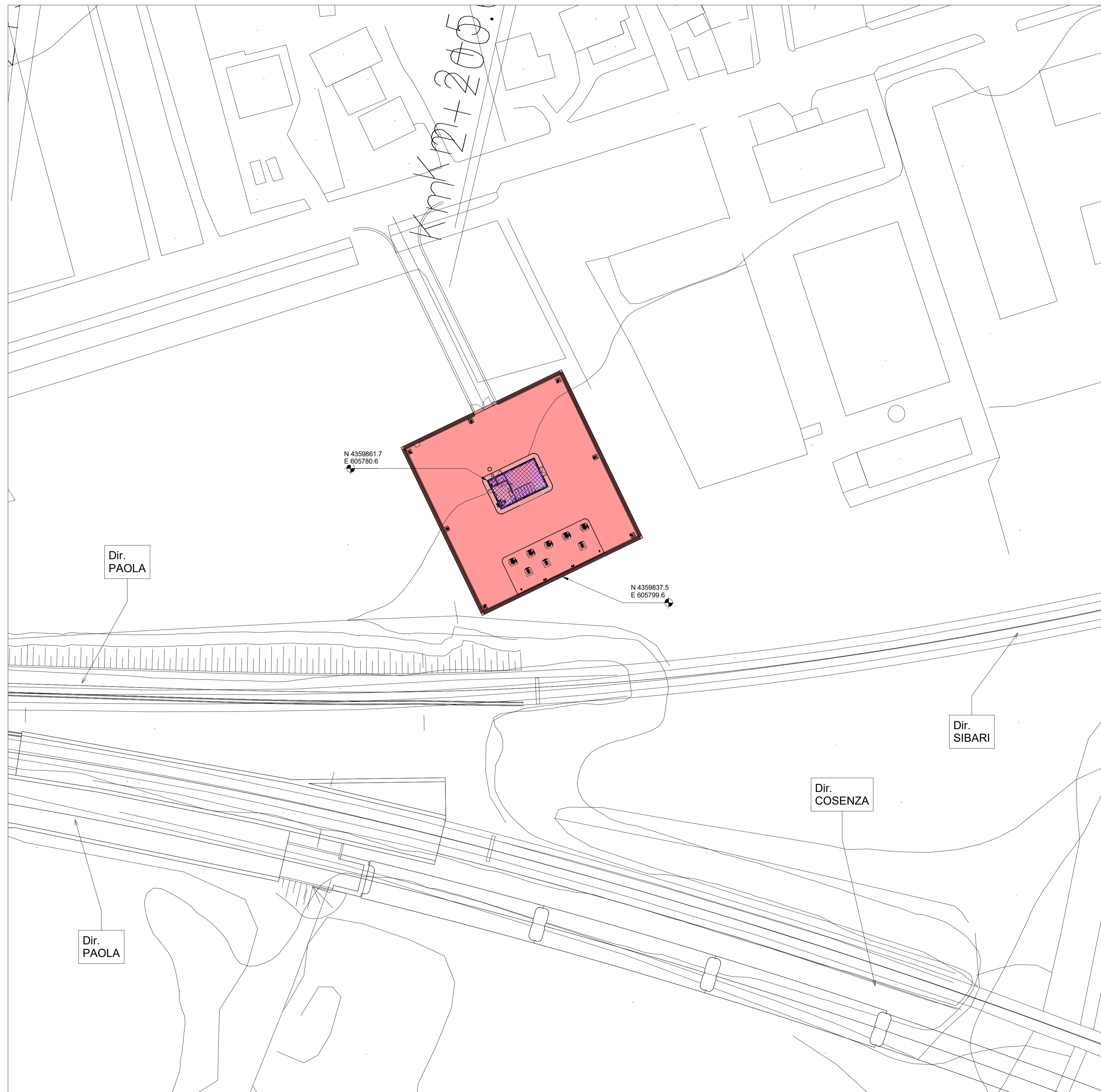
1 Ubicazione impianto 1 : 500
