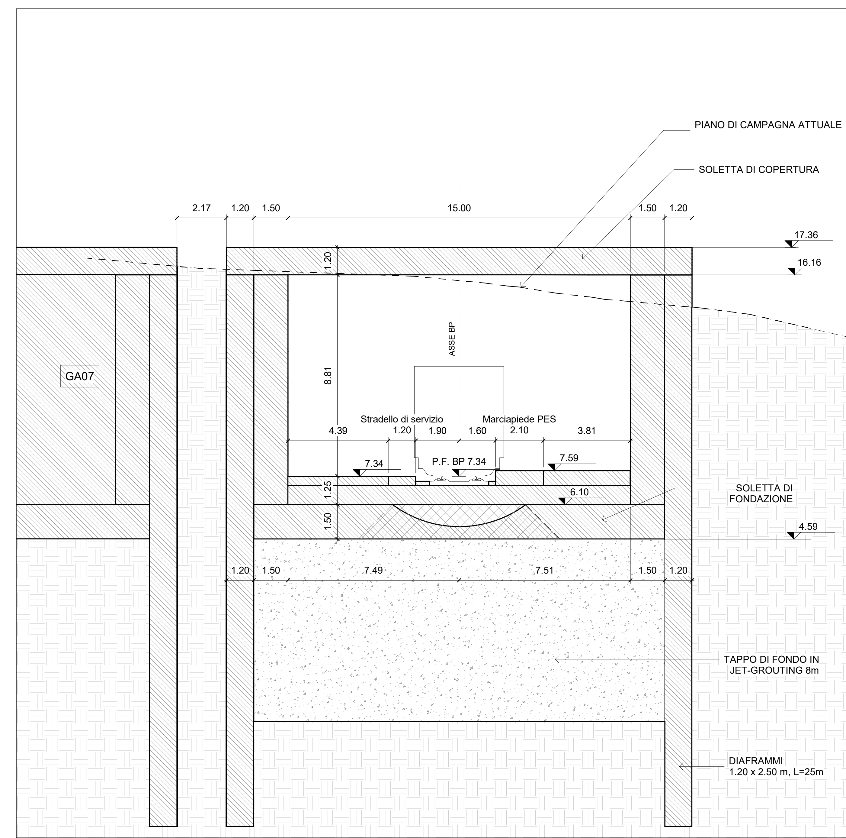
S2 - Sezione Trasversale 1 : 100
