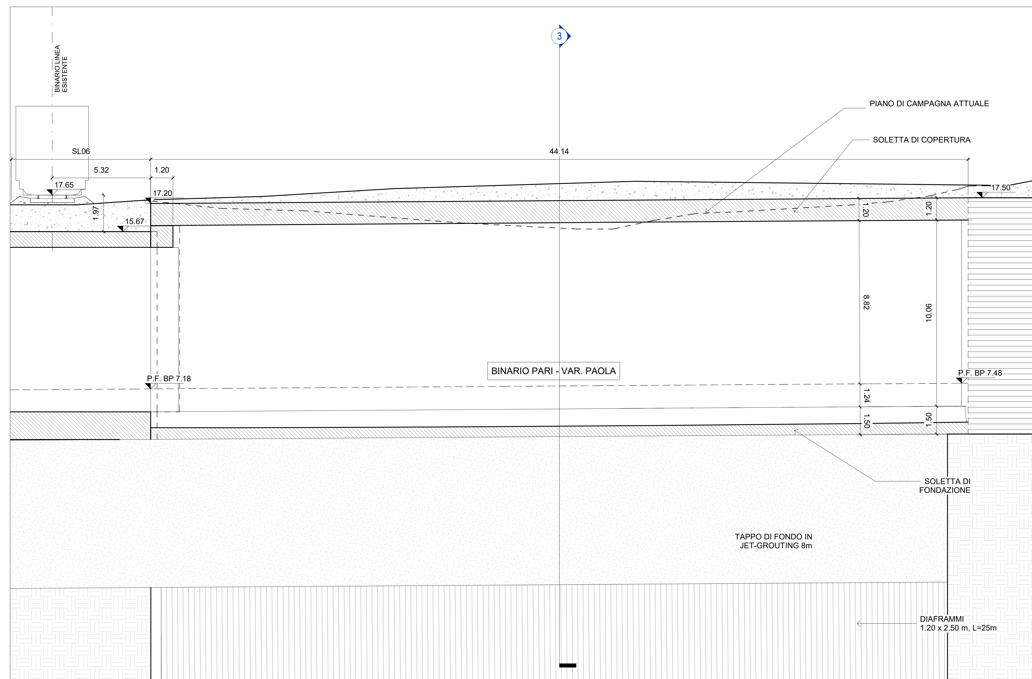
S1 - Sezione Longitudinale 1 : 100
