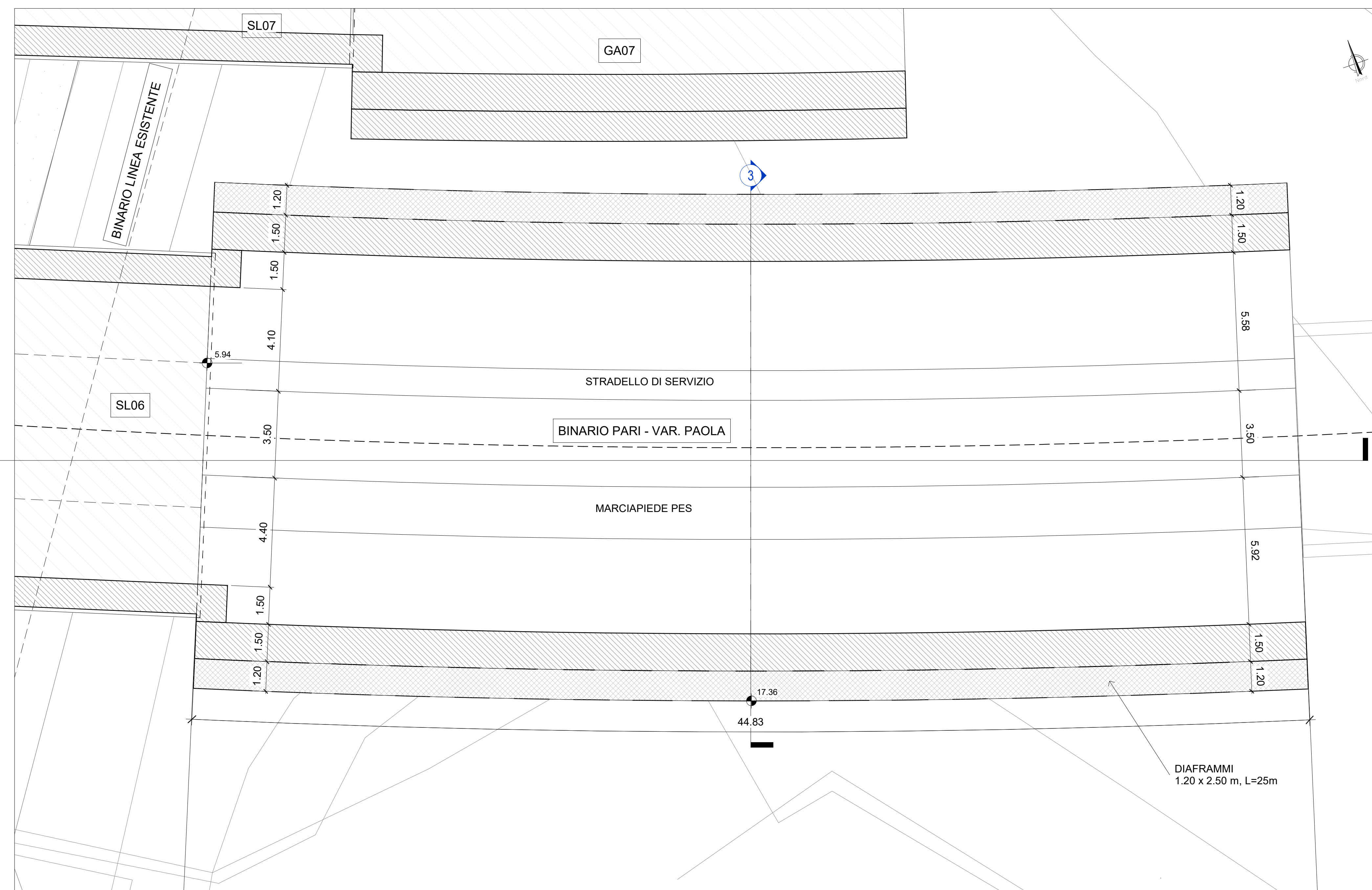
Pianta P.F. 1 : 100
