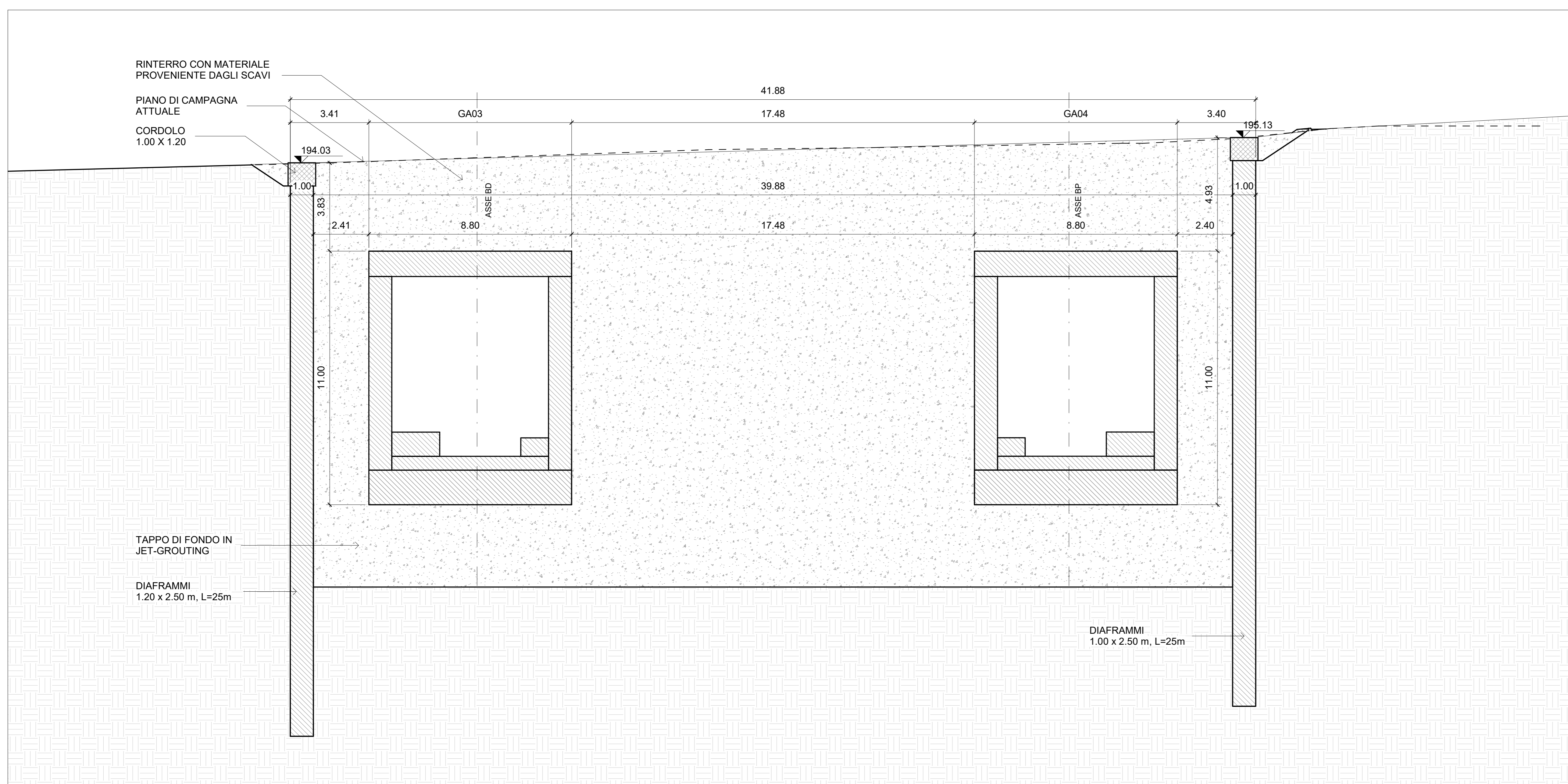
S2 - Sezione Trasversale 1 : 100
