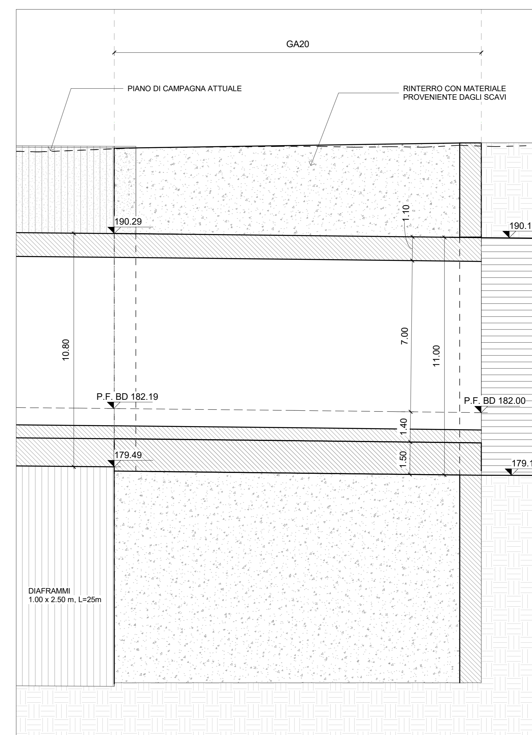
S1 - Sezione Longitudinale 1 : 100
