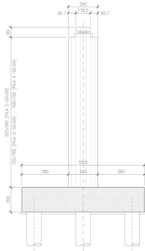
VISTA LATERALE PILE P.2-P.3-P.4 CARPENTERIA
