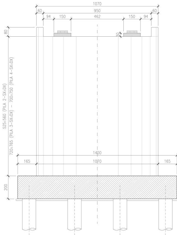
FIGURA 3-7: CARPENTERIA PILE 2-3-4.
