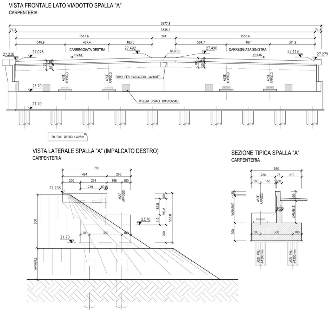
FIGURA 3-9: CARPENTERIA SPALLA A.
