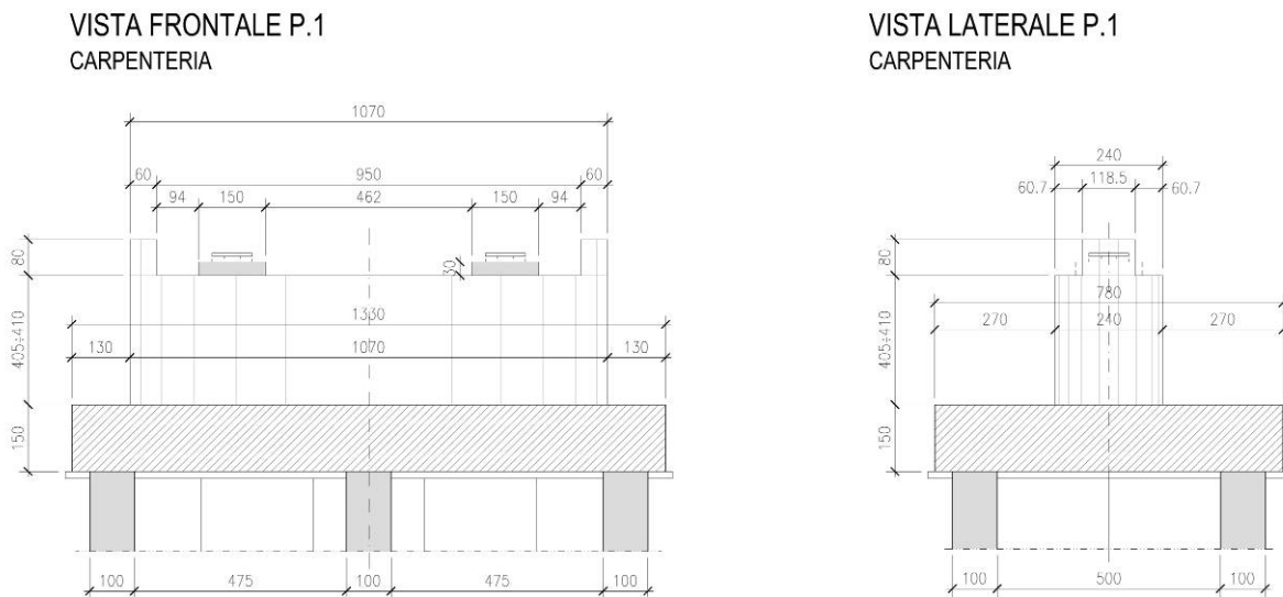
FIGURA 3-6: CARPENTERIA PILA 1.
