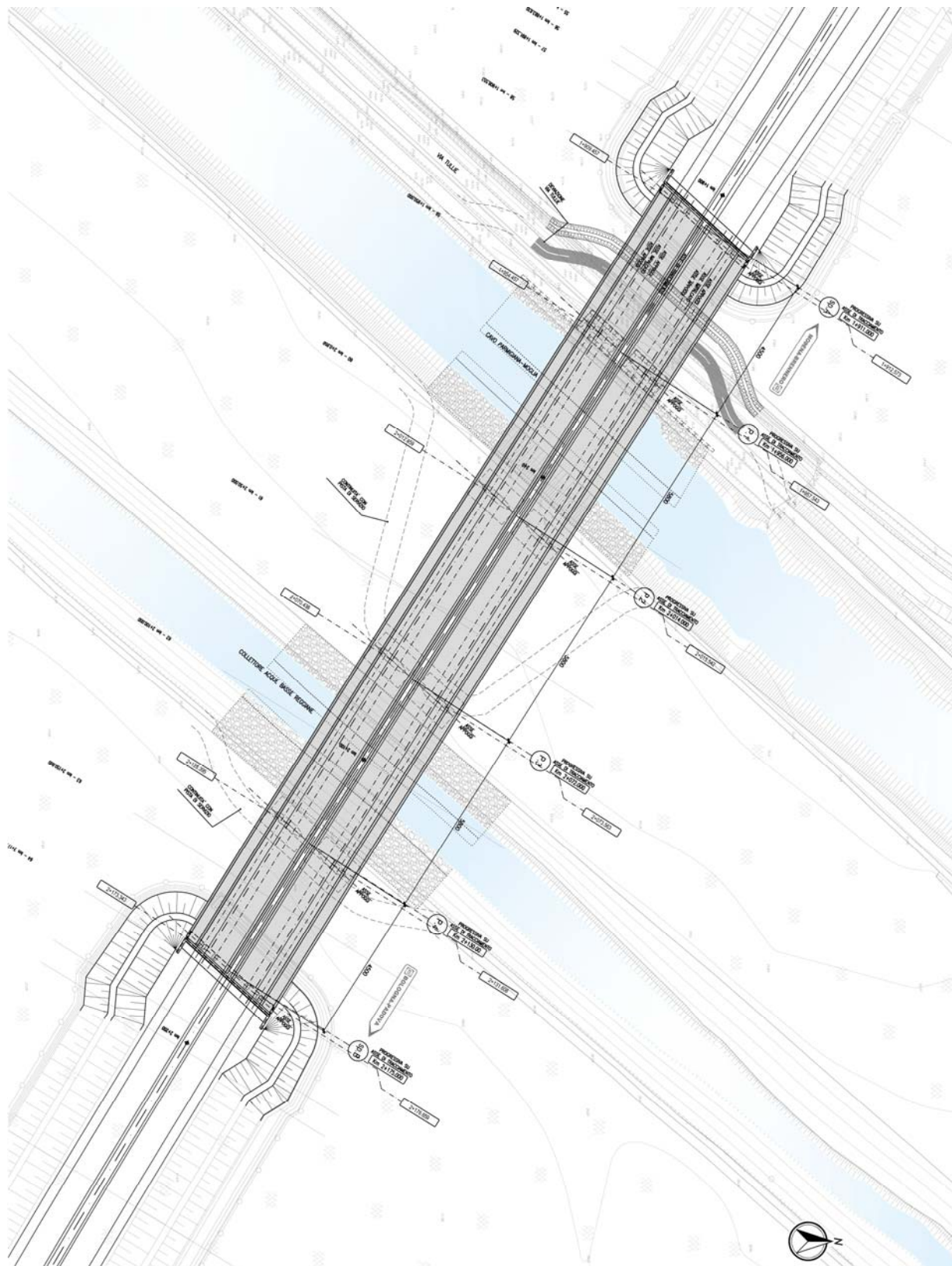
FIGURA 3-1: PLANIMETRIA.
