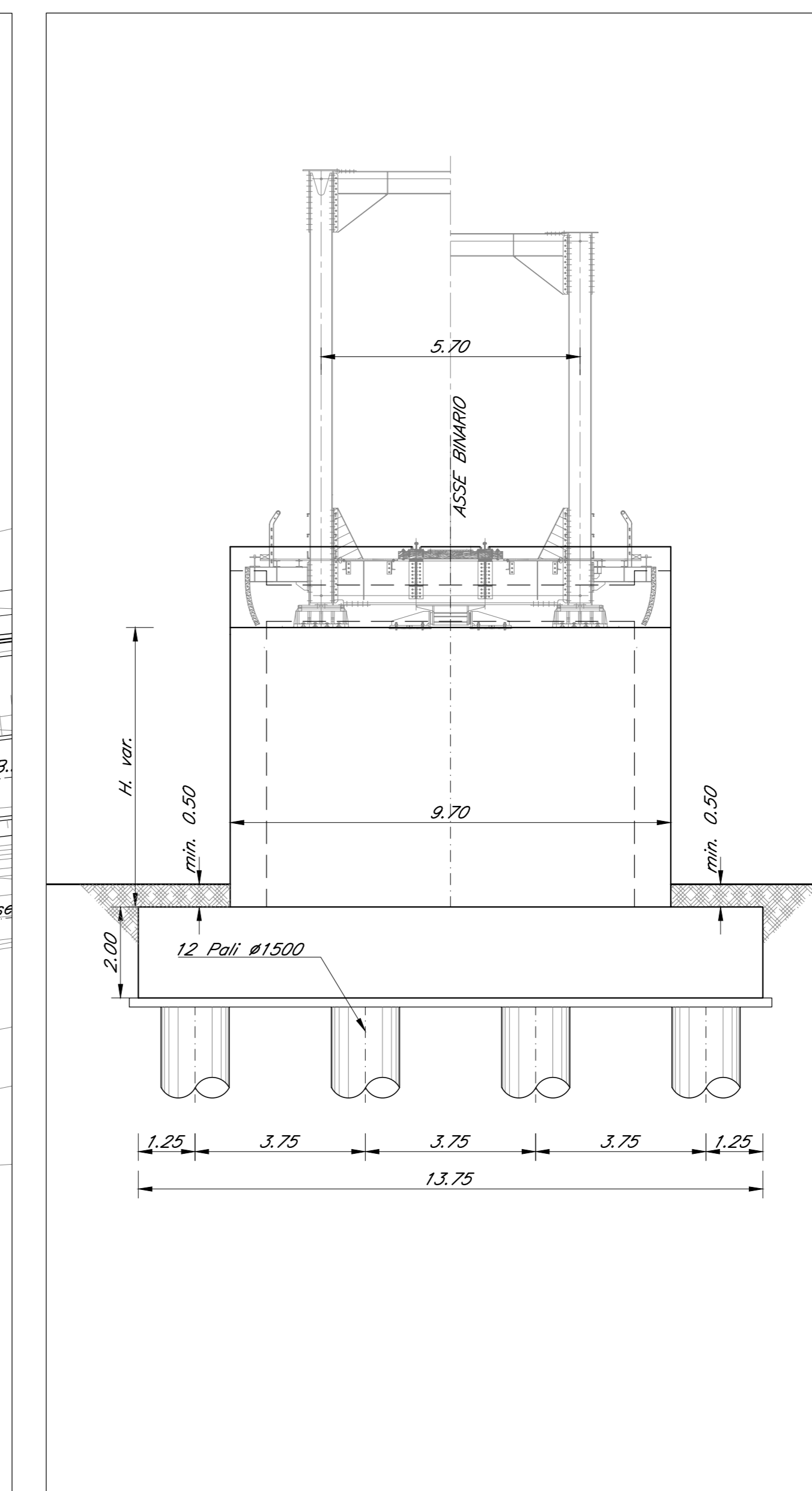
SEZIONE TRASVERSALE SPALLA TIPO Scala 1:100
