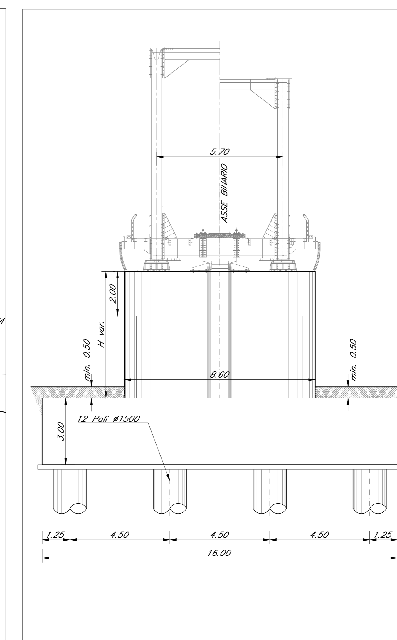
SEZIONE TRASVERSALE PILA TIPO Scala 1:100
