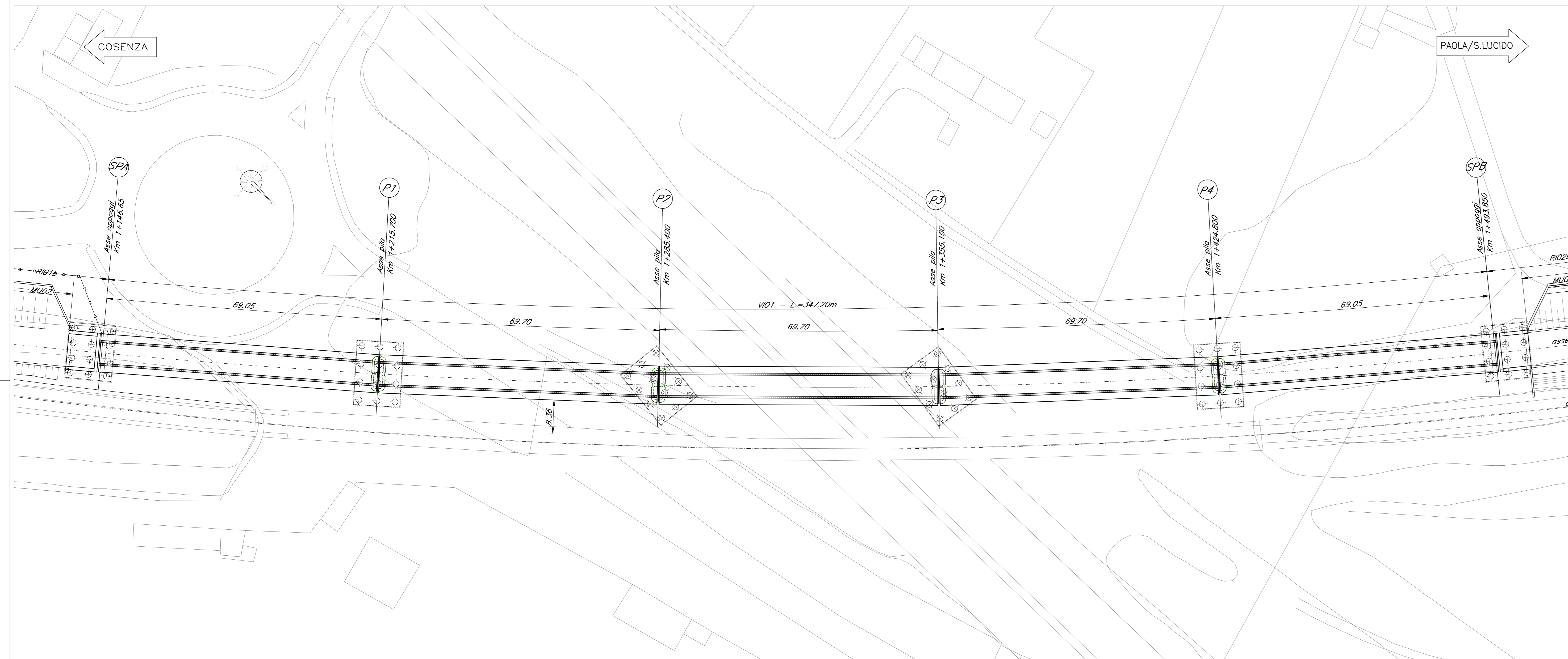
PIANTA IMPALCATO Scala 1:500
