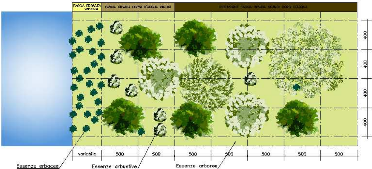
Figura 4-4 – MODULO D – Sistemazione vegetazione spondale: sesto d'impianto e sezione tipologica
