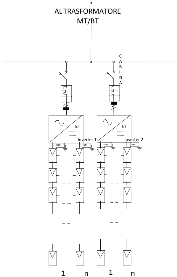
Figura 1: schema unifilare tipo di principio dell'impianto fotovoltaico.
