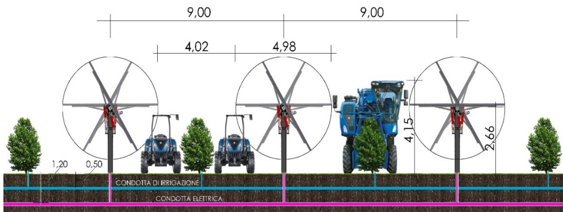
Sezione tipo impianto integrato
