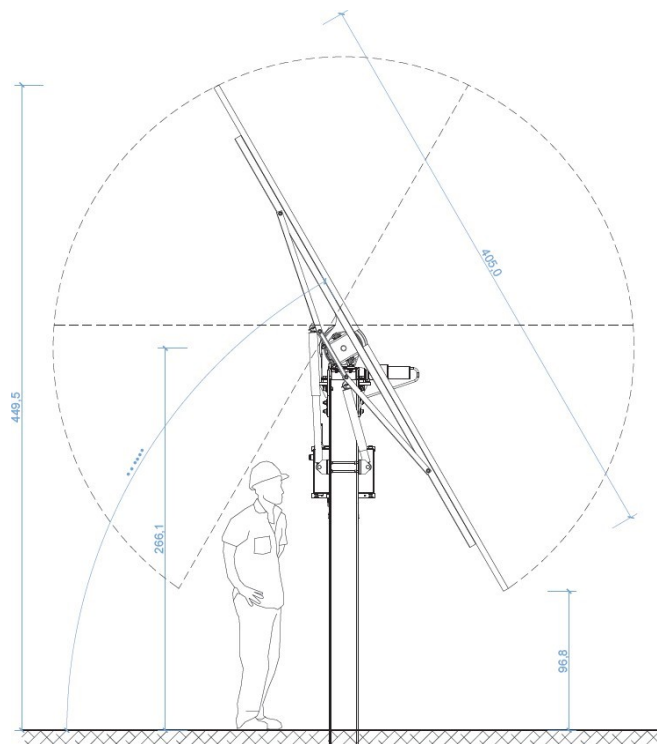
Sezione tipo del Tracker
