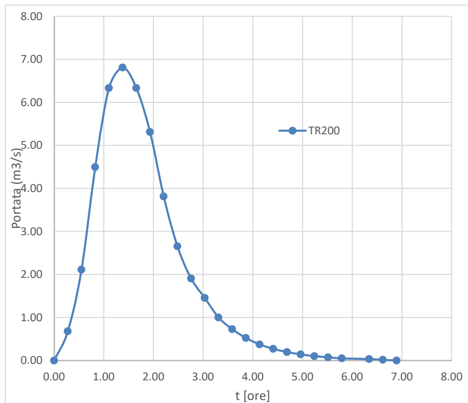
Grafico 10 - Idrogramma di Mockus nei tre tempi di ritorno TR200 – Bacino 3
