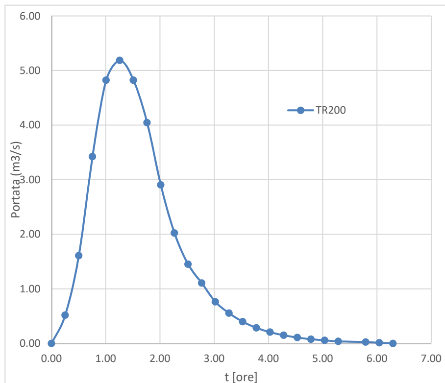
Grafico 8 - Idrogramma di Mockus nei tre tempi di ritorno TR200 – Bacino 1
