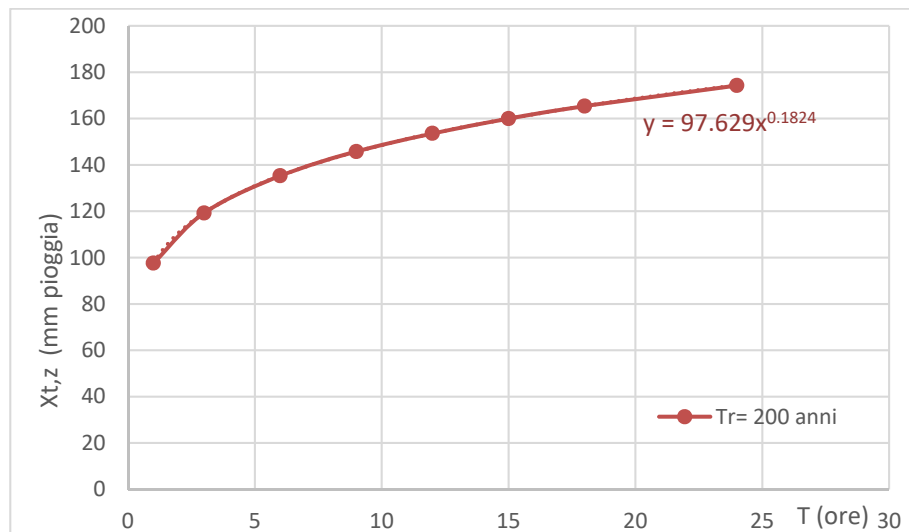
Grafico 3 - Curve di possibilità pluviometrica per 200 – Bacino 4
