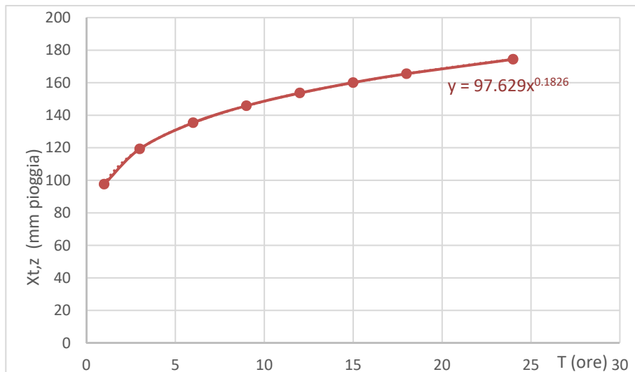
Grafico 6 - Curve di possibilità pluviometrica per Tr 30, 200 e 500 – Bacino C e Bacino F
