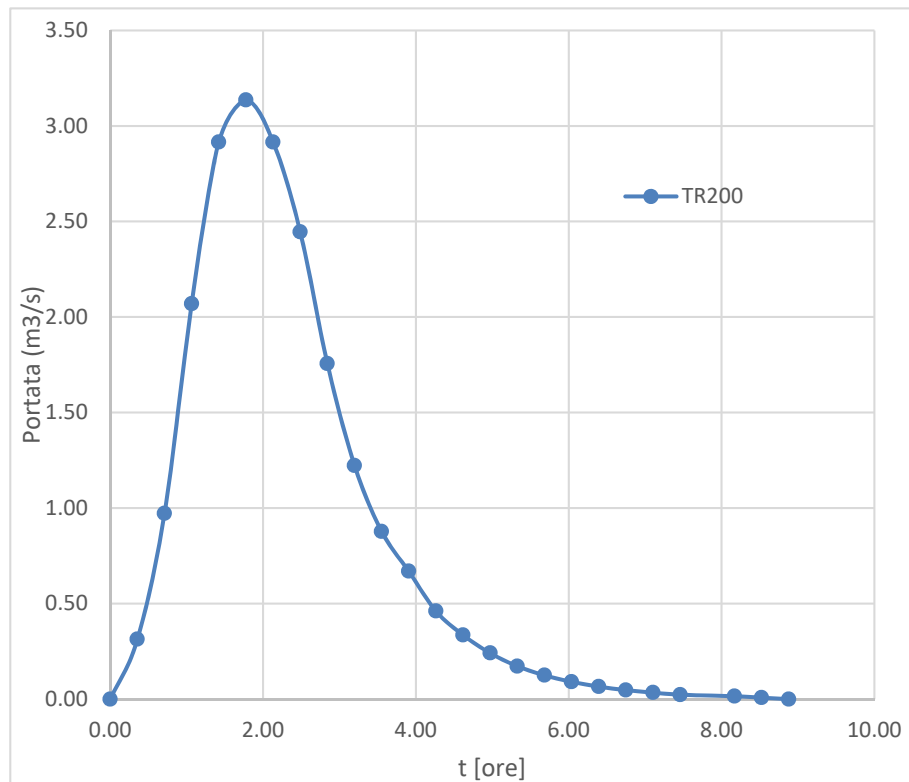
Grafico 16 - Idrogramma di Mockus TR200 – Bacino D
