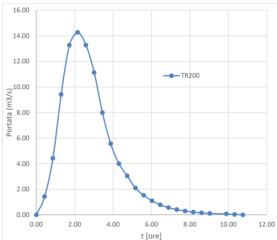
Grafico 17 - Idrogramma di Mockus TR200 – Bacino E
