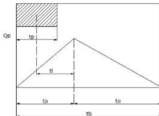
Grafico 7 - Idrogramma di Mockus
