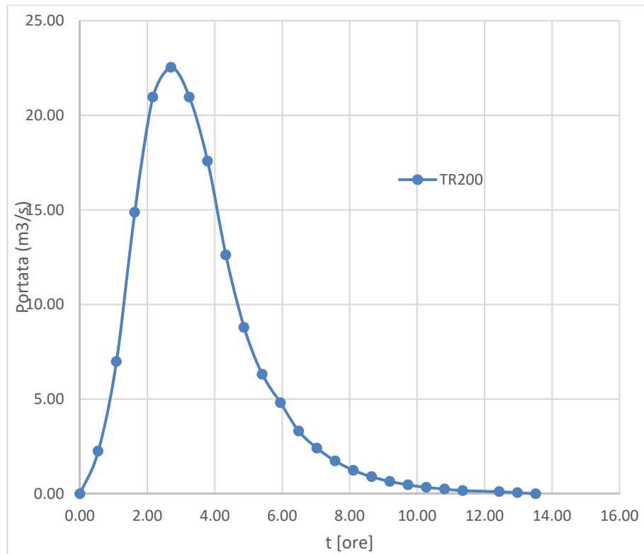
Grafico 11 - Idrogramma di Mockus nei tre tempi di ritorno TR200 – Bacino 4
