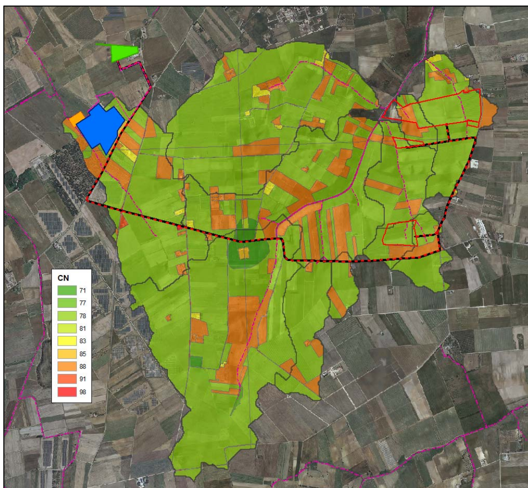
Figura 6 - Mappatura delle aree con CN omogeneo
