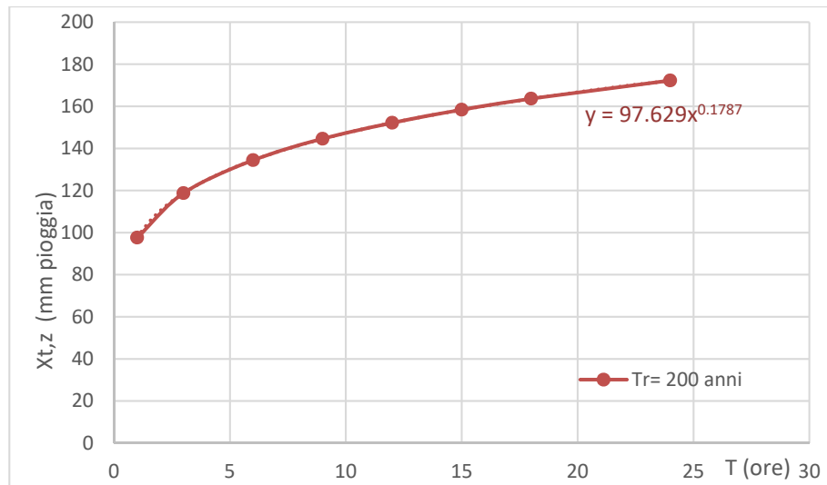
Grafico 2 - Curve di possibilità pluviometrica per 200 – Bacino 3
