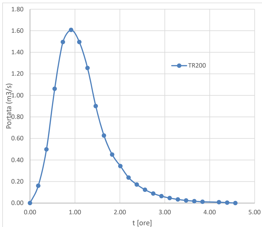
Grafico 14 - Idrogramma di Mockus TR200 – Bacino B
