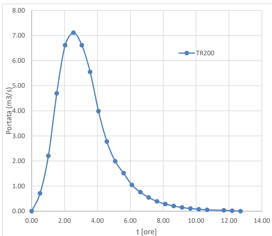
Grafico 18 - Idrogramma di Mockus TR200 – Bacino F
