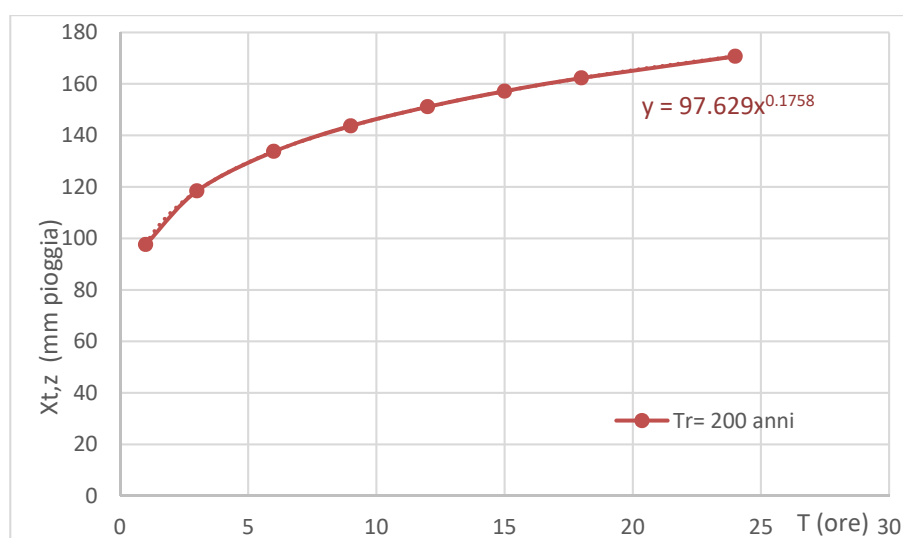
Grafico 1 - Curve di possibilità pluviometrica per 200 – Bacini 1 e 2
