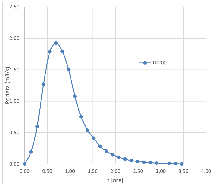
Grafico 15 - Idrogramma di Mockus TR200 – Bacino C
