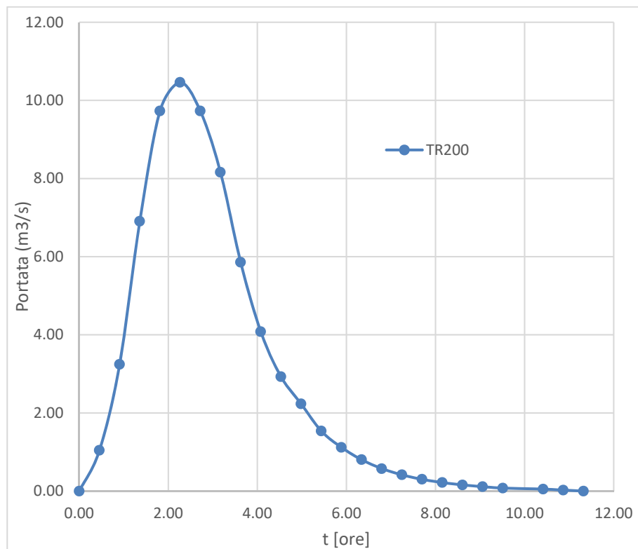
Grafico 12 - Idrogramma di Mockus TR200 - Bacino 5
