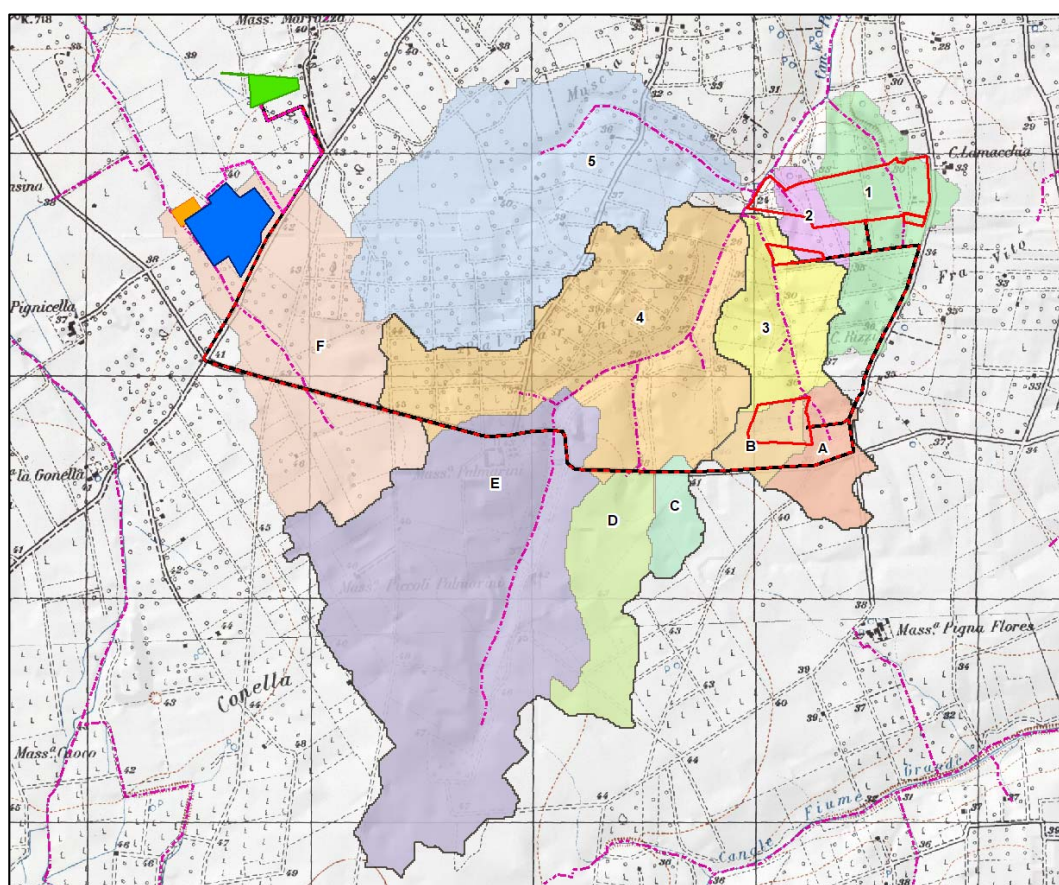
Figura 4 - Bacini idrografici afferenti all’area di studio
