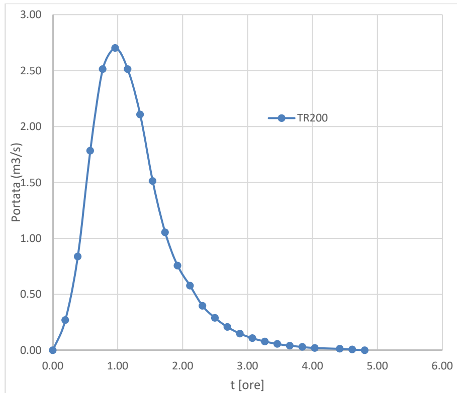
Grafico 13 - Idrogramma di Mockus TR200 – Bacino A
