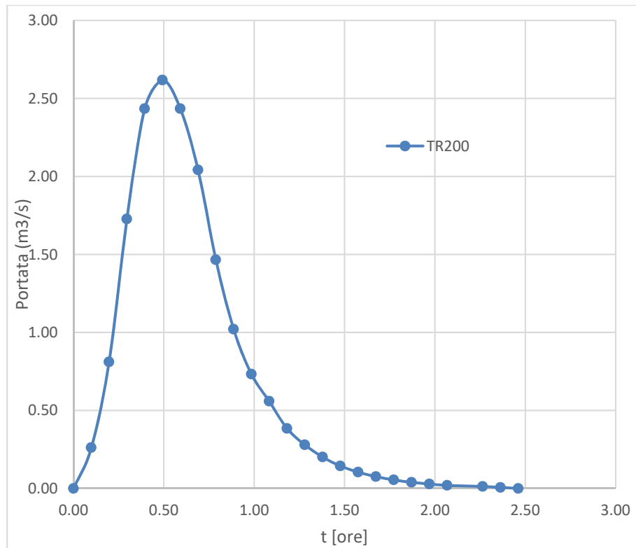
Grafico 9 - Idrogramma di Mockus nei tre tempi di ritorno TR200 – Bacino 2
