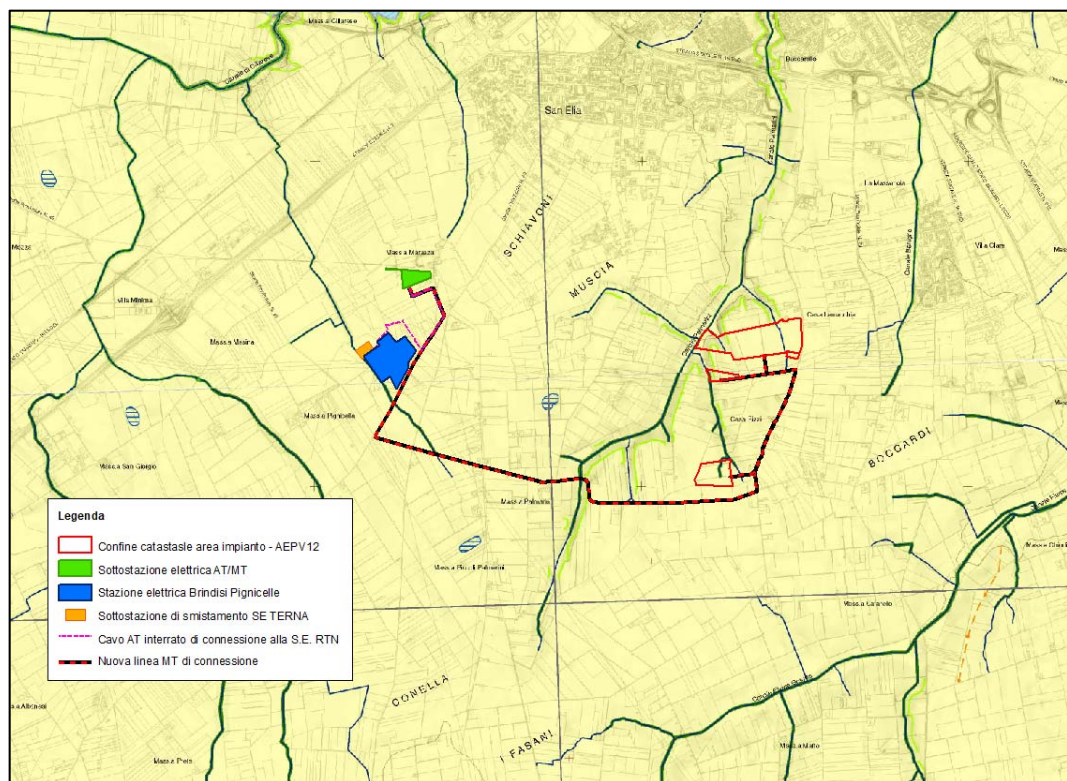
Figura 3 - Estratto della Carta Idrogeomorfológica della Regione Puglia - Foglio 476 "Brindisi" e 495 "Mesagne"
