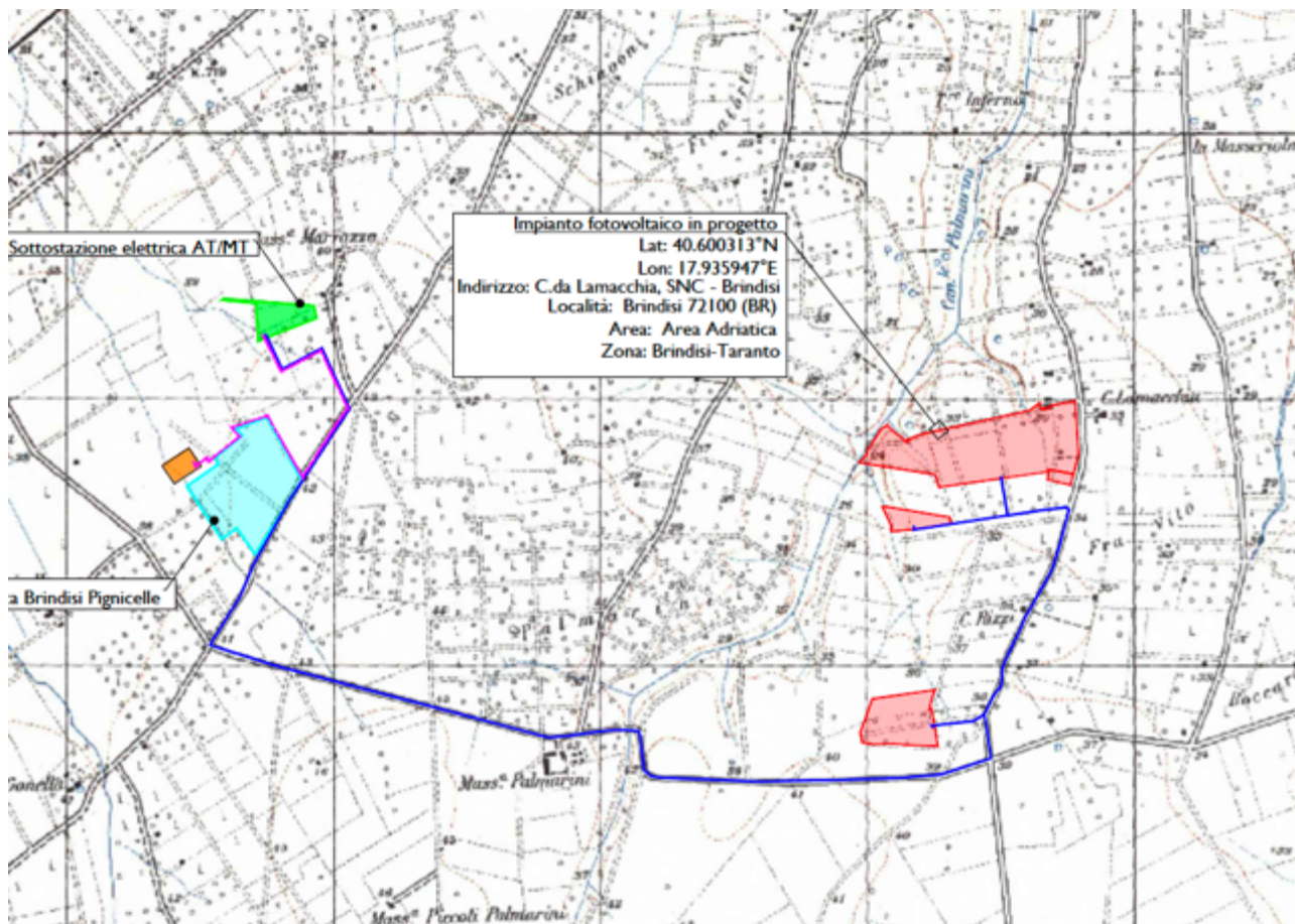
Tavola n. 5 : rappresentazione dei collegamenti previsti per l'impianto.
