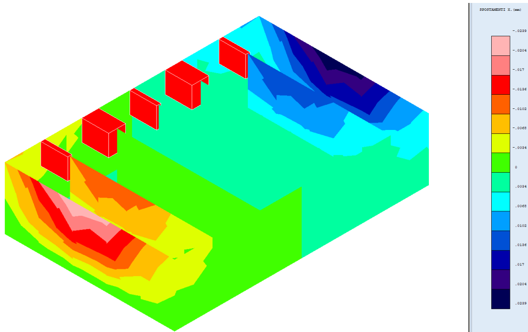
STATO DEFORMATIVO
