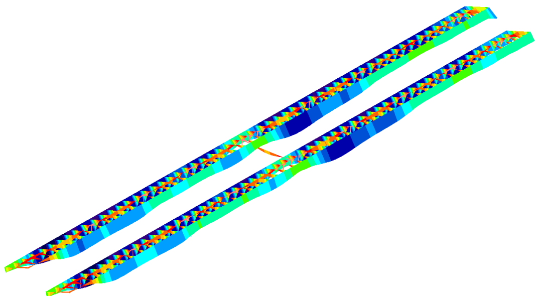
DIAGRAMMA SPOSTAMENTI COMB.5 (SISMA)
