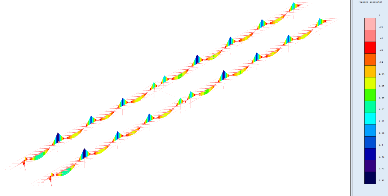
DIAGRAMMA SOLLECITAZIONI MX-MY COMB.1
