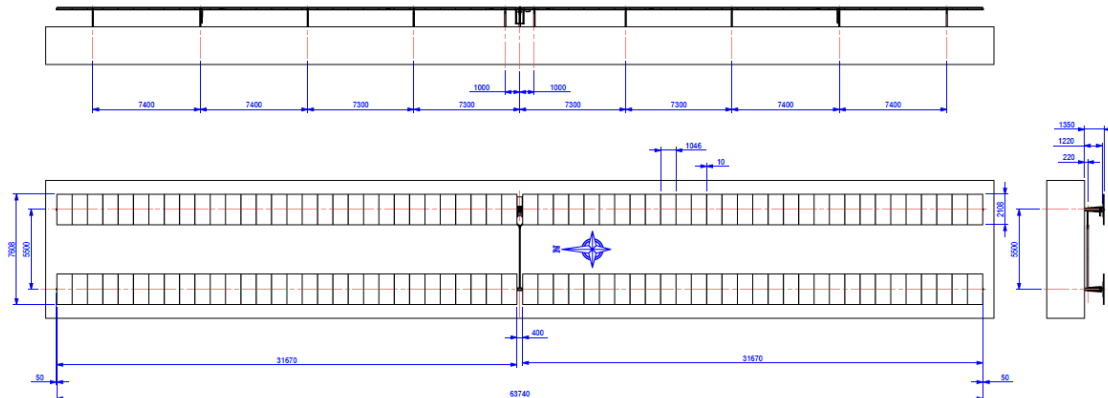
Fig.3 - Schema della struttura – vista longitudinale
