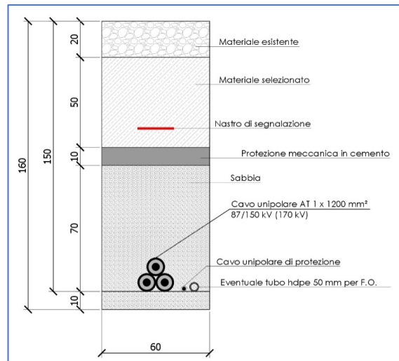
Figura 1 - Tipologico scavo per cavo AT
