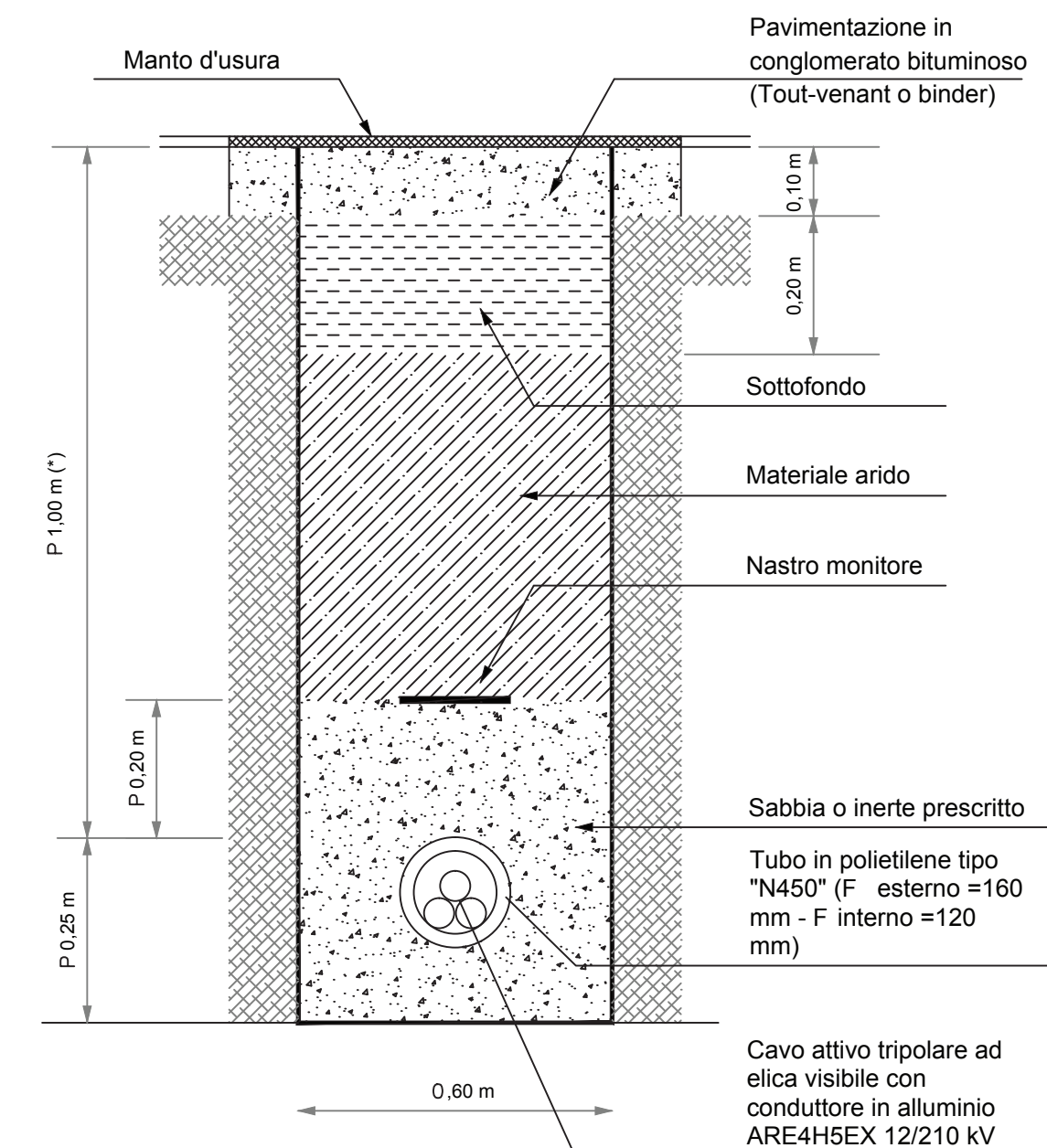
LINEA IN CAVO SOTTERRANEO IN TUBAZIONE POSA DI N.1 CAVI MT IN STRADA COMUNALE ASFALTATA
