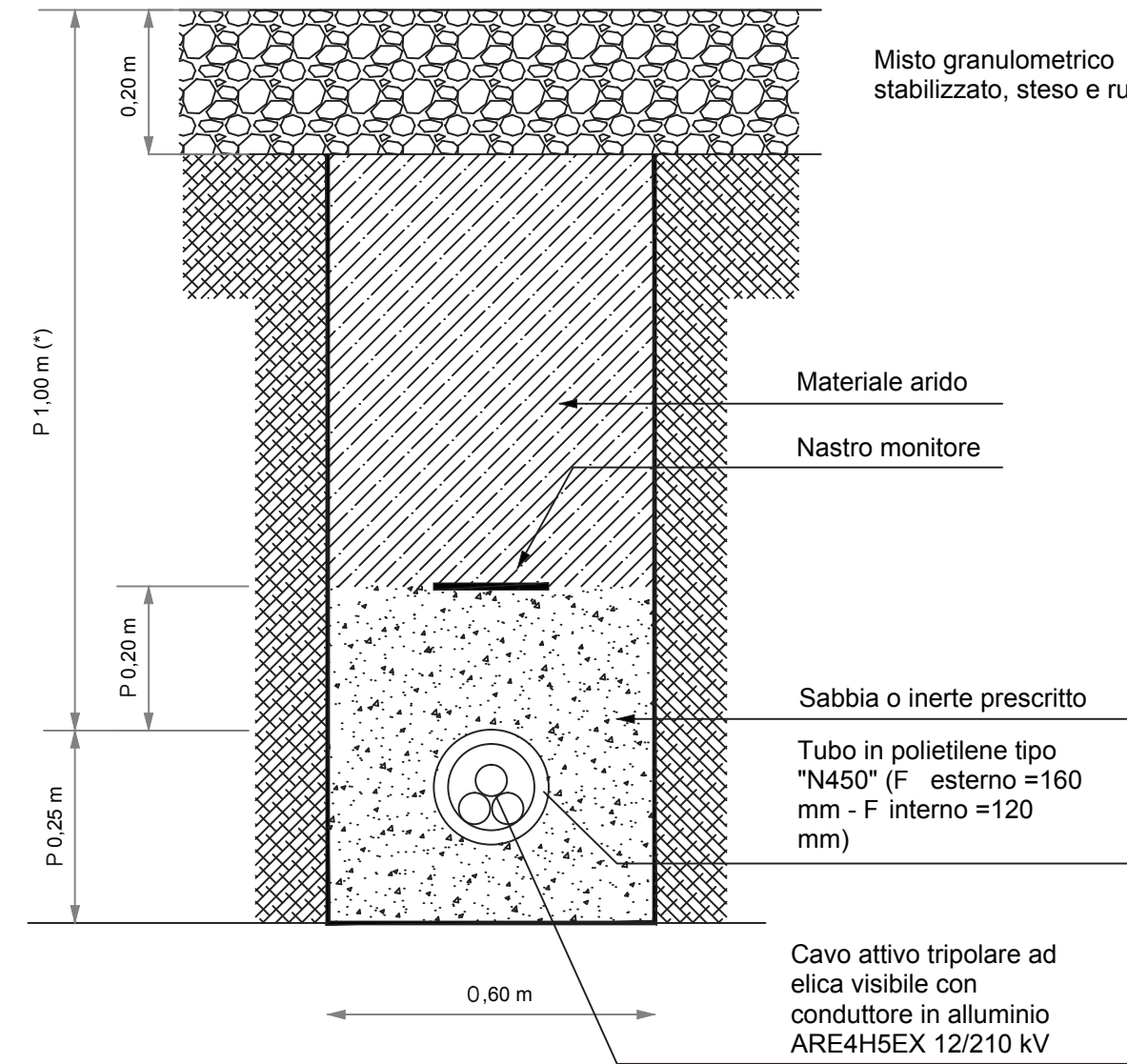
LINEA IN CAVO SOTTERRANEO IN TUBAZIONE POSA DI N.1 CAVI MT IN VIABILITÀ DI SERVIZIO SU MISTO STABILIZZATO
