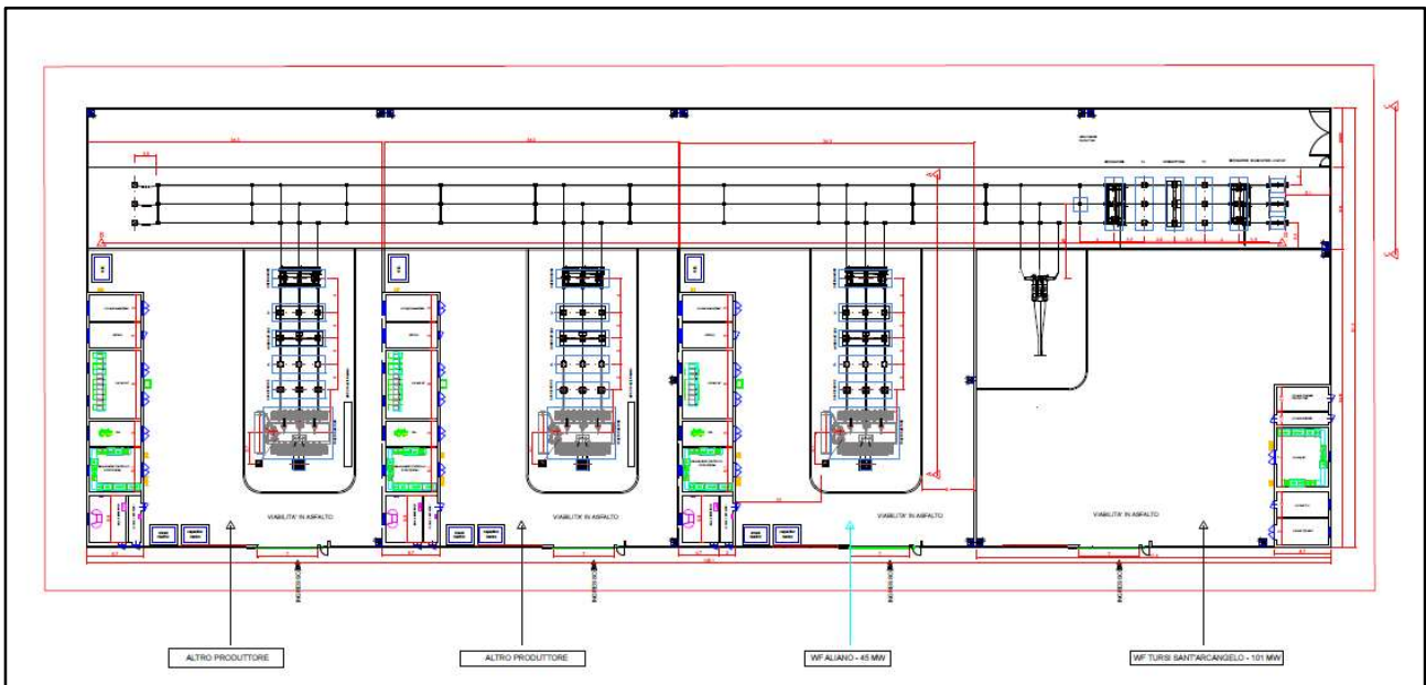
Figura 2.3.5.3: Planimetria elettromeccanica della Sottostazione elettrica condivisa
