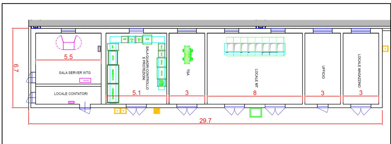
Figura 2.3.2.2: Pianta edificio di controllo SEU
