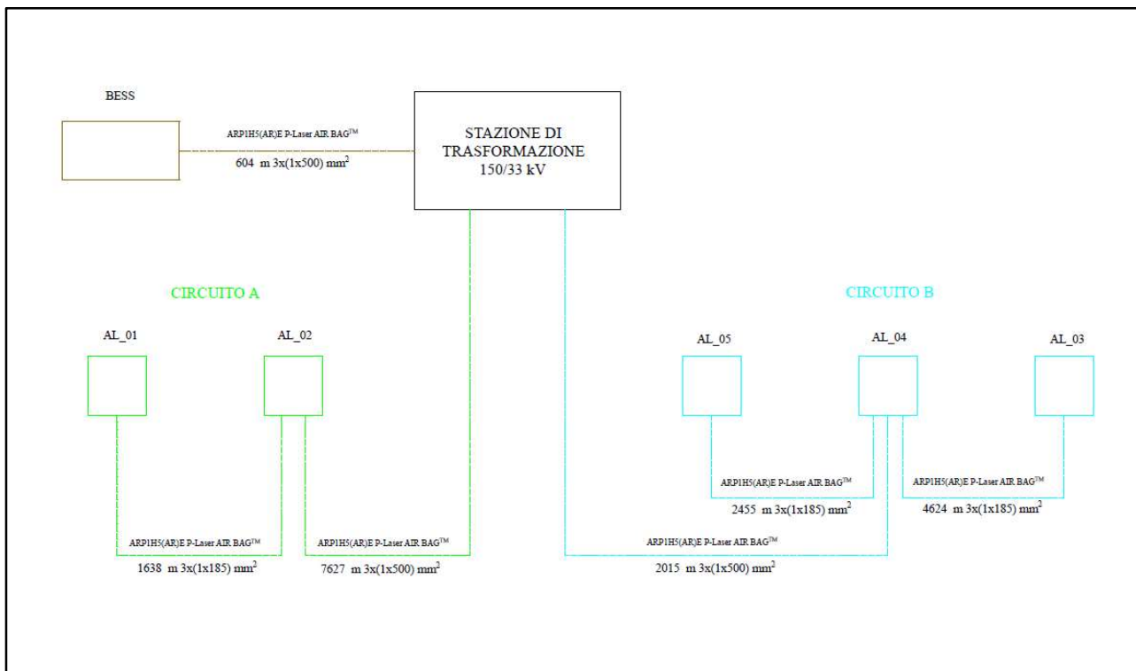
Figura 2.3.4.1: Schema a blocchi del Parco Eolico Aliano
