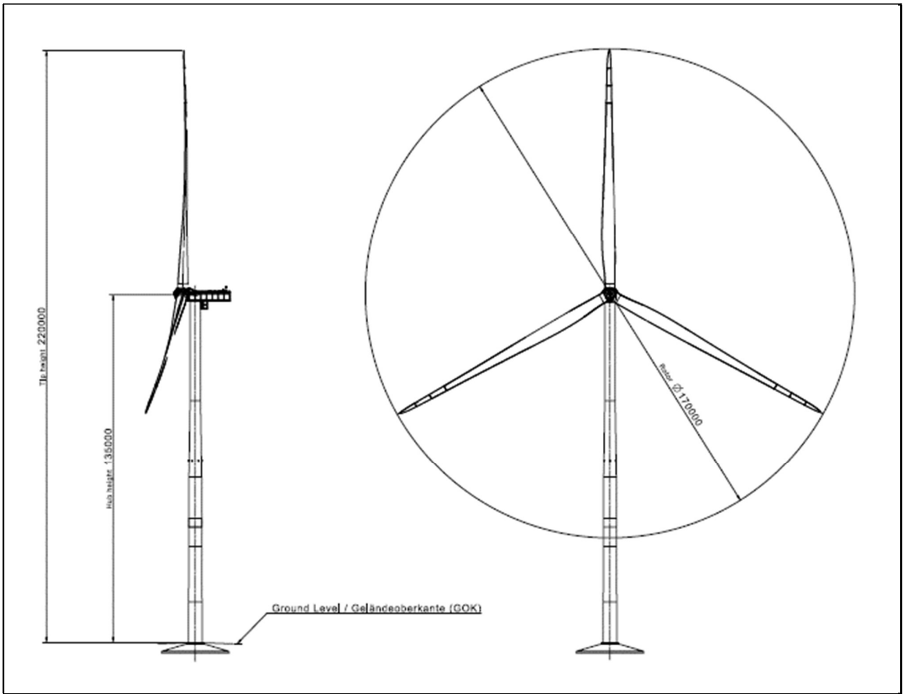
Figura 2.1.1: Profilo aerogeneratore SG170 HH135 – 6.2 MW
