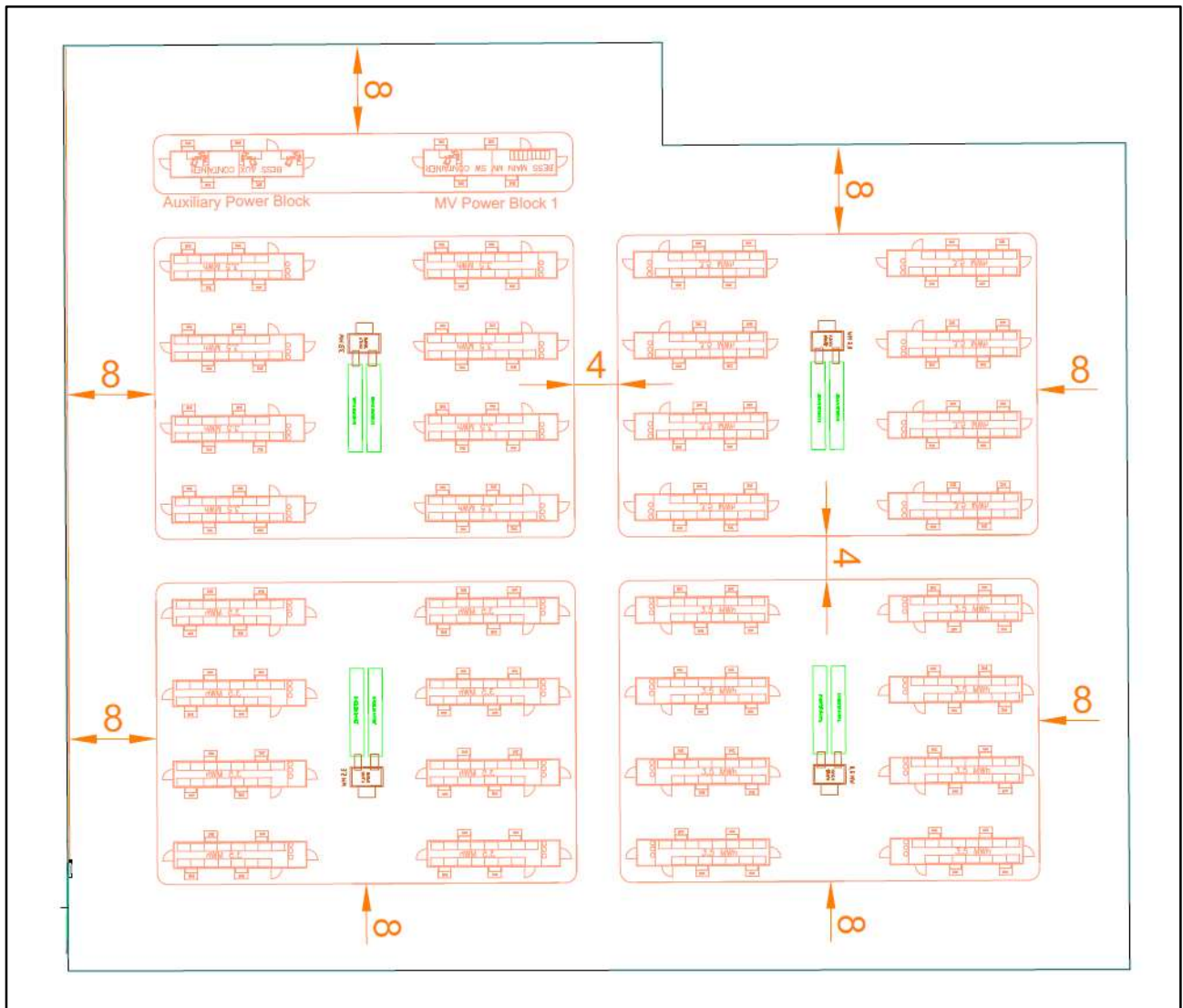
Figura 2.3.3.3: Esempio di configurazione BESS di potenza 14 MW
