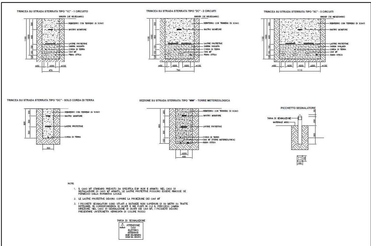
Figura 2.3.4.3: Sezioni tipiche delle trincee cavidotto su strada sterrata
