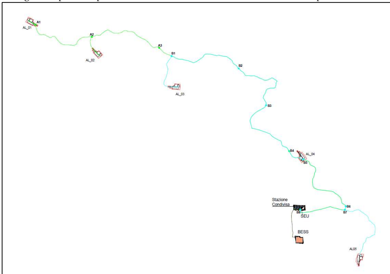
Figura 2.3.4.2: Planimetria di distribuzione linee MT dell'intero impianto
