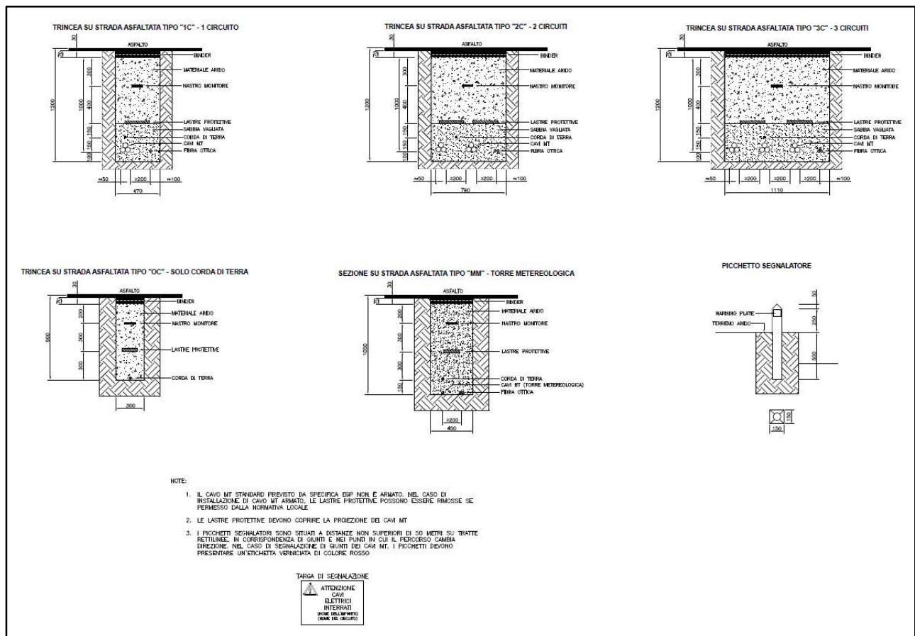
Figura 2.3.4.4: Sezioni tipiche delle trincee cavidotto su strada asfaltata
