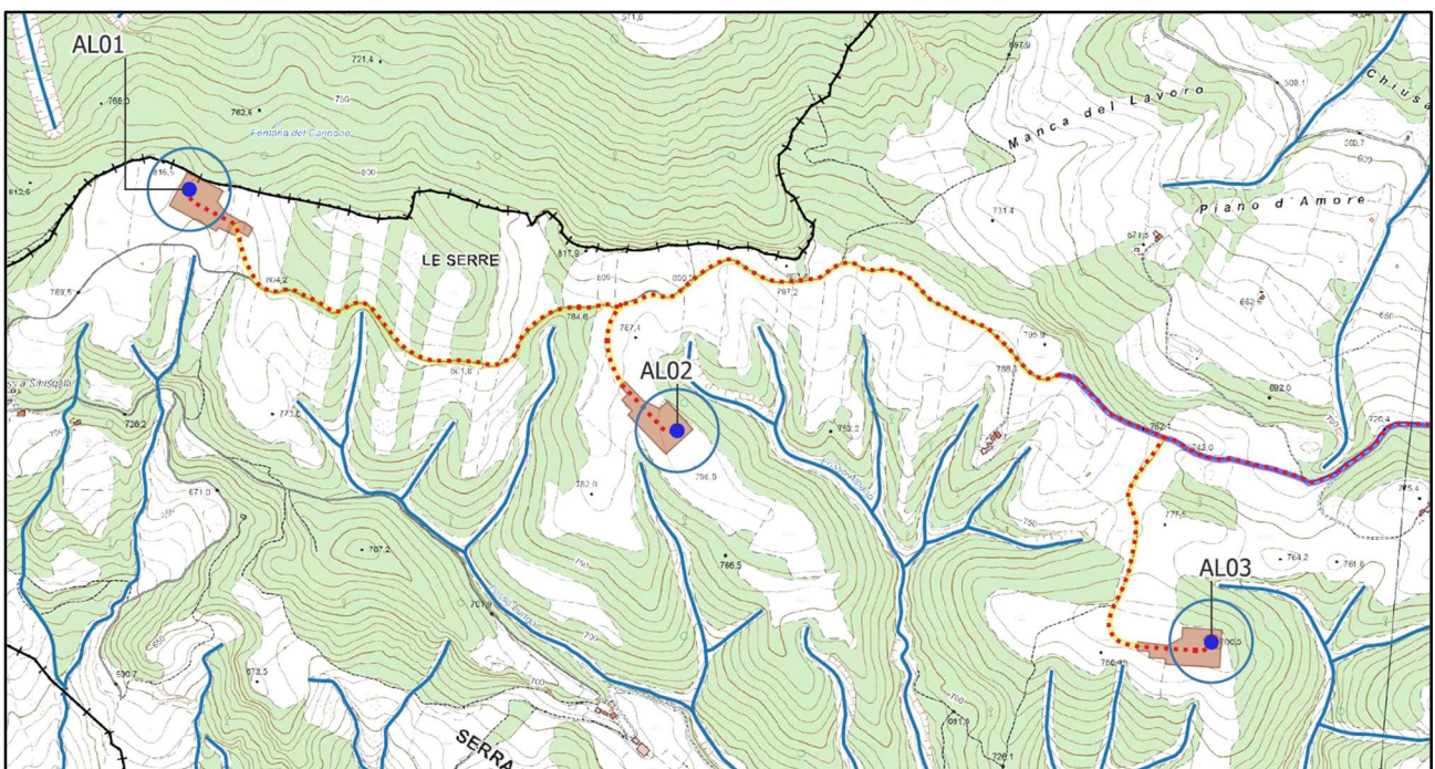
Figura 3.1: Interferenza del Parco Eolico con il reticolo idrografico dell'area (Fonte RSDI)
