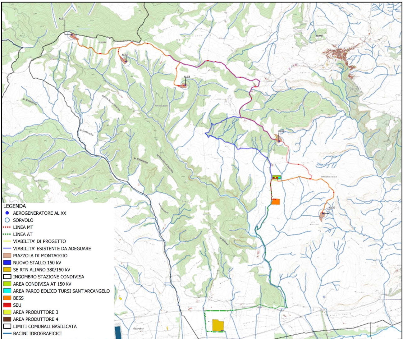
Figura 3.1: Interferenza del Parco Eolico con il reticolo idrografico dell'area (Fonte RSDI)
