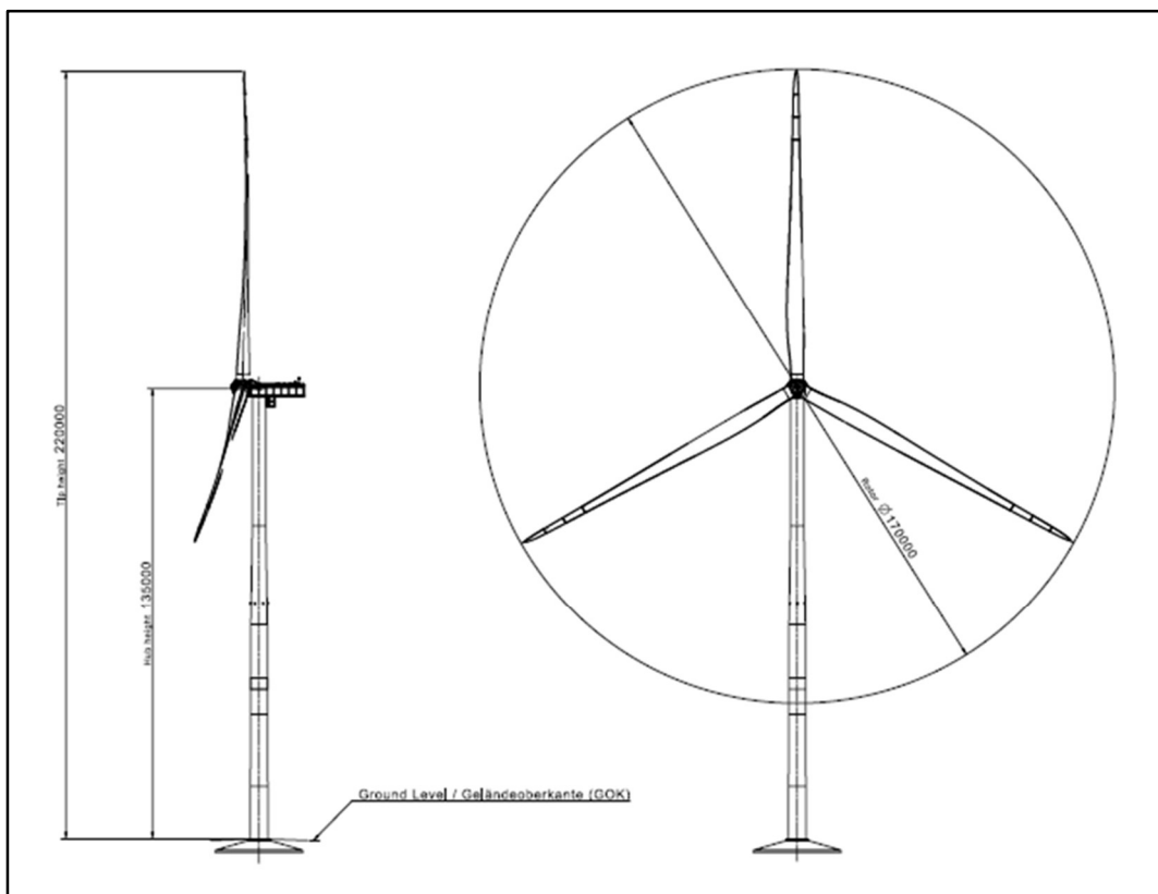
Figura 2.1.1: Profilo aerogeneratore SG170 HH135 – 6.2 MW
