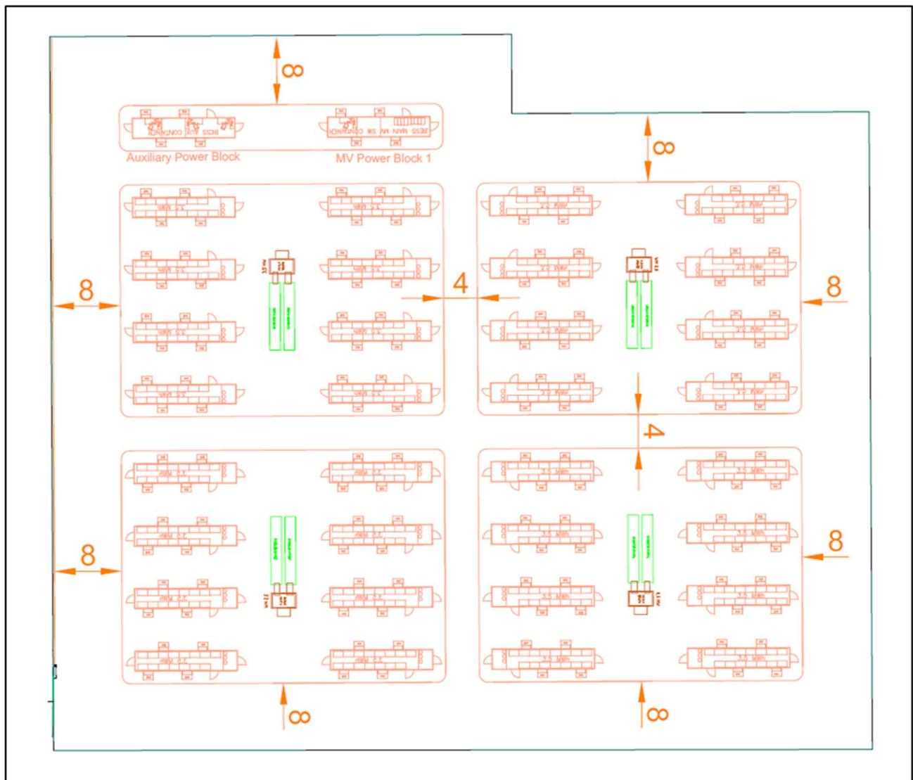
Figura 2.3.2: Esempio di configurazione BESS di potenza 14 MW
