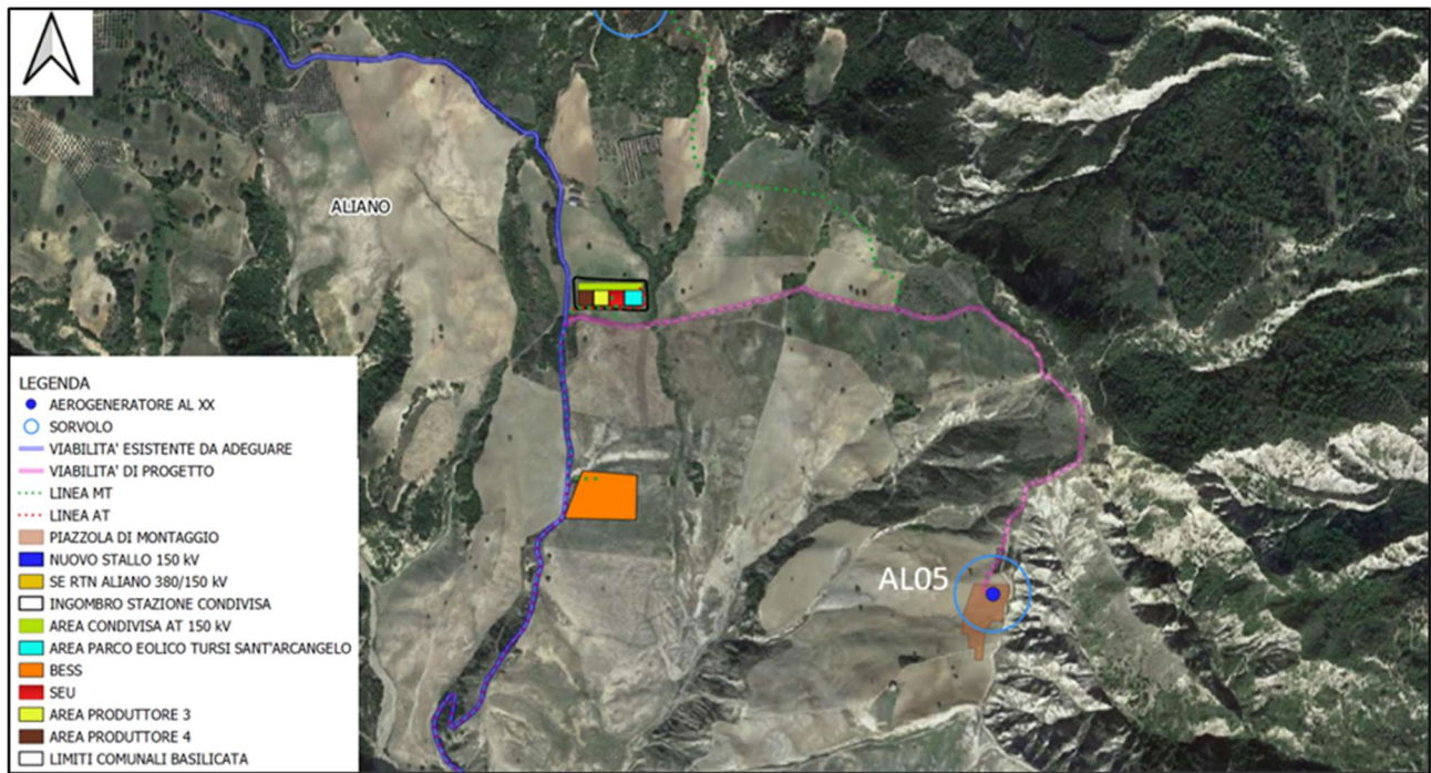
Figura 2.3.1: Localizzazione SEU 150/33 kV e BESS su ortofoto
