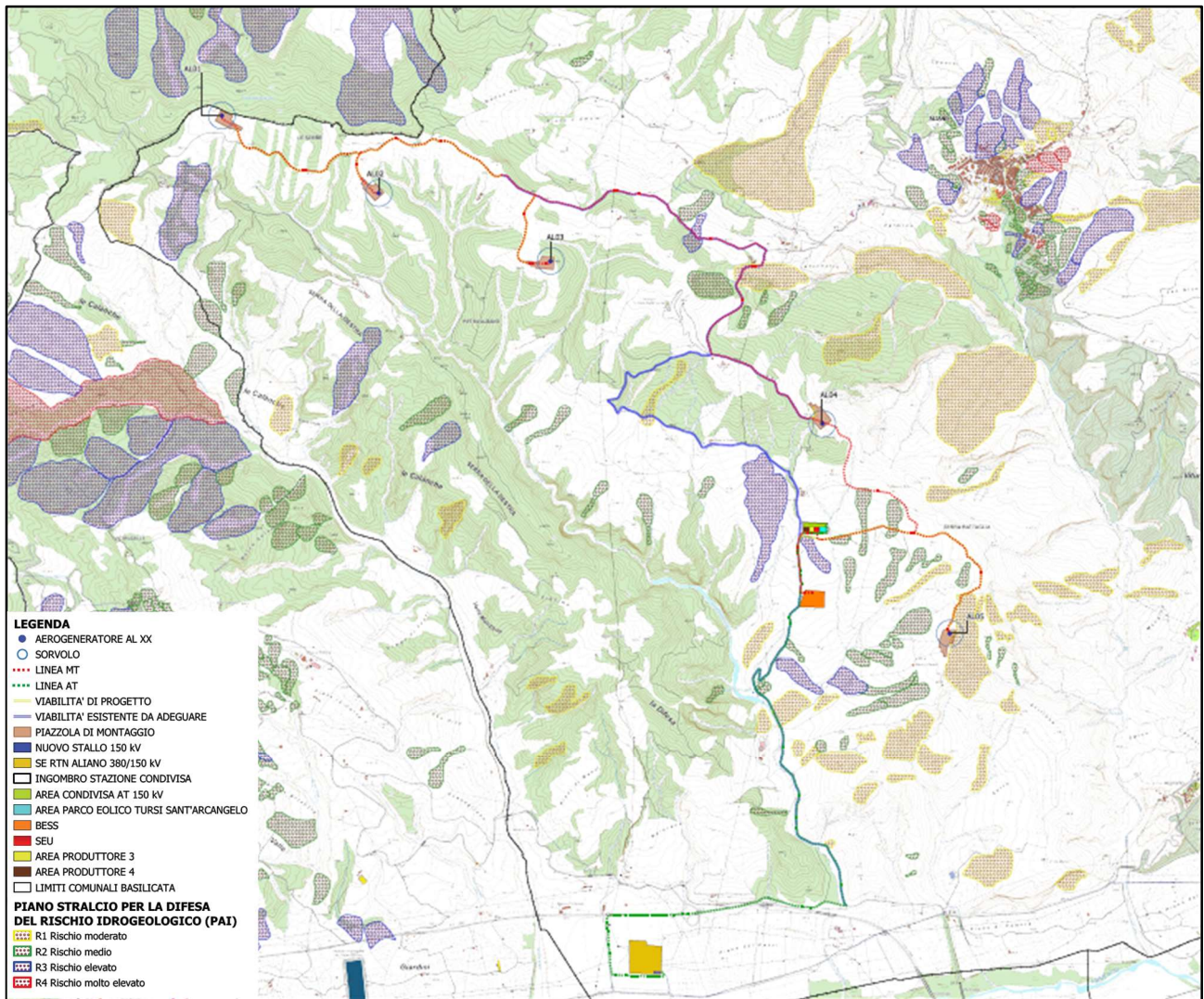
Figura 4.1: Interferenza del Parco Eolico con il Piano di Assetto Idrogeologico Regione Basilicata (Fonte RSDI)
