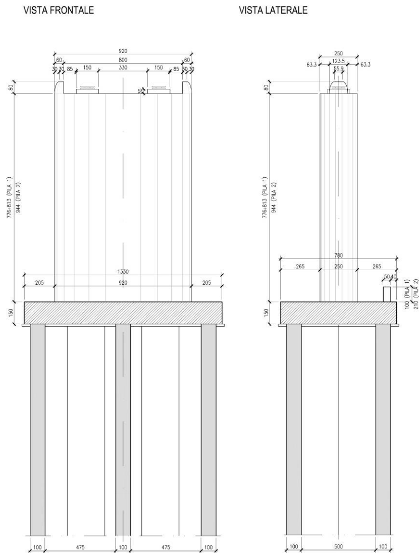
FIGURA 3-6: CARPENTERIA PILE.
