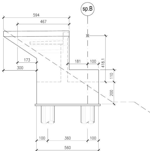
FIGURA 3-8: CARPENTERIA SPALLE.
