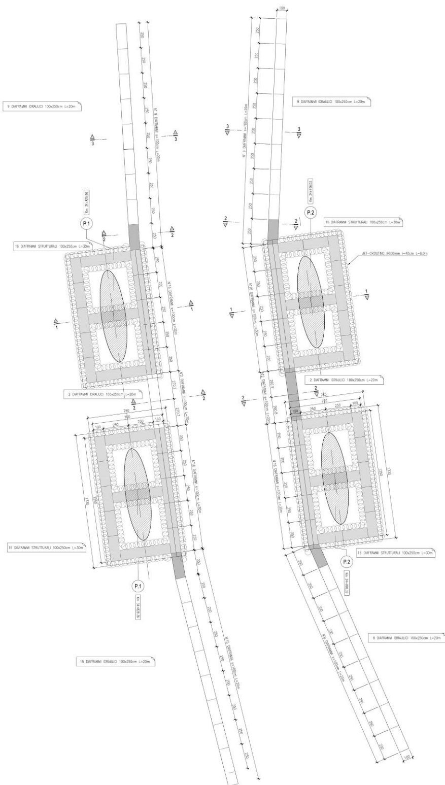
FIGURA 3-7: PIANTA PILE E DISPOSIZIONE DEI DIAFRAMMI STRUTTURALI ED IDRAULICI.
