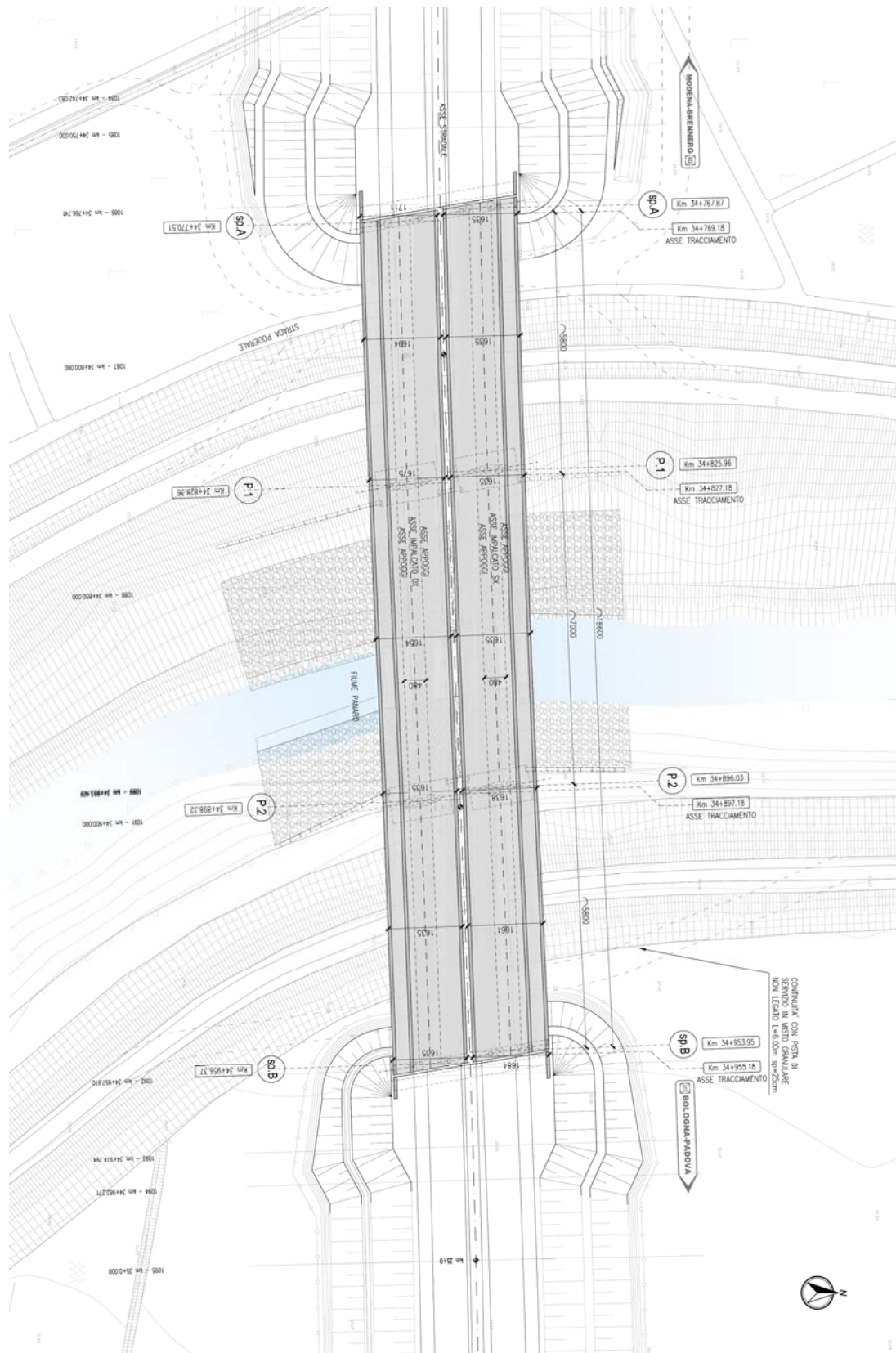
FIGURA 3-1: PLANIMETRIA.
