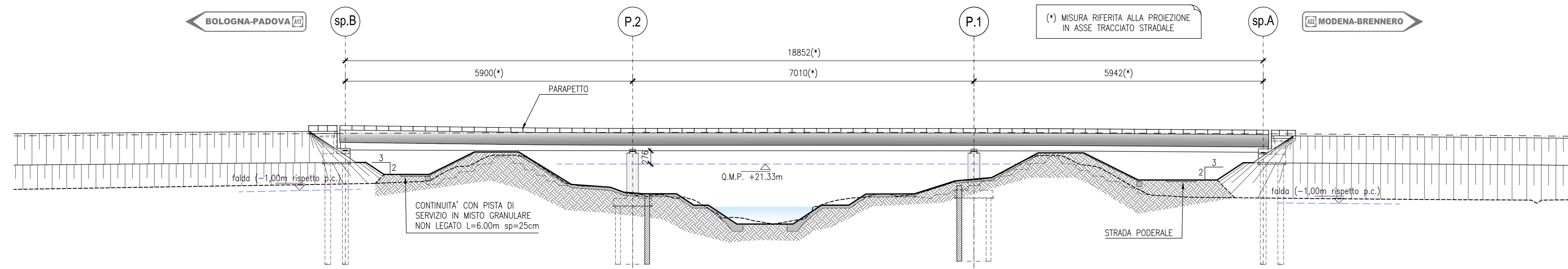
PROSPETTO LATO SX SCALA 1:500
