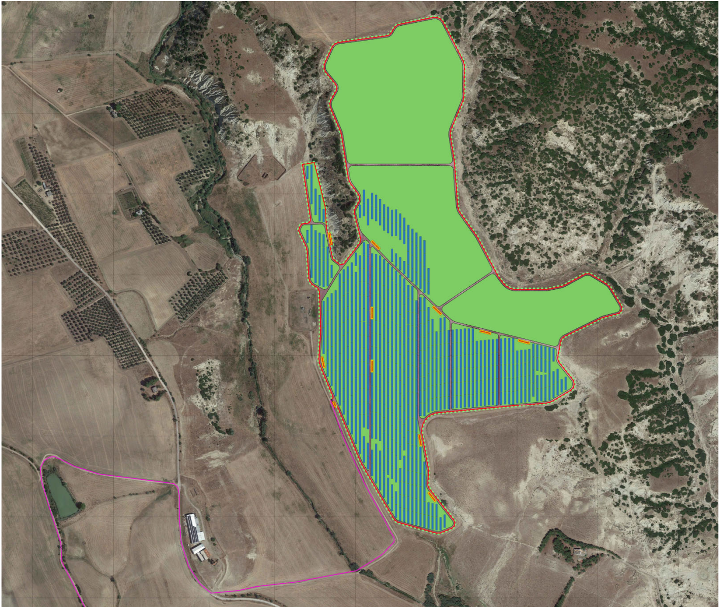
Figura 2 –Layout dell’impianto fotovoltaico su ortofoto
