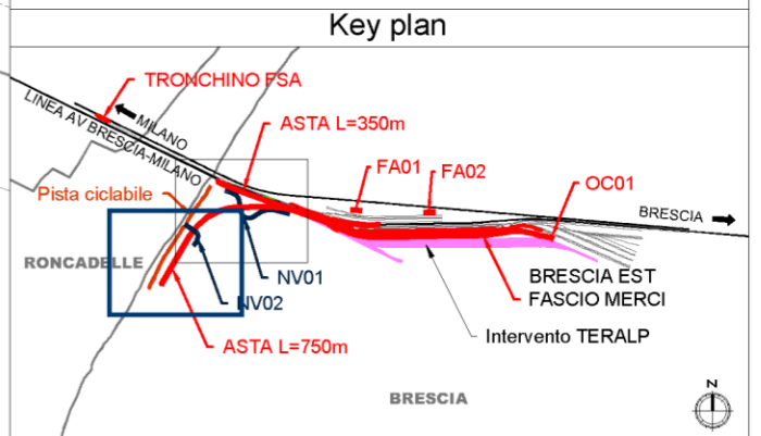
Planimetria opere a verde 2/2
