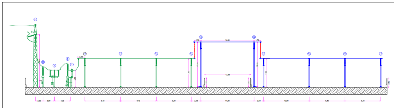
Figura 13 – Prolungamento della Stallo linea in condivisione con altri produttori.
