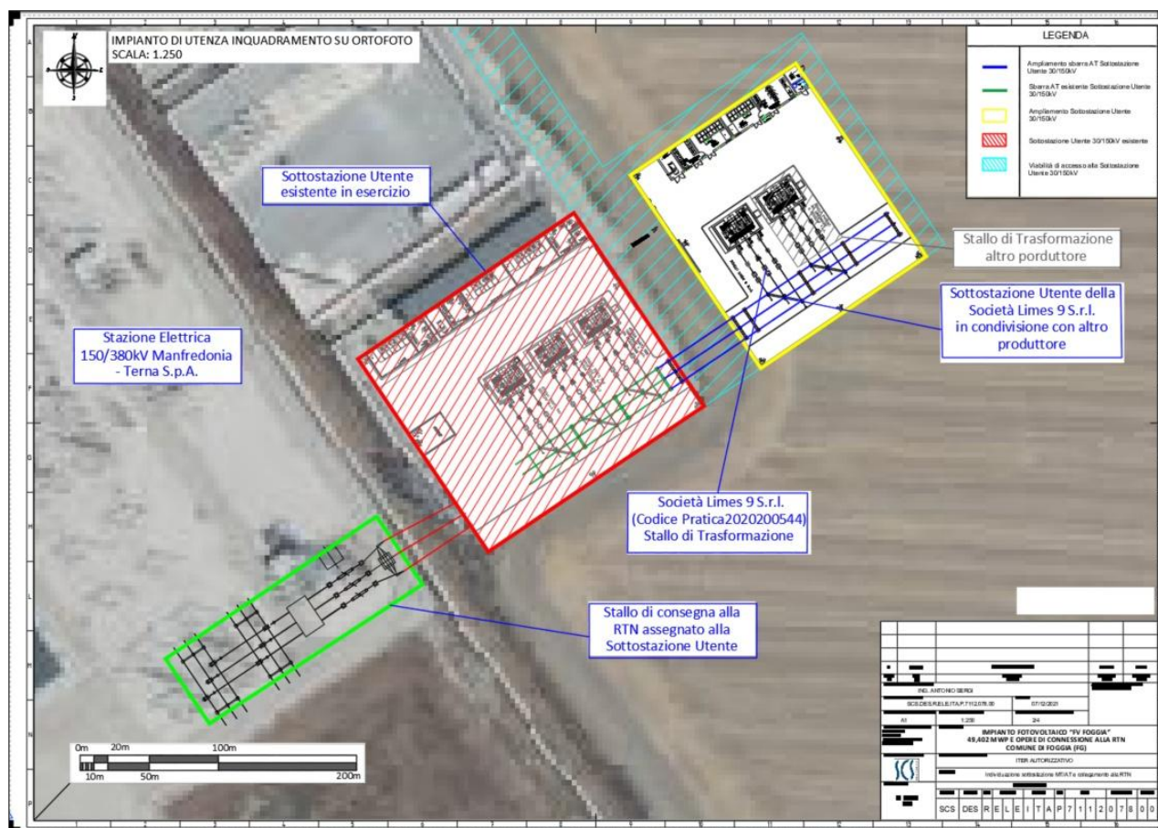
Figura 18 – Individuazione su ortofoto Stallo AT nella SE Terna
