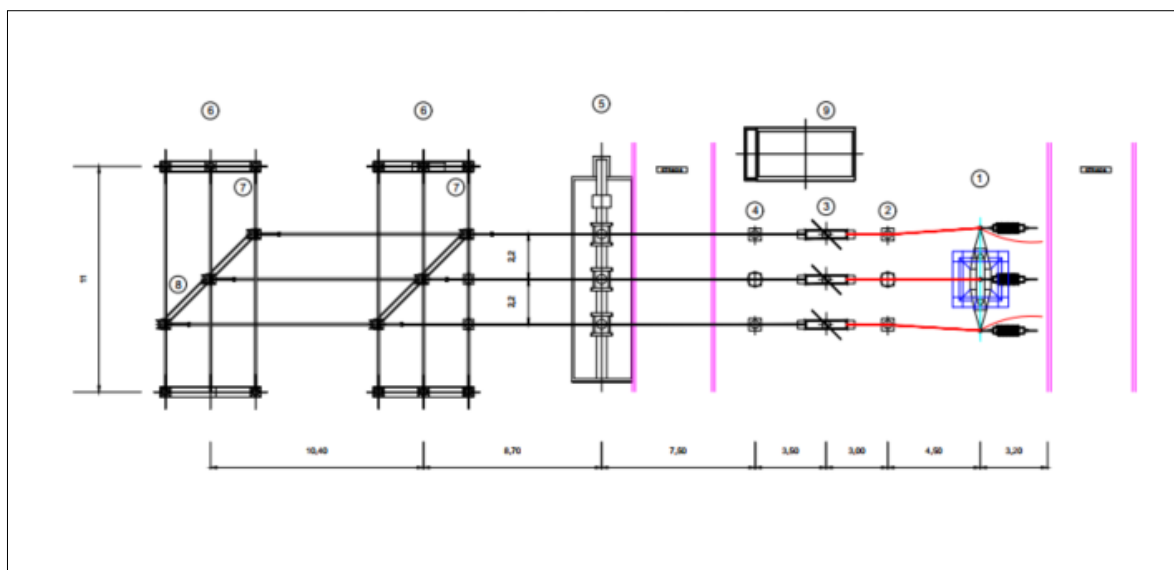
Figura 19 - Planimetria apparecchiature stallo 150 KV nella SE Terna
