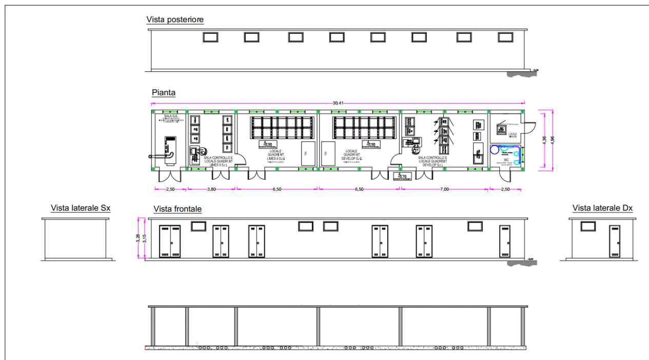
Figura 16 - Edificio interno alla SSU.
