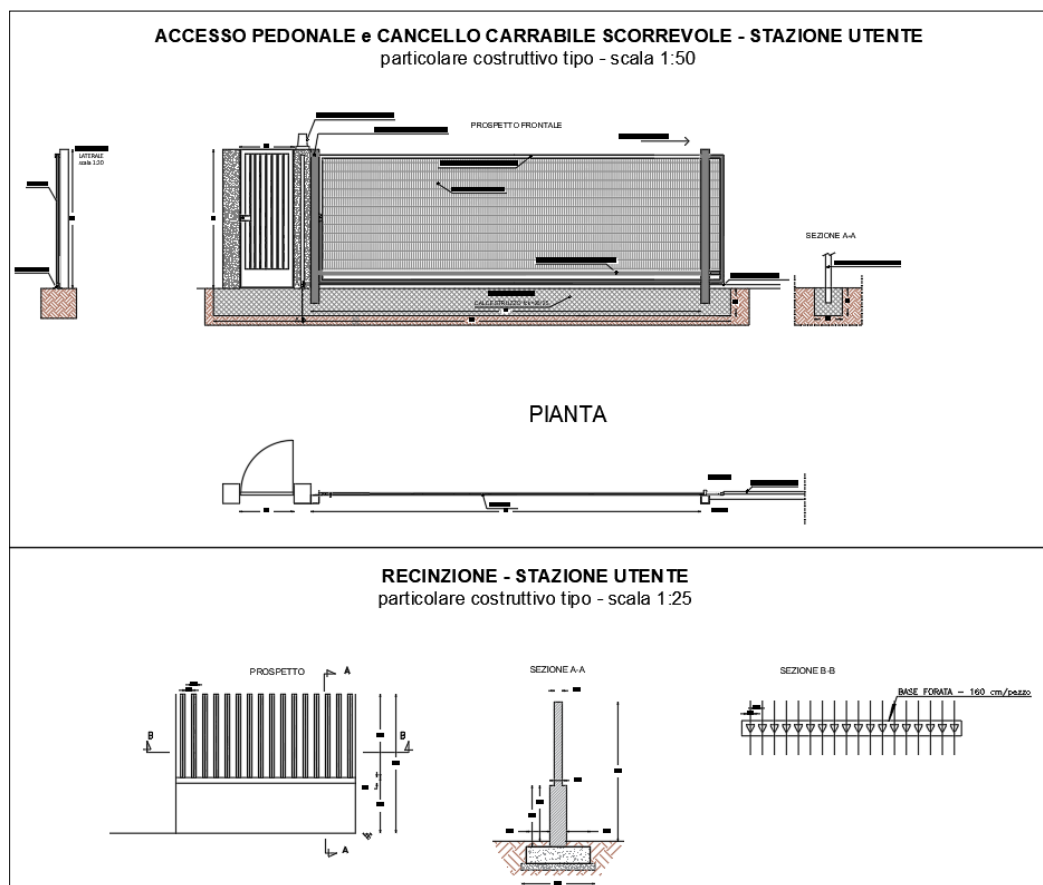
Figura 17: Recinzione e cancello.
