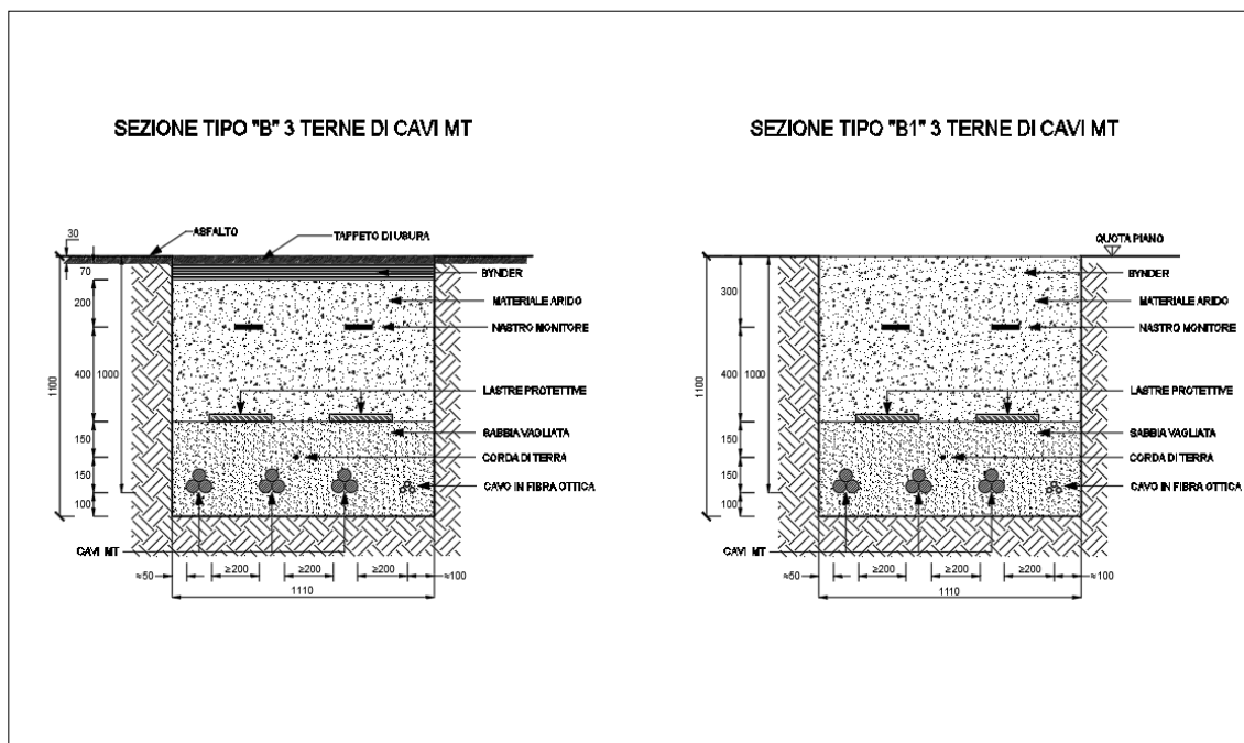
Figura 2: Tipo sezione su strada asfaltata e sterrata
