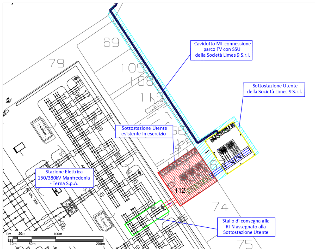
Figura 6 - Stralcio 4 da planimetria catastale - percorso cavidotto MT
