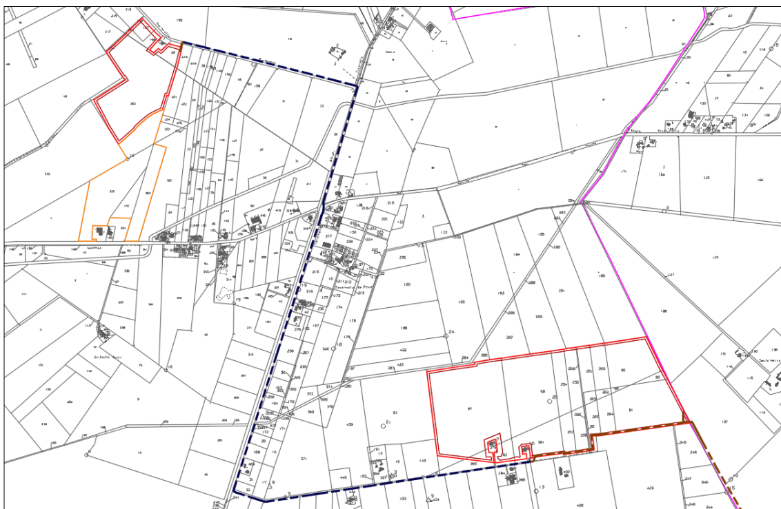
Figura 3: Stralcio 1 da planimetria catastale - percorso cavidotto MT
