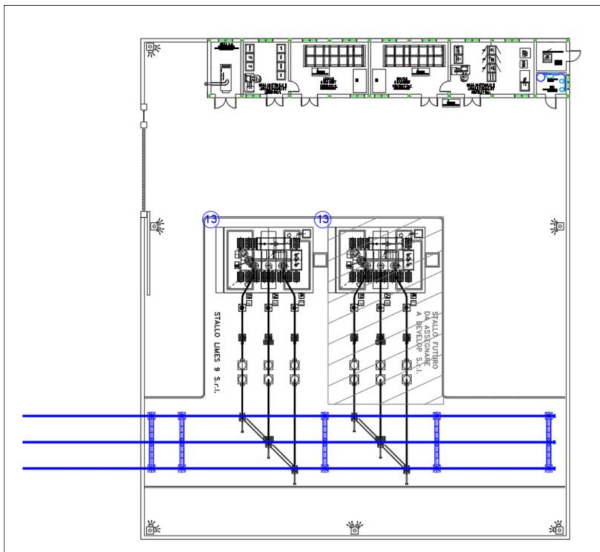
Figura 11 - Pianta Sottostazione MT/AT Limes 9 S.r.l.
