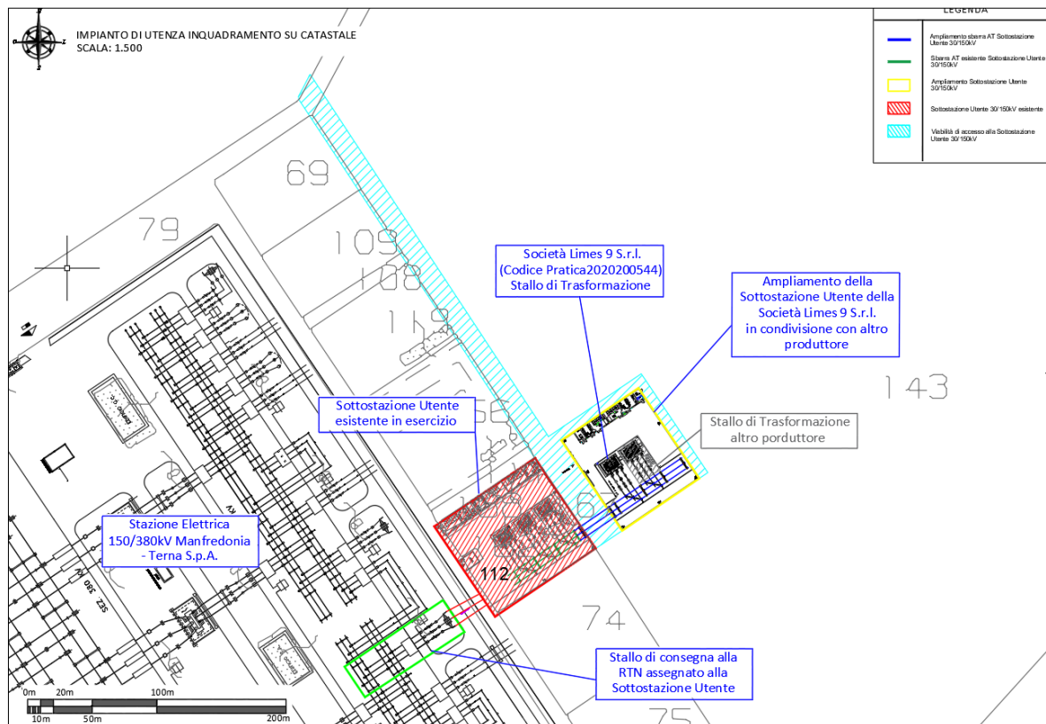
Figura 9 Stralcio della SSU d'impianto su Mappa catastale(riquadro giallo).
