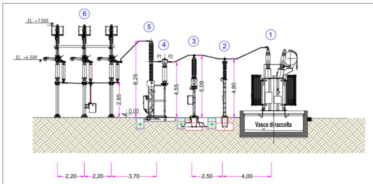
Figura 12 - Stallo di trasformazione LIMES 9 S.r.l.
