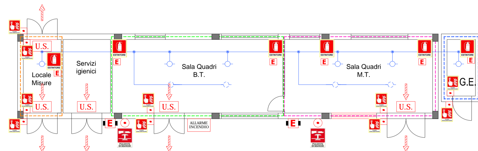
PIANTA EDIFICIO UTENTE SISTEMA DI ACCUMULO - SCALA 1:100
