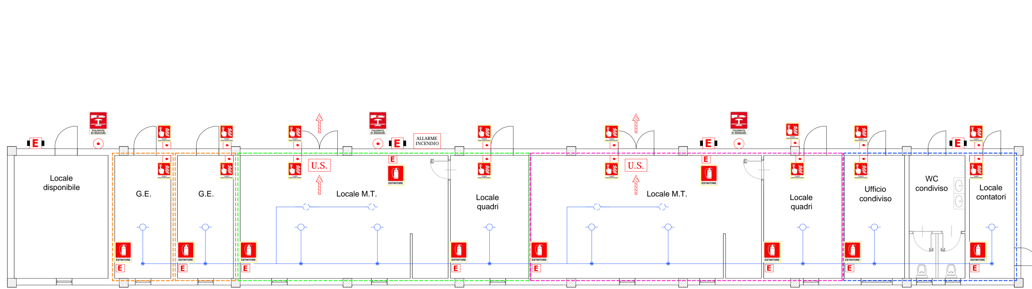
PIANTA EDIFICIO UTENTI IN SSEU - SCALA 1:100
