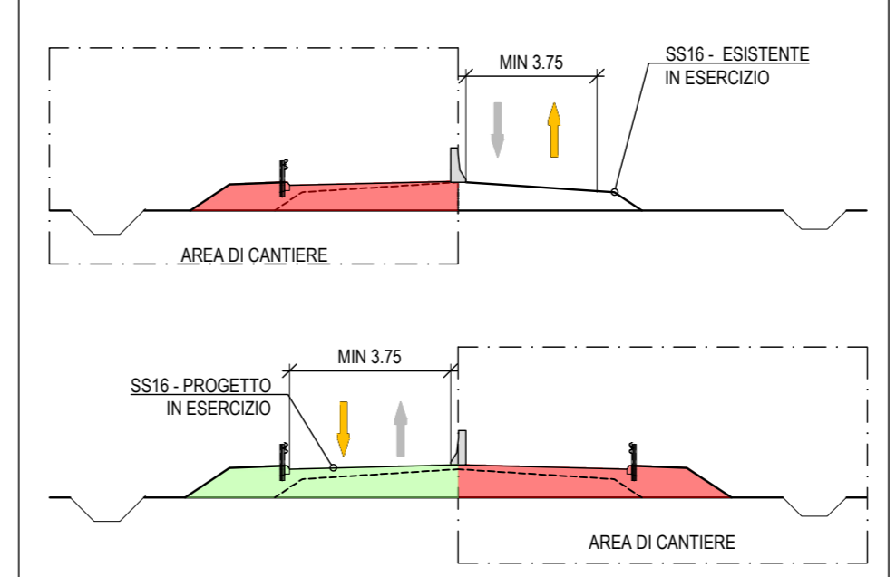
SCHEMA FASI REALIZZATIVE - FASE 5 (DA PK 21+660.00 A PK 22+280.00)
