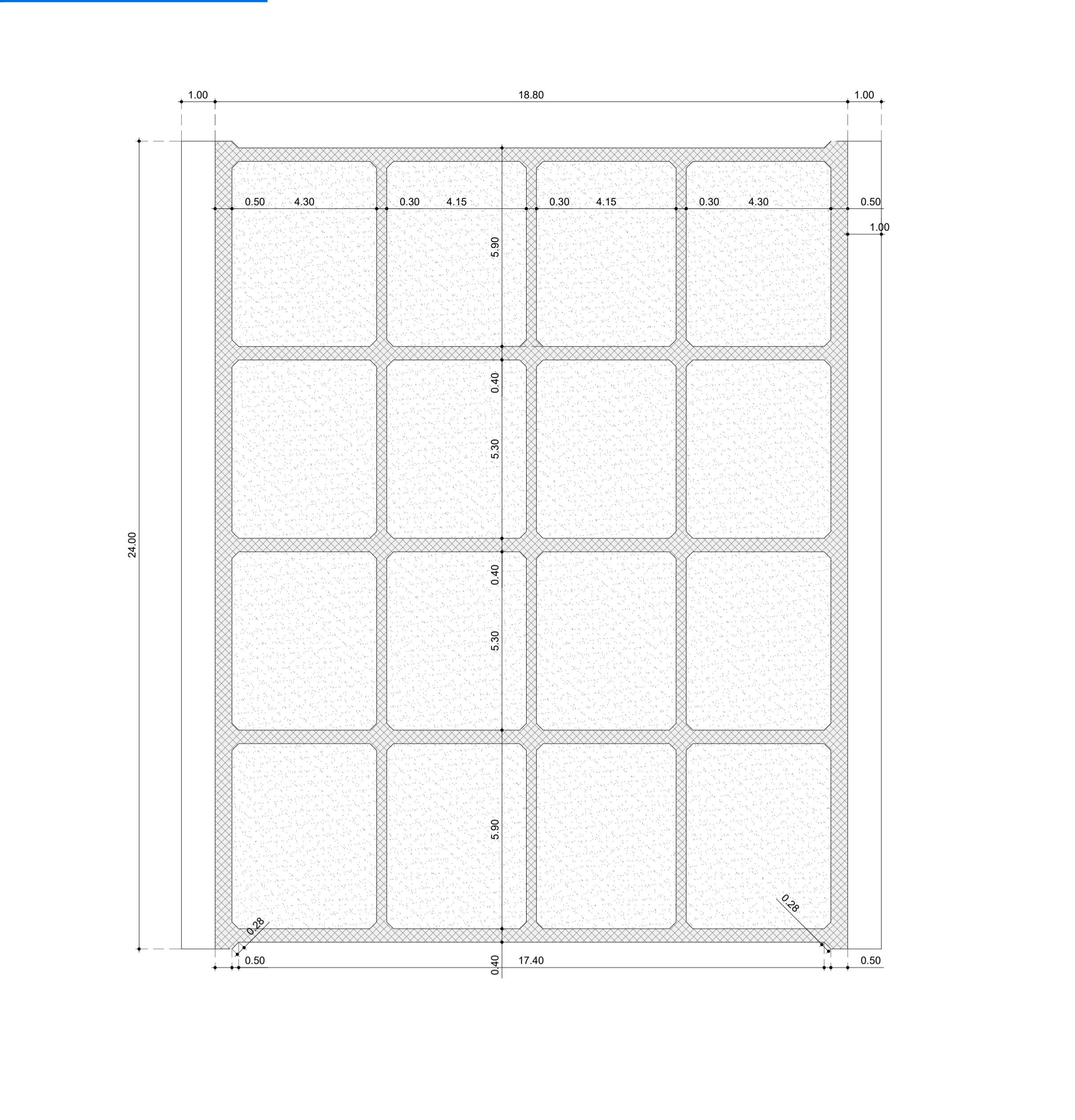
PIANTA CASSONE CELLULARE - (scala 1:100)
