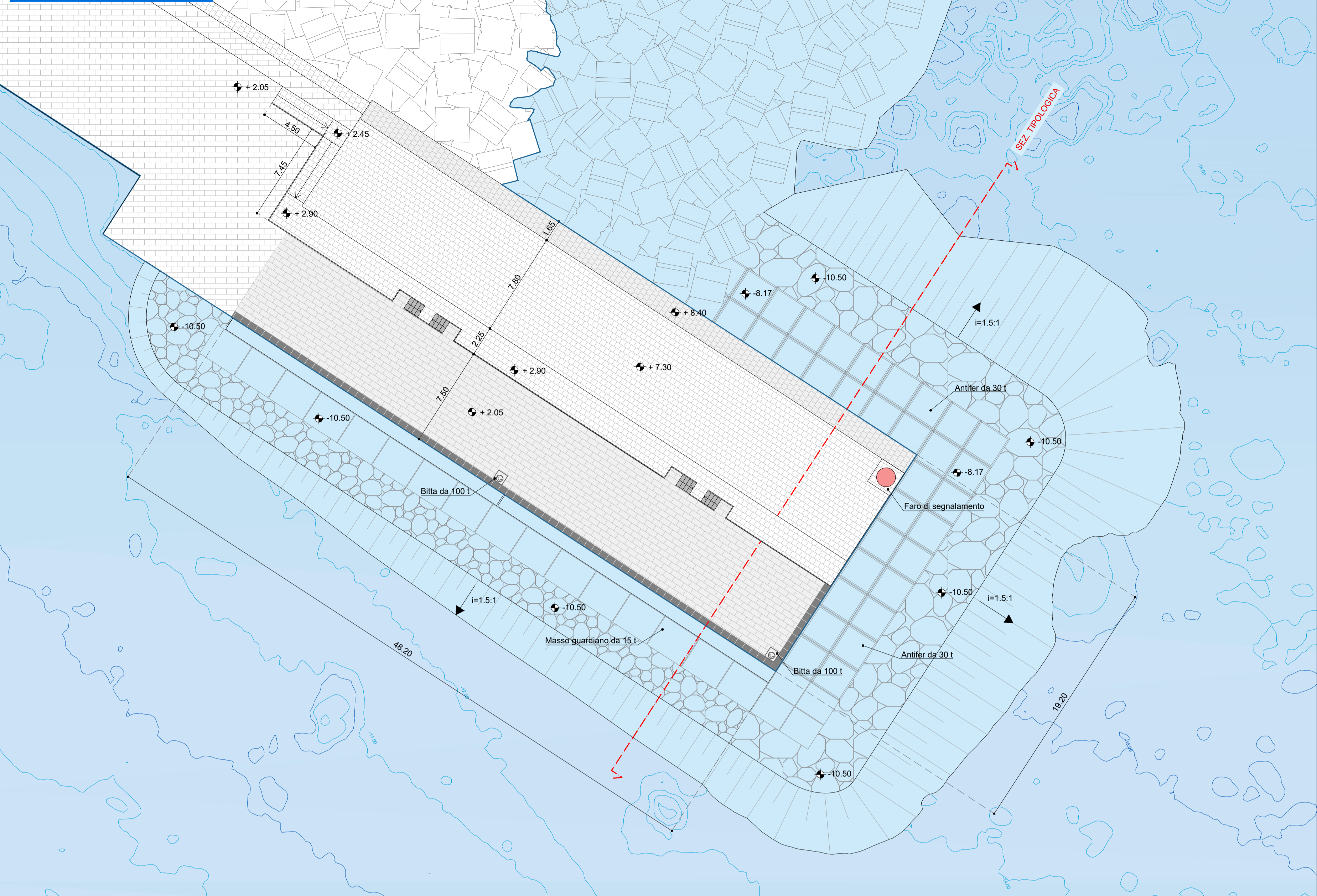
PLANIMETRIA DI DETTAGLIO - (scala 1:200)
