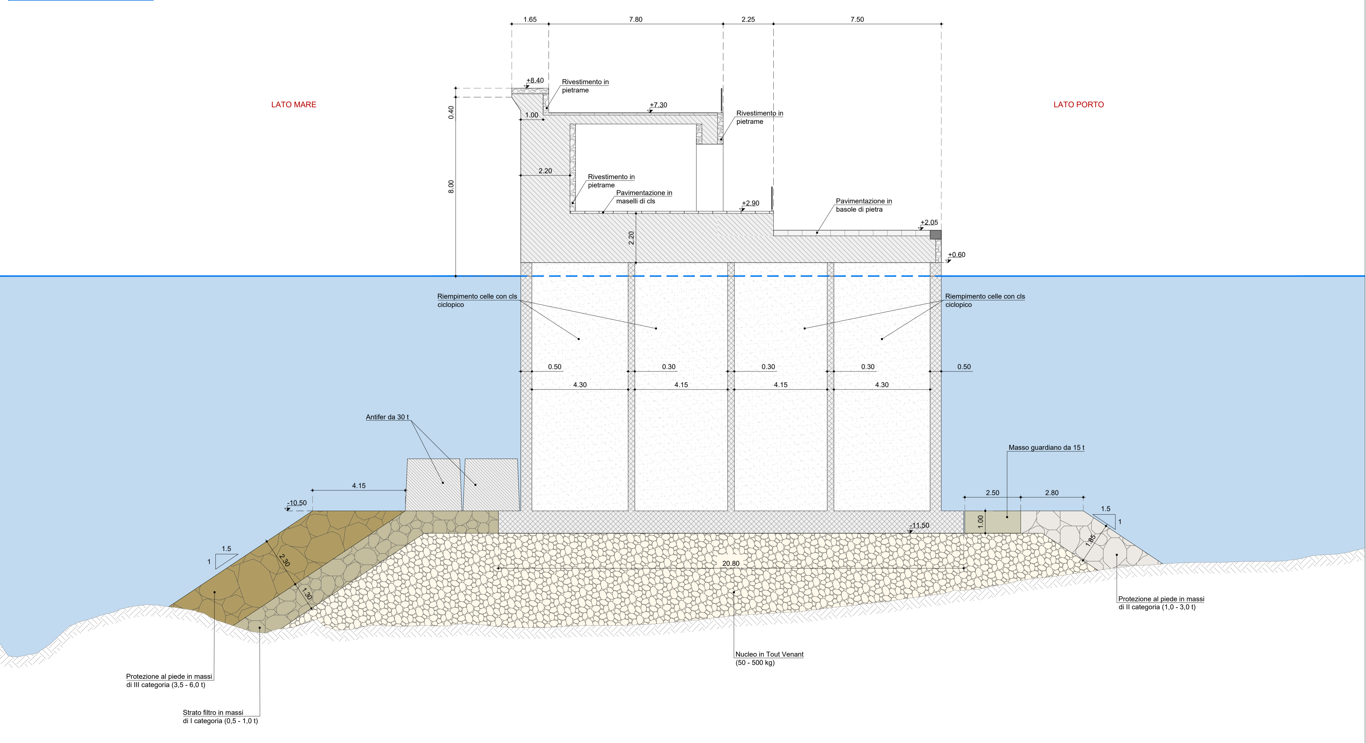
SEZIONE TIPOLOGICA - (scala 1:100)
