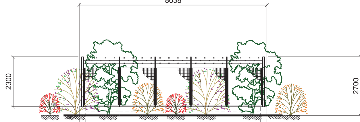
PROSPETTO B
