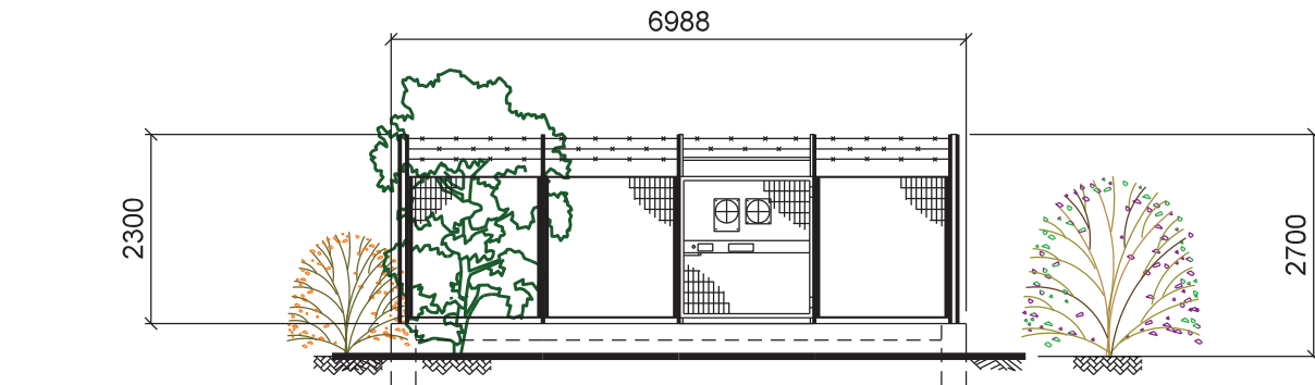
PROSPETTO A
