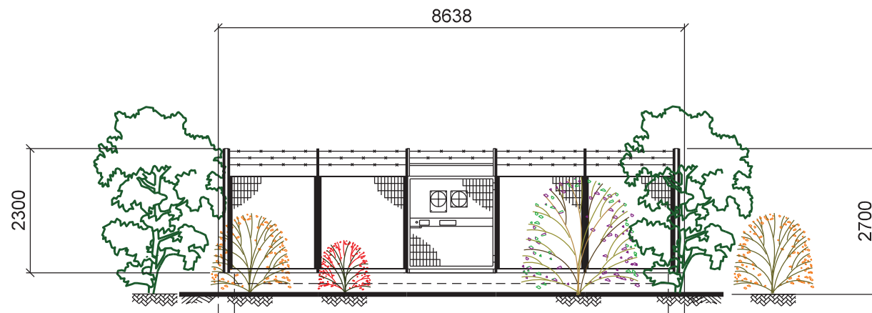
PROSPETTO A
