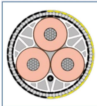
Figura 6.1: Esempio di cavo di collegamento a 66 kV / 220 kV e tipico di sezione
