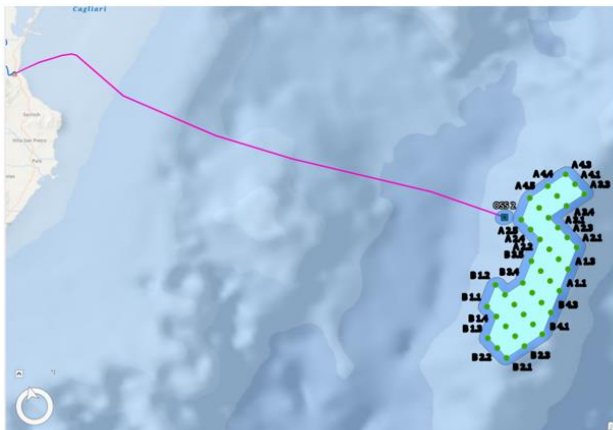
Figura 3.1: Vista del tracciato preliminare del cavidotto marino
