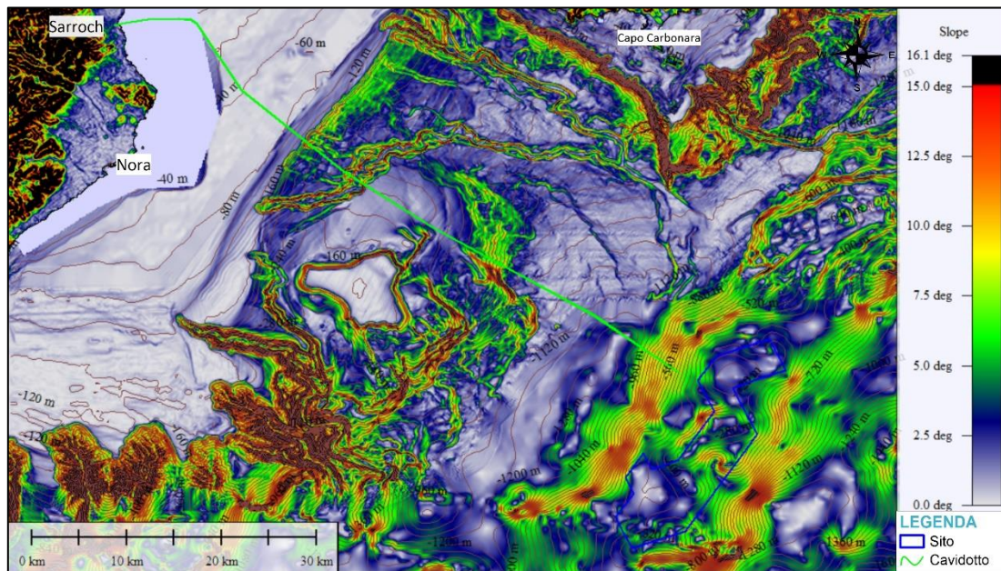
Figura 3.9: Carta delle pendenze dell’area marina di interesse (dati: EMODNet)
