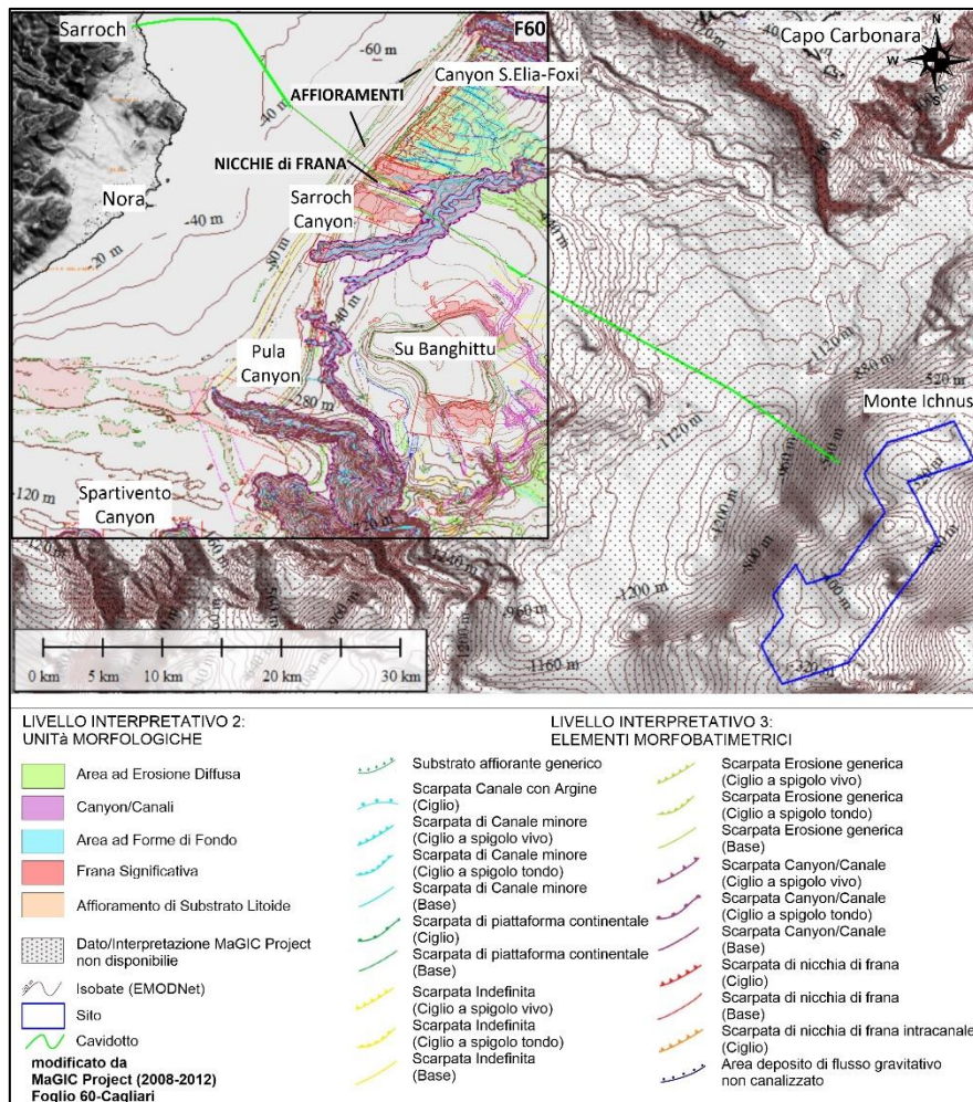
Figura 3.11: Elementi morfobatimetrici presenti nel sito (Ref.[30]). Il rettangolo nero indica il Foglio del Progetto Magic F60 (Cagliari)
