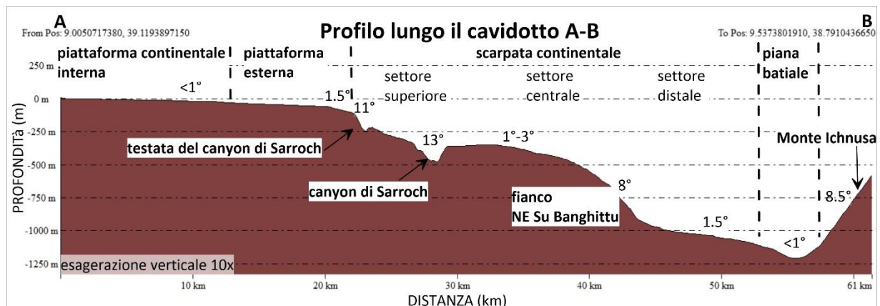
Figura 3.10: Profilo lungo il cavidotto A-B
