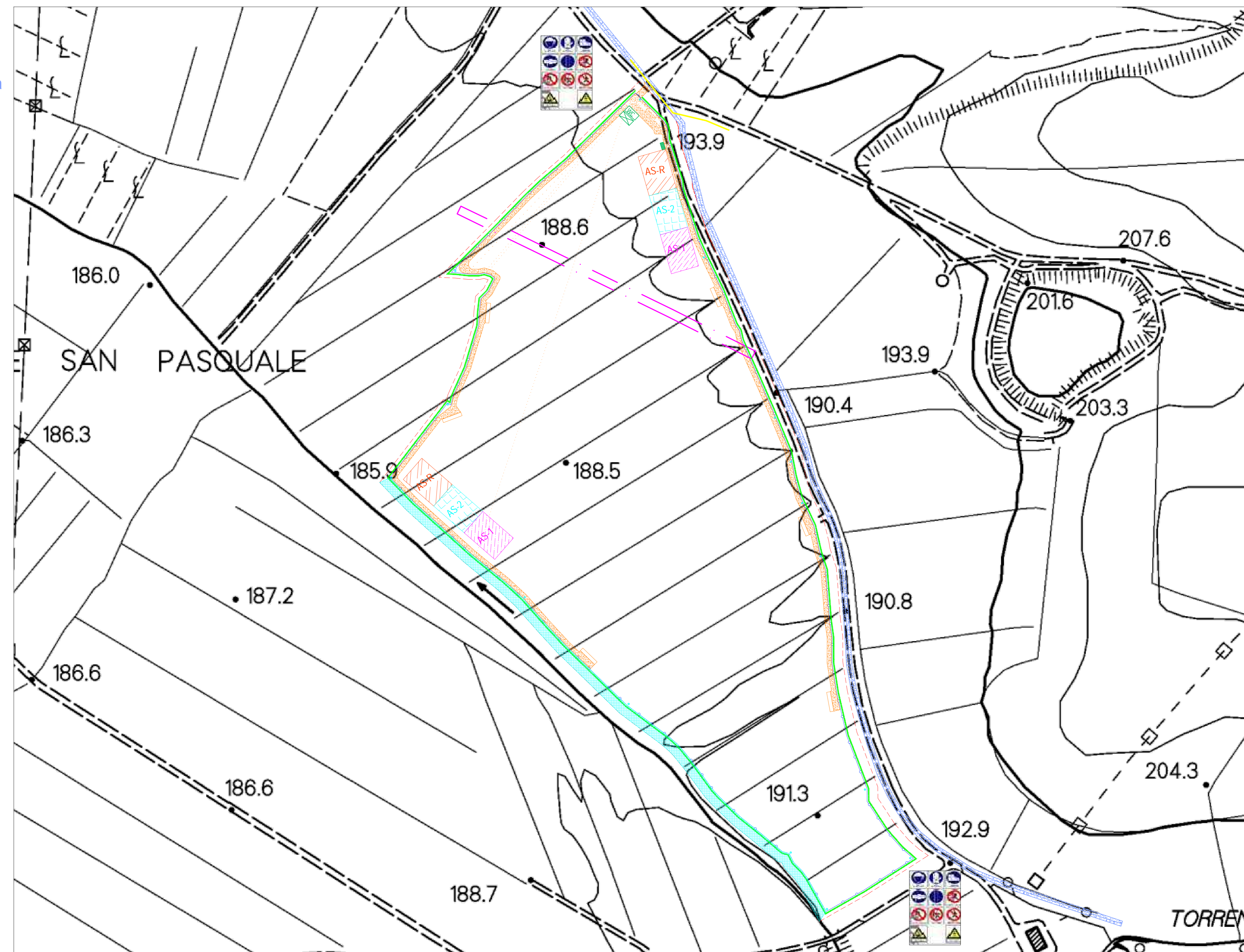
INQUADRAMENTO CANTIERE IMPIANTO FOTOVOLTAICO SU STRALCIO CTR - scala 1:2.000
