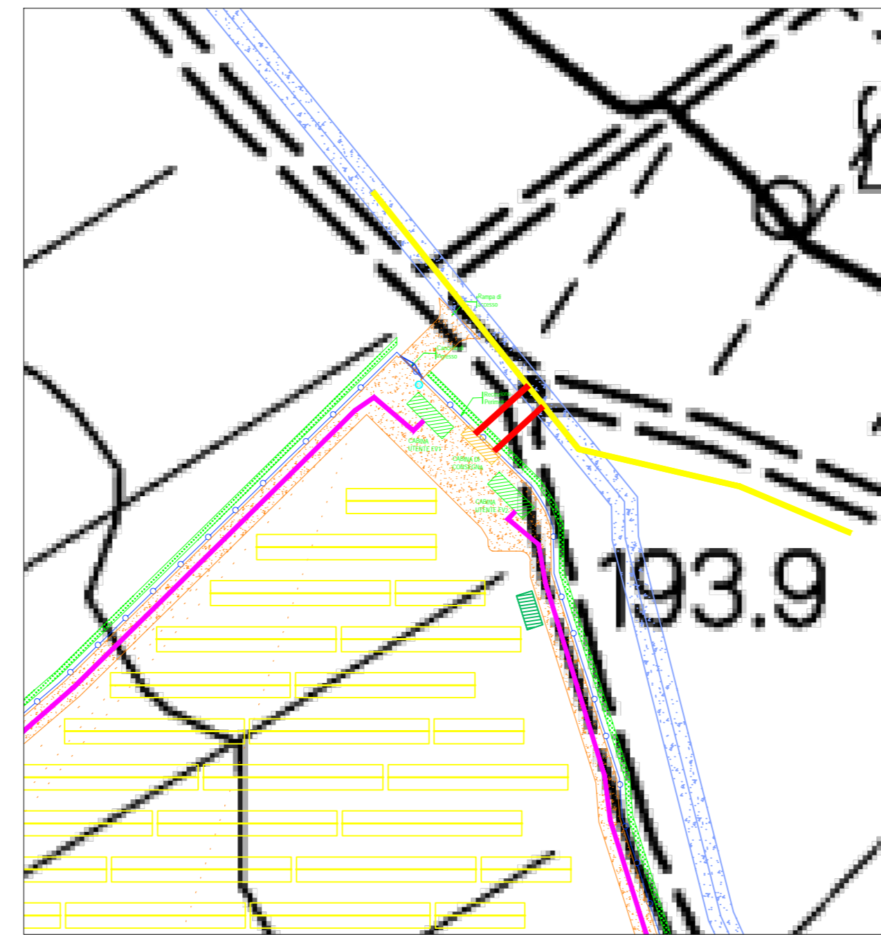
PARTICOLARE INGRESSO IMPIANTO FV - scala 1:1.000
