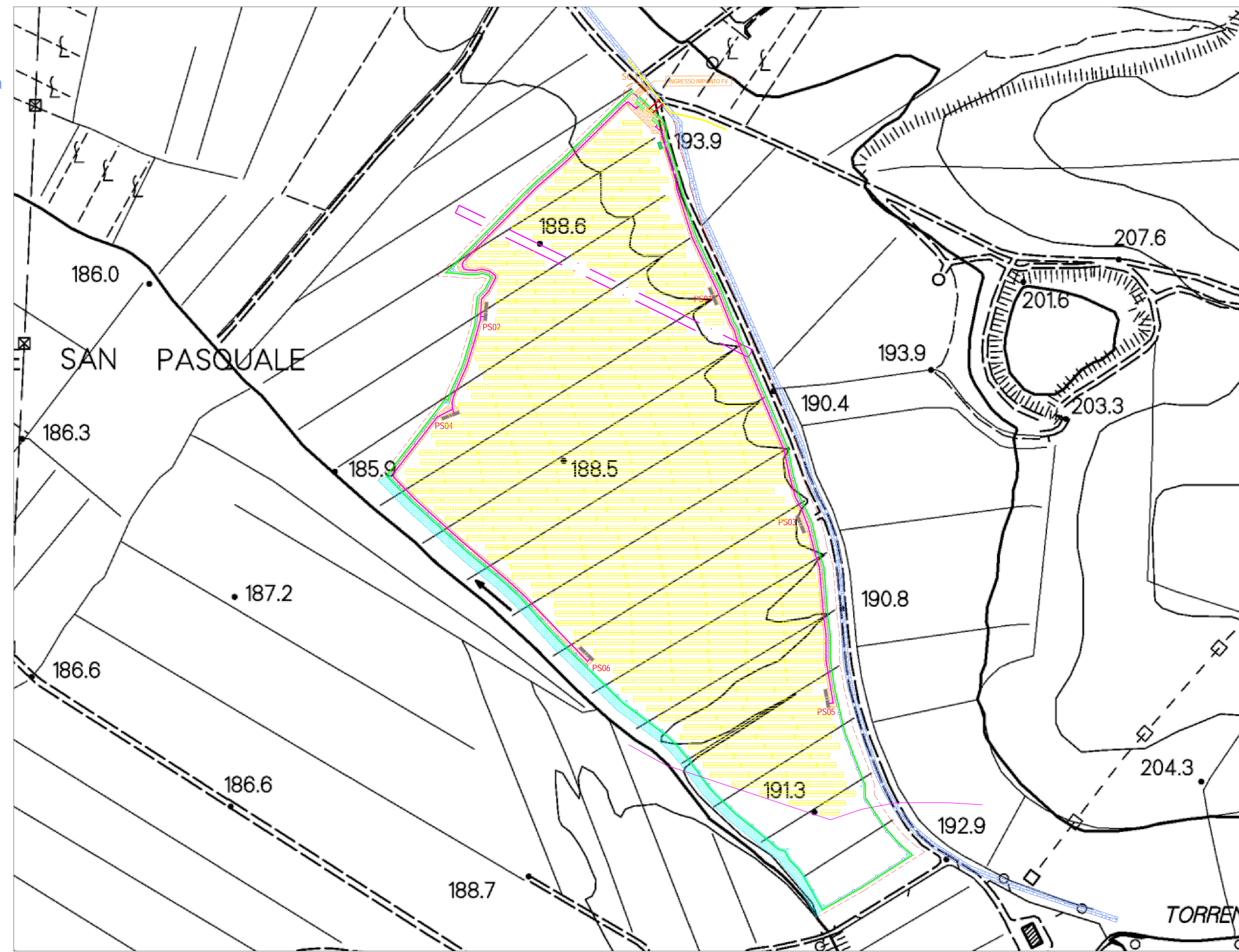
INQUADRAMENTO IMPIANTO FOTOVOLTAICO SU STRALCIO CTR - scala 1:2.000
