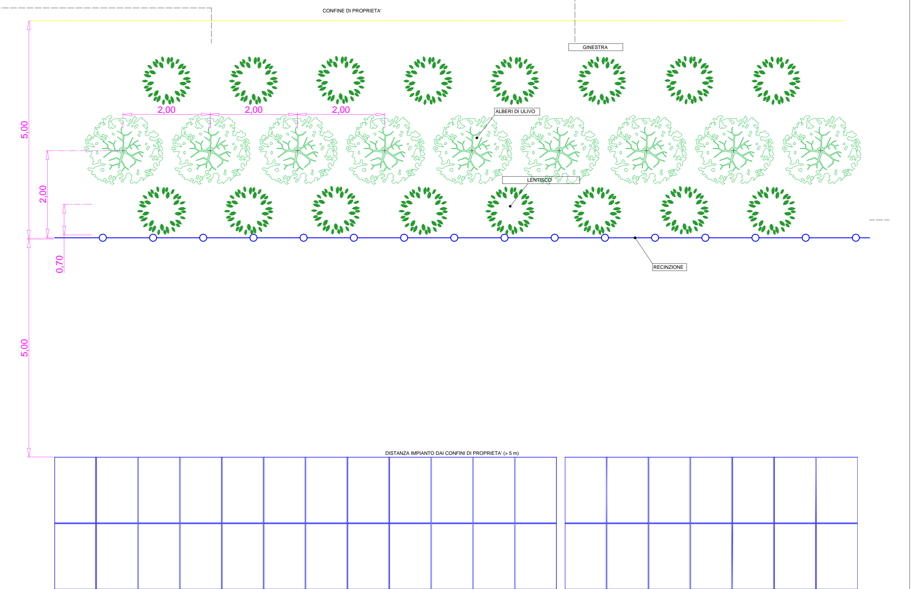
PARTICOLARE OPERE DI MITIGAZIONE - PLANIMETRIA - scala 1:20
