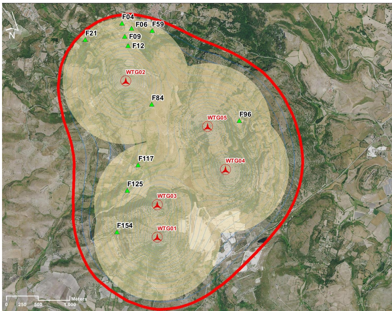
Figura 2.5 – Campo sonoro generato dall’impianto. In rosso l’isofonica dei 30 dBA, attestata ad una distanza indicativa di 1.000 m dalle postazioni eoliche in progetto
