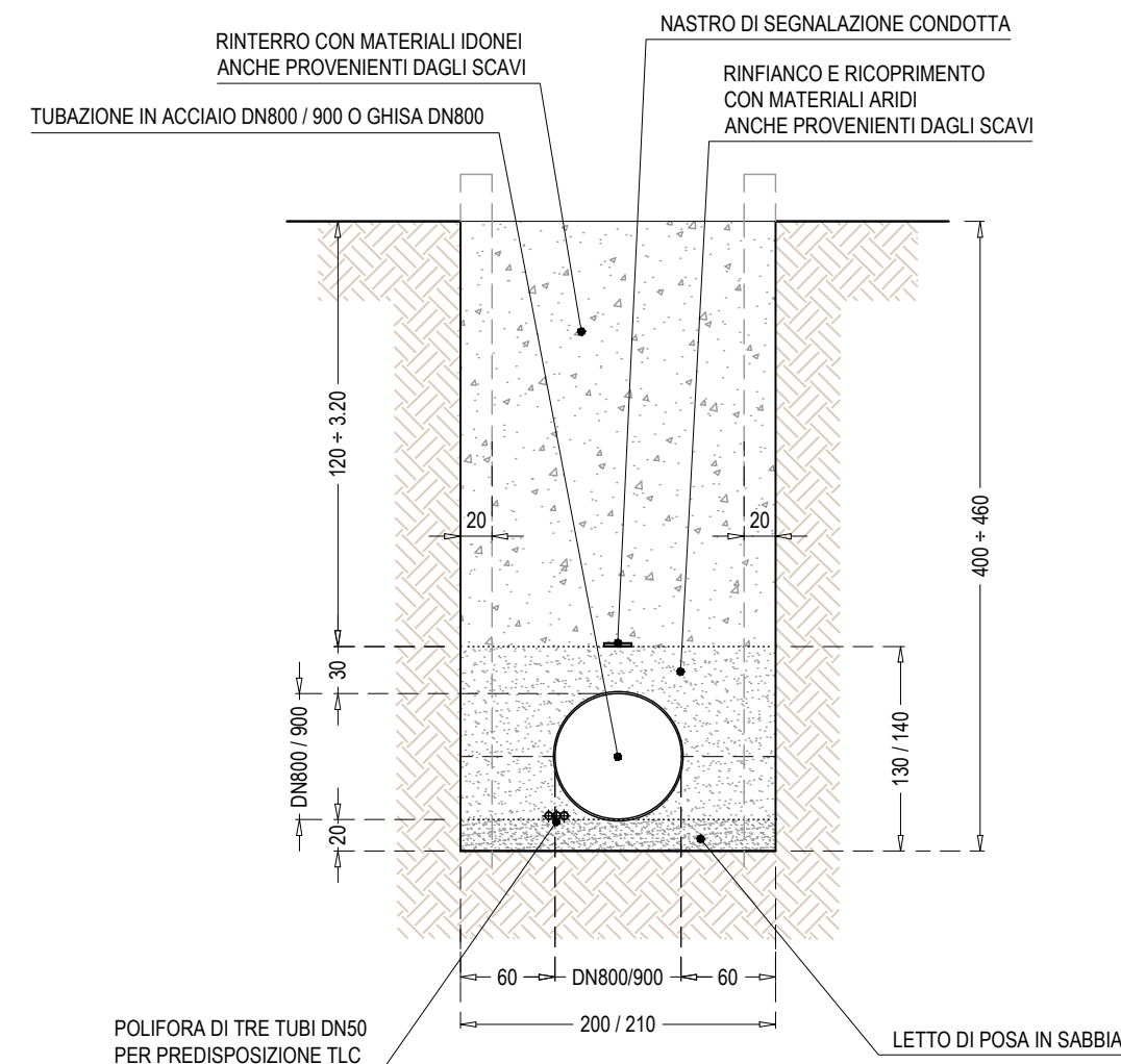
SEZIONE DI SCAVO TIPO PER TERRENI NON COESIVI O SCAVI PROFONDI Scala 1:50
