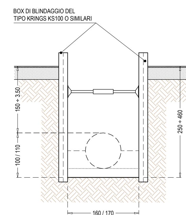
SEZIONE DI SCAVO TIPO Scala 1:50
