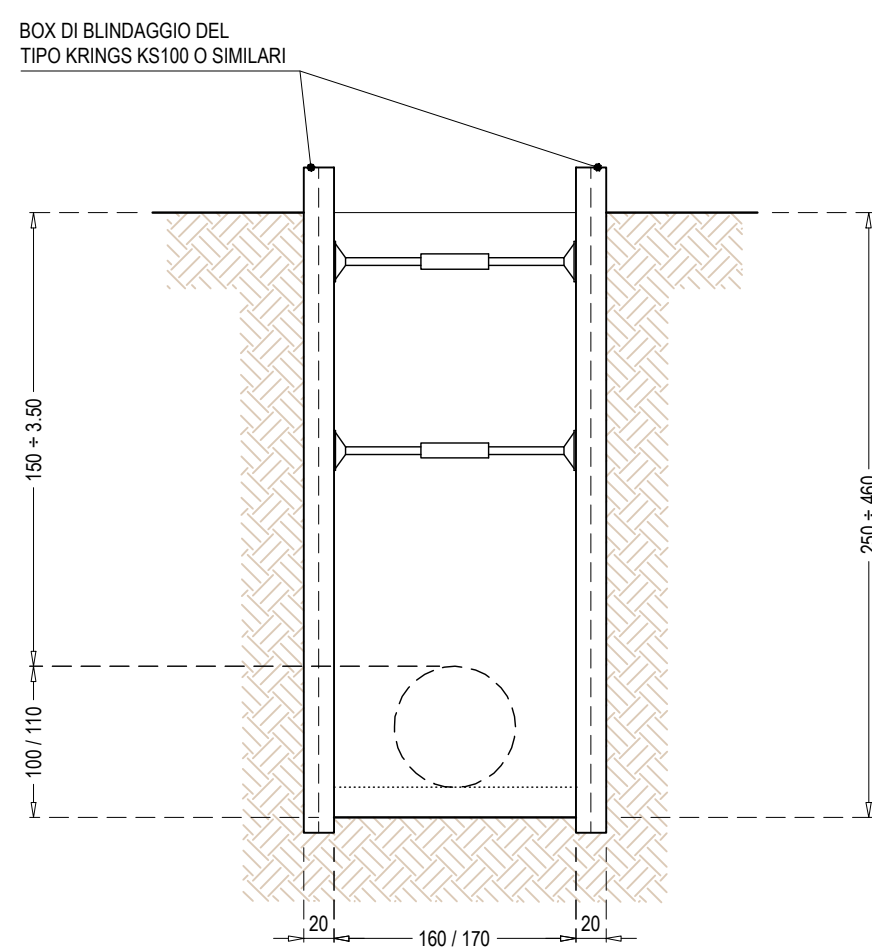
SEZIONE DI SCAVO TIPO PER TERRENI NON COESIVI O SCAVI PROFONDI Scala 1:50
