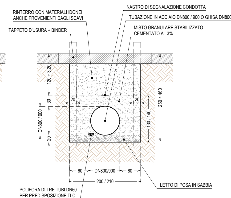
SEZIONE DI POSA TIPO Scala 1:50
