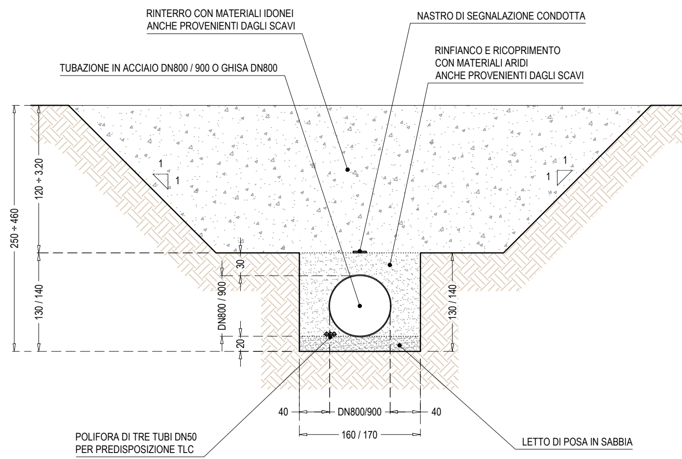
SEZIONE DI POSA TIPO PER TERRENI DEBOLMENTE COESIVI Scala 1:50
