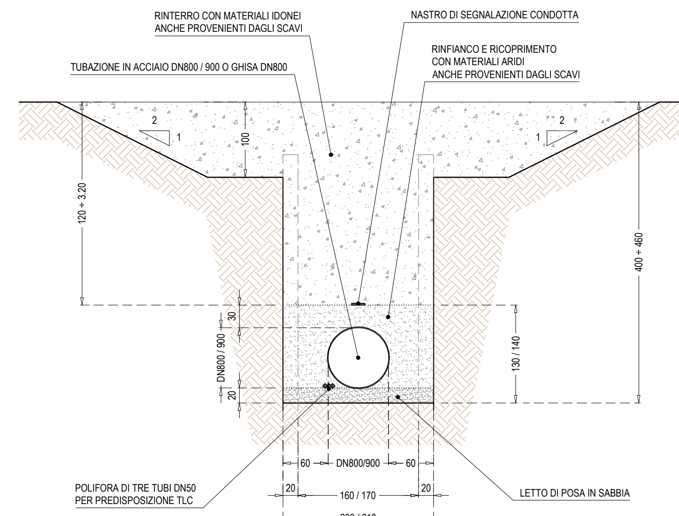
SEZIONE DI SCAVO TIPO PER TERRENI NON COESIVI O SCAVI PROFONDI Scala 1:50
