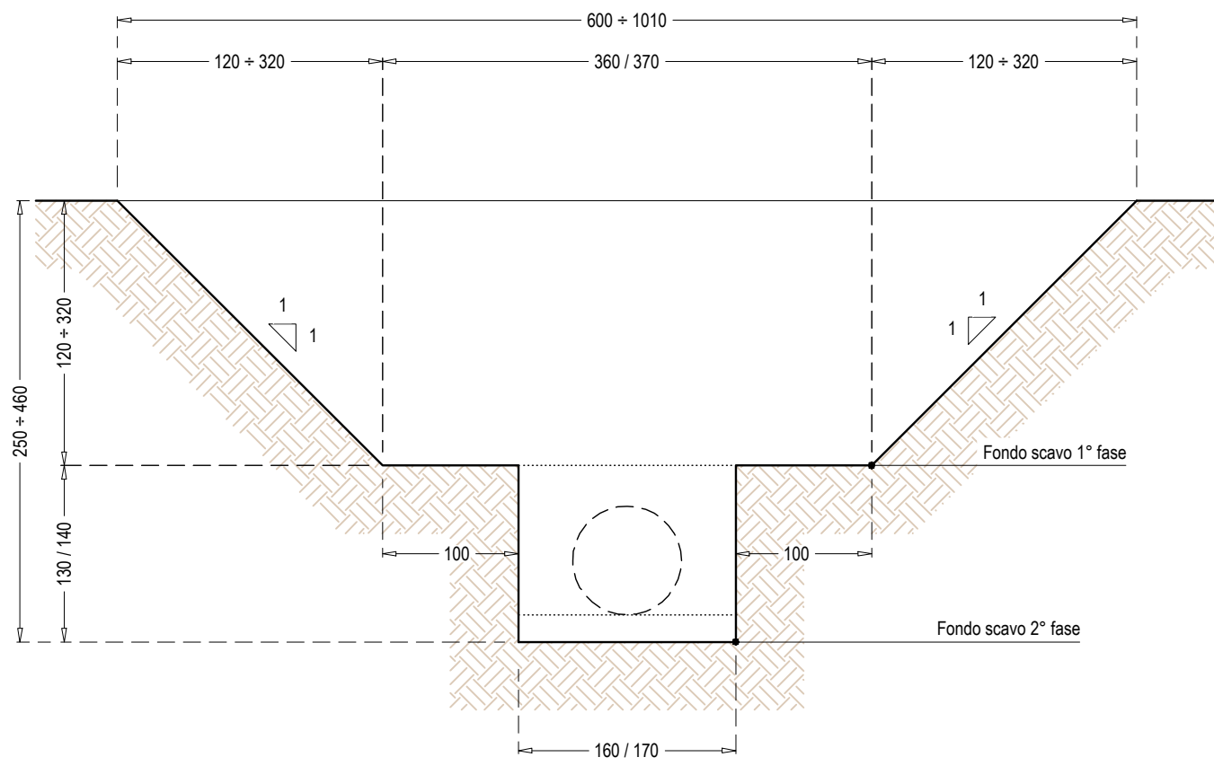
SEZIONE DI SCAVO TIPO PER TERRENI MEDIAMENTE COESIVI Scala 1:50
