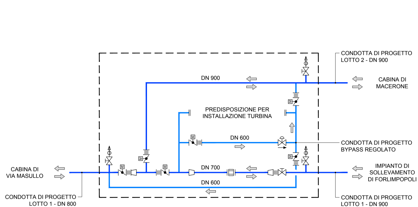
SCHEMA FUNZIONALE
