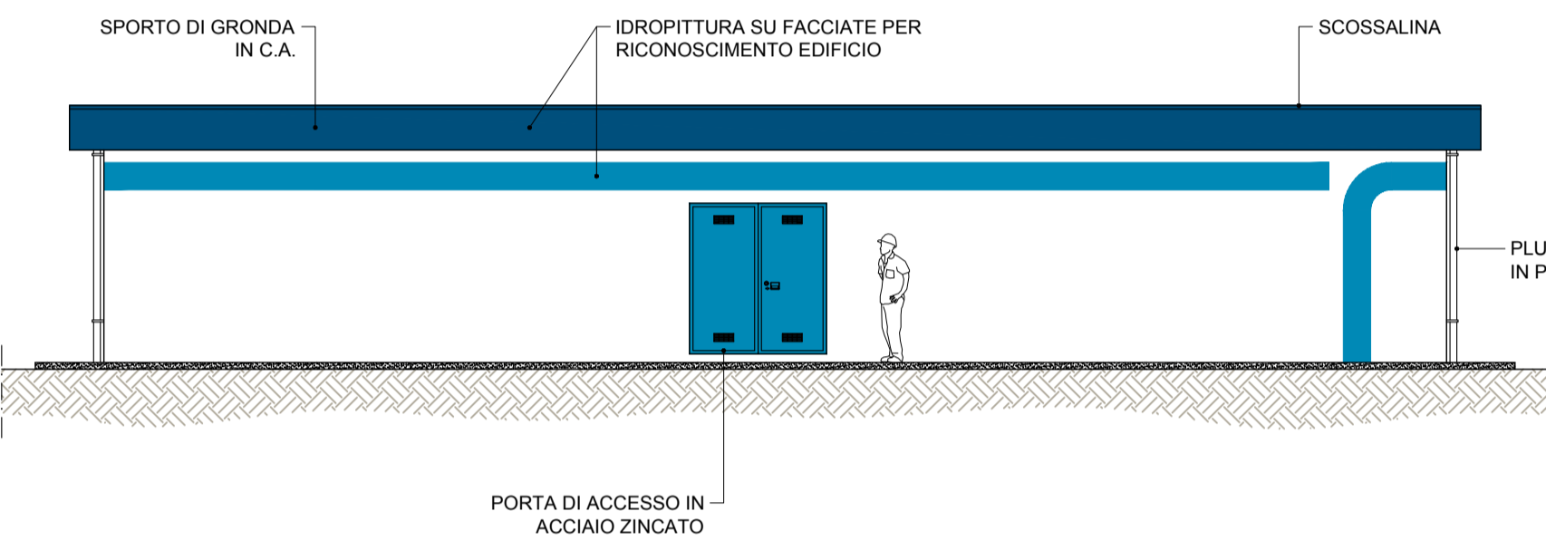
PROSPETTO FRONTALE - Scala 1:100
