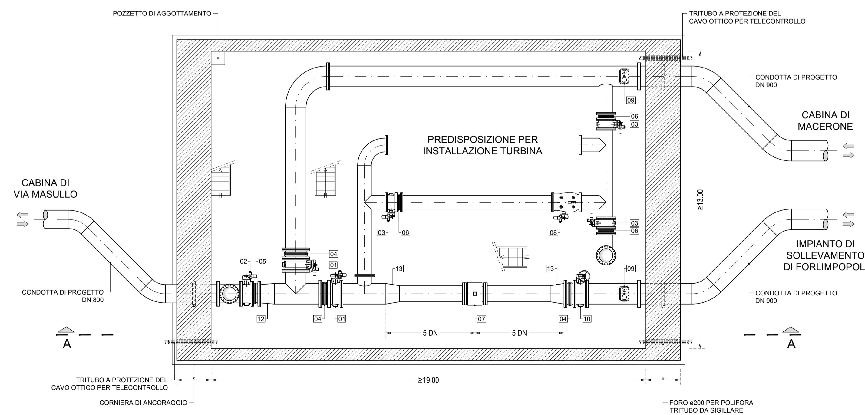
PIANTA PIANO INTERRATO - Scala 1:100
