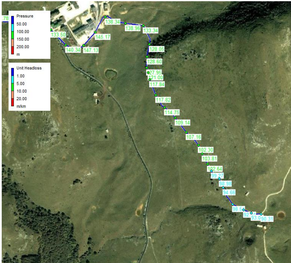
Estratto del modello idraulico.
