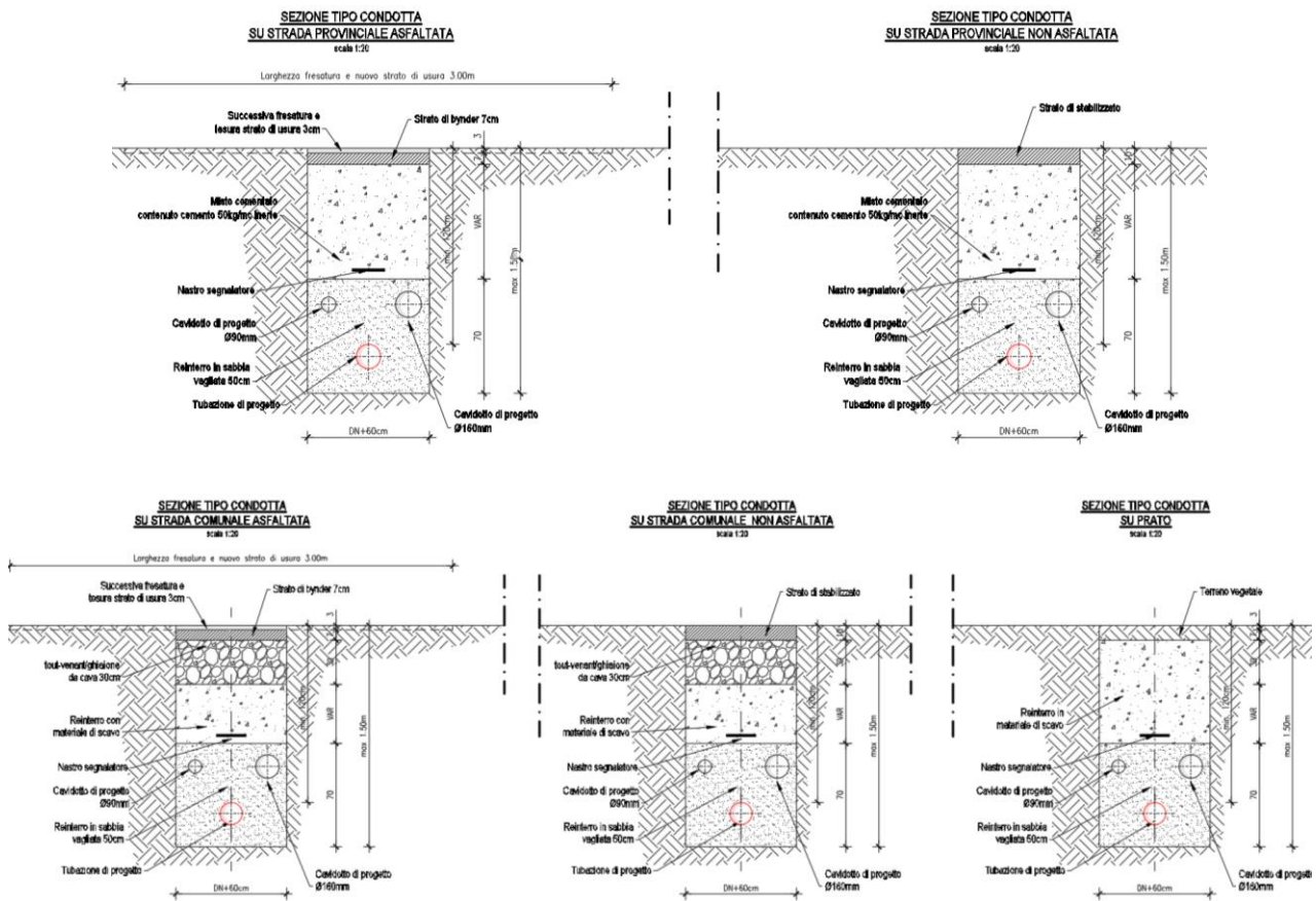
Sezioni tipologiche di posa.
