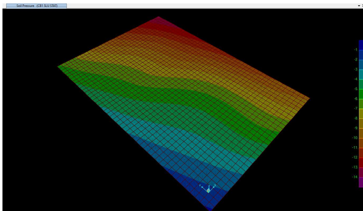
Figura 12: Pressioni del terreno
