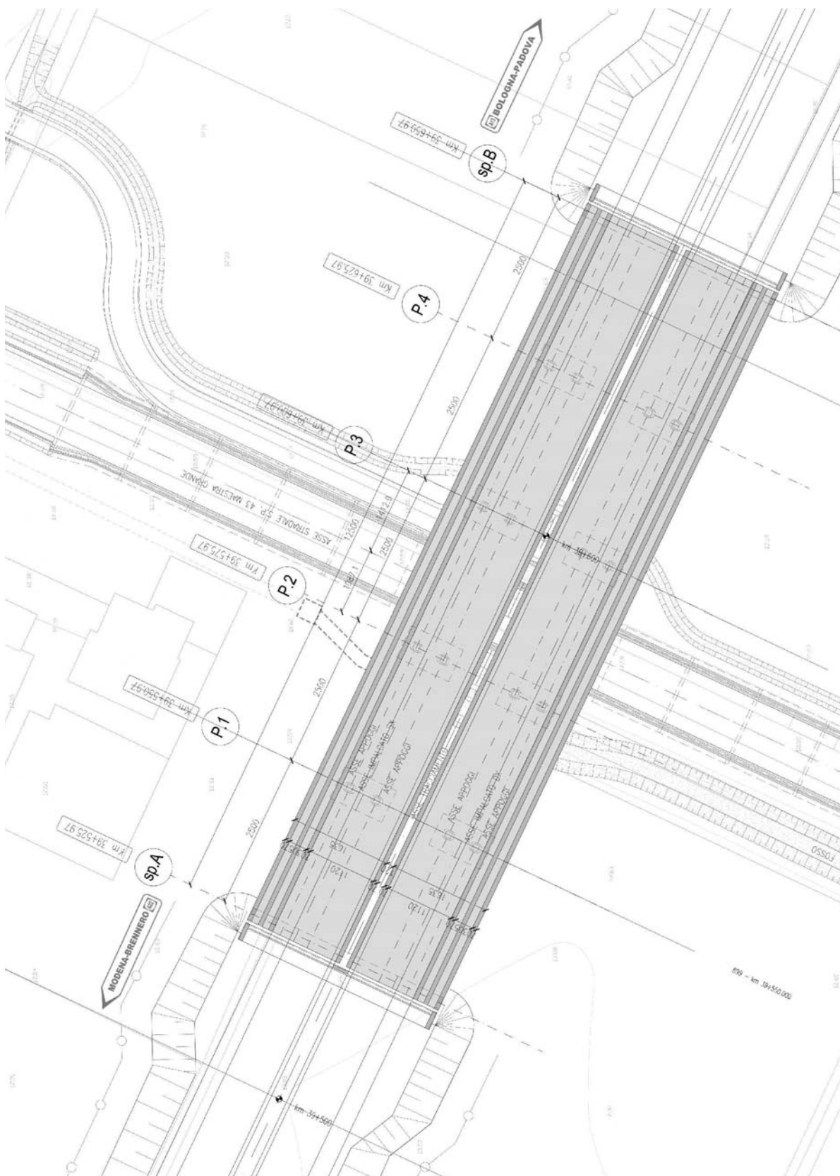
FIGURA 3-1: PLANIMETRIA.
