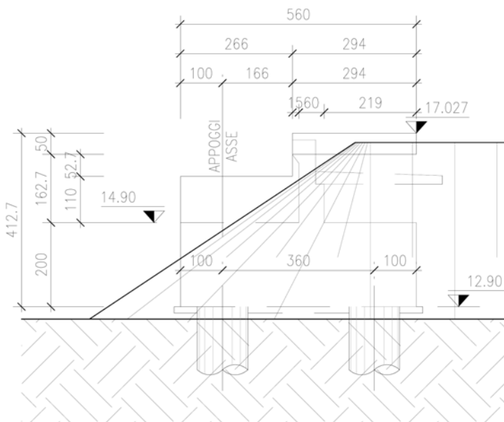
FIGURA 3-7: CARPENTERIA SPALLE.
