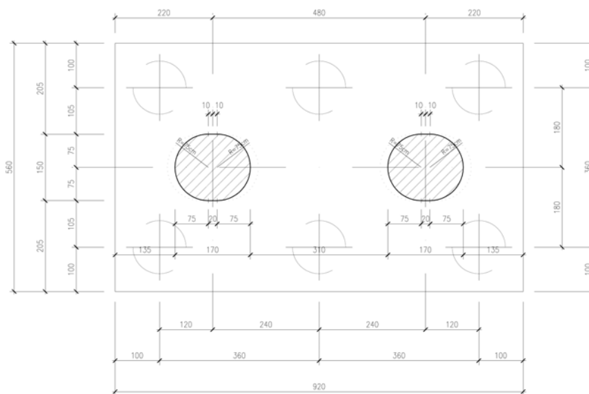
FIGURA 3-6: CARPENTERIA PILA.
