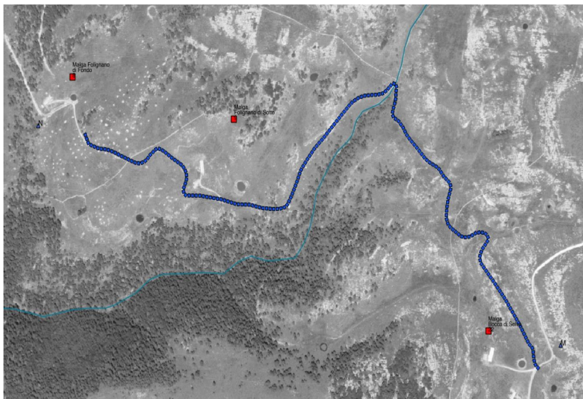
Fig. 43: tracciato di progetto su ortofoto 1988 PCN
