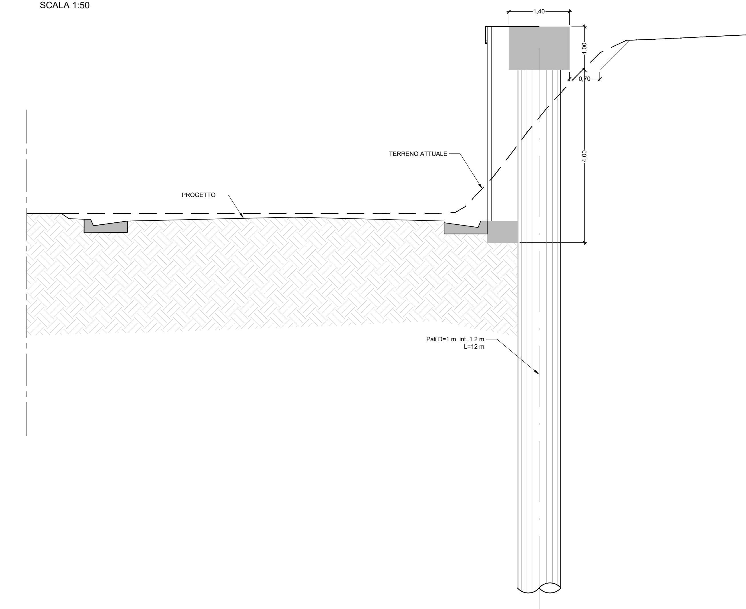
SEZIONE TIPO OS7 pk 0+025.00 SCALA 1:50
