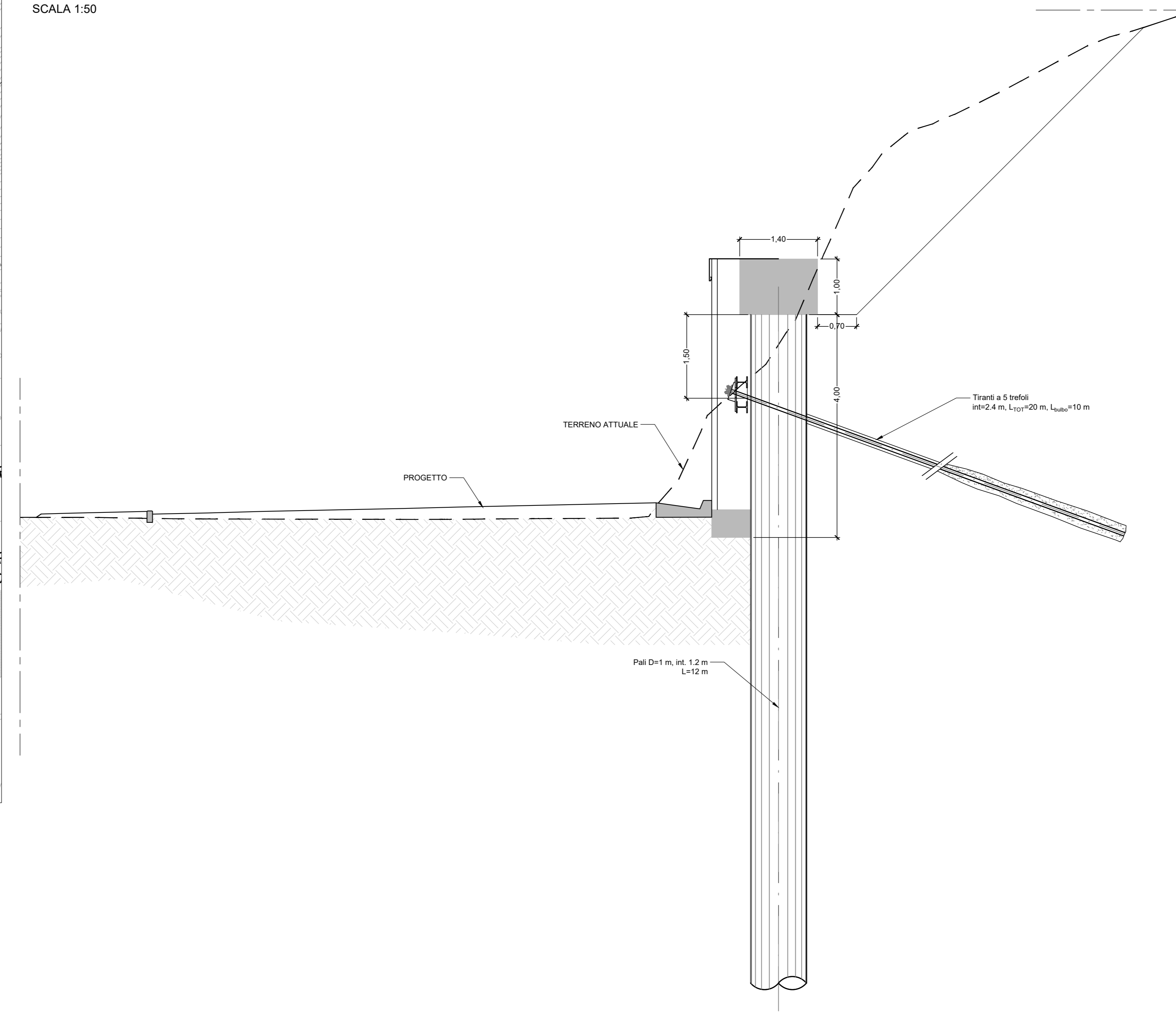
SEZIONE TIPO OS7 pk 0+0155.00 SEZIONE TIPO OS8 pk 0+0155.00 SCALA 1:50
