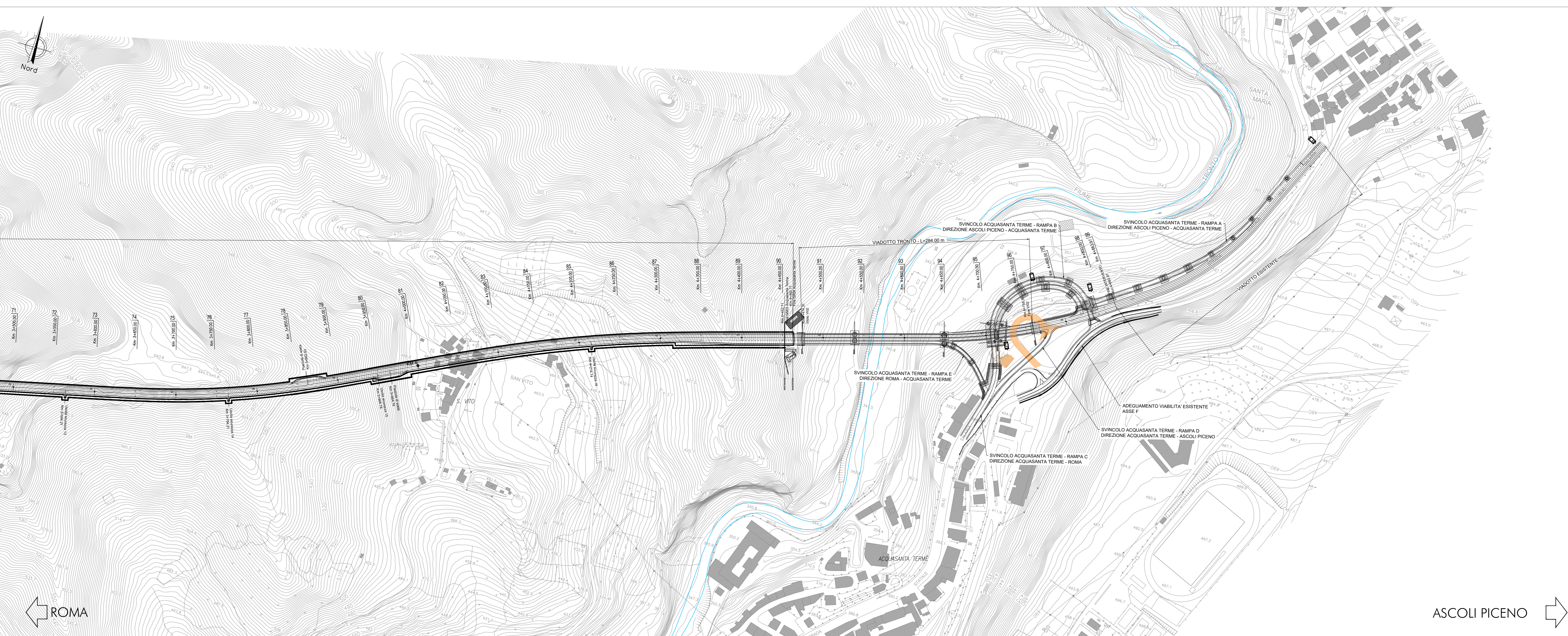
PLANIMETRIA DI PROGETTO SCALA 1:2000
