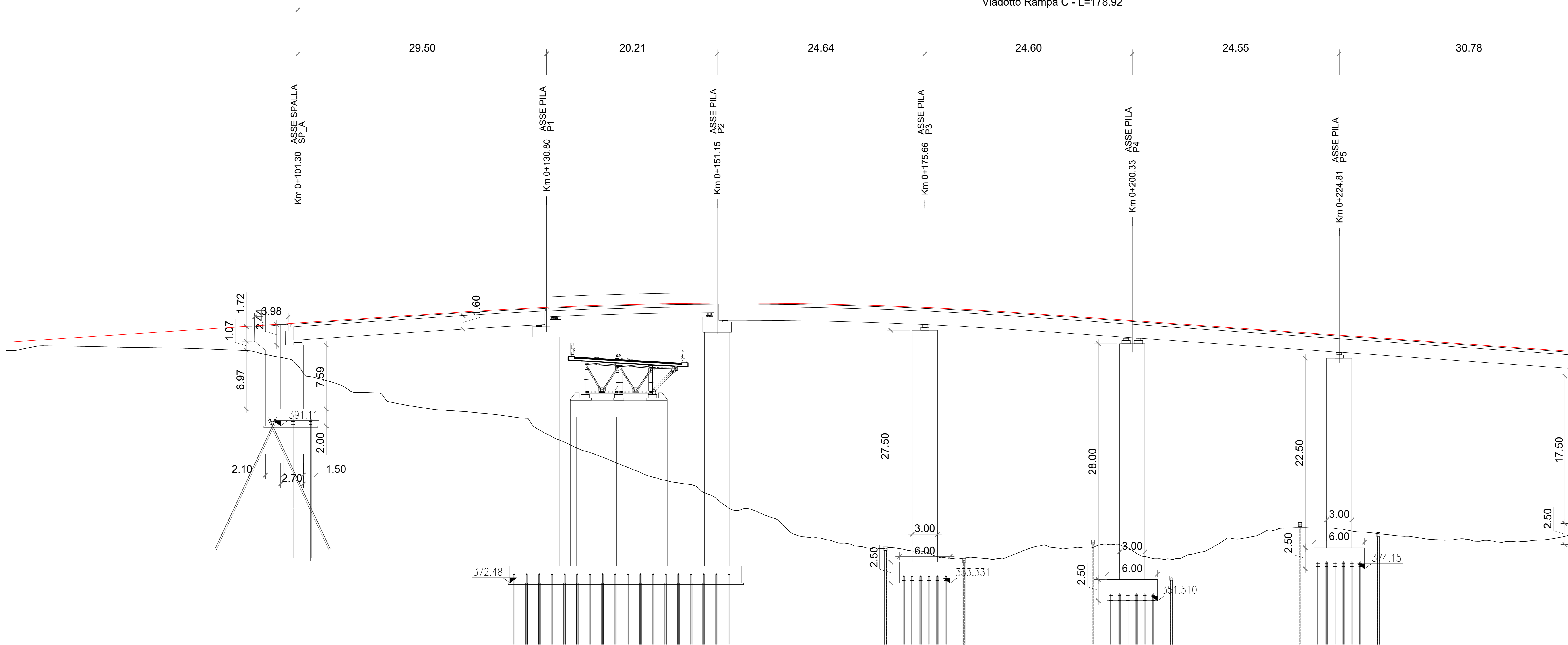
VIADOTTO RAMPA C SCALA 1:200 PROFILO LONGITUDINALE
