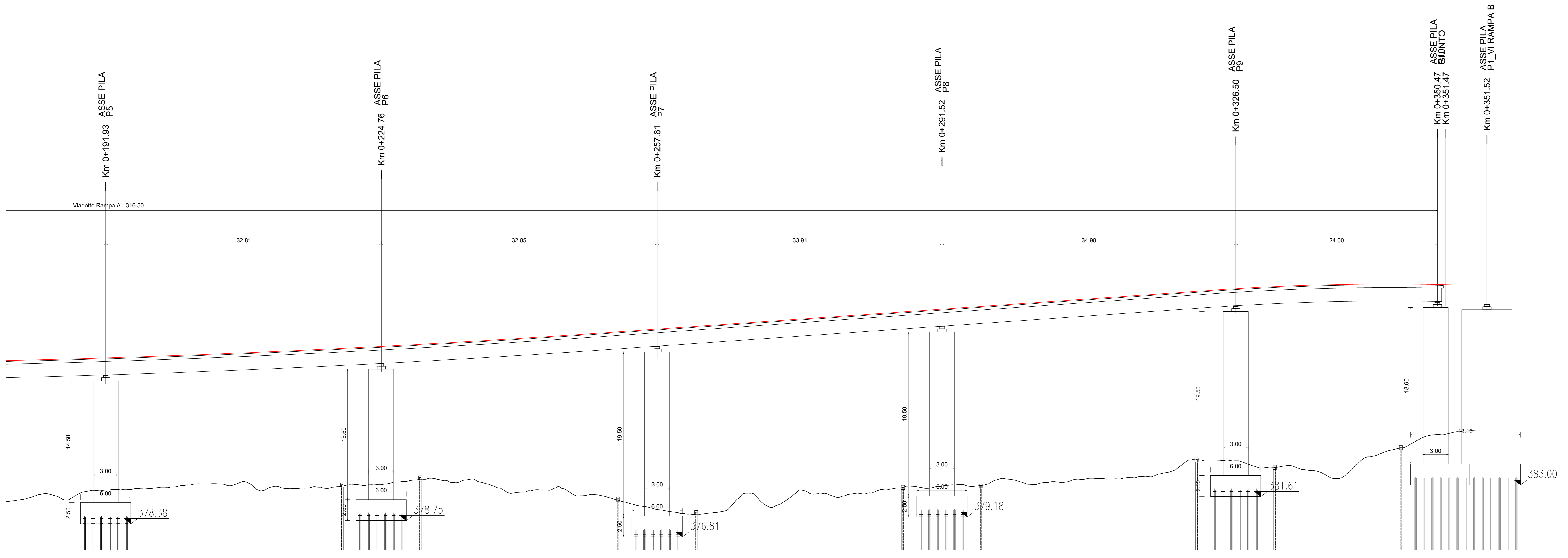
VIADOTTO RAMPA A SCALA 1:200 PROFILO LONGITUDINALE
