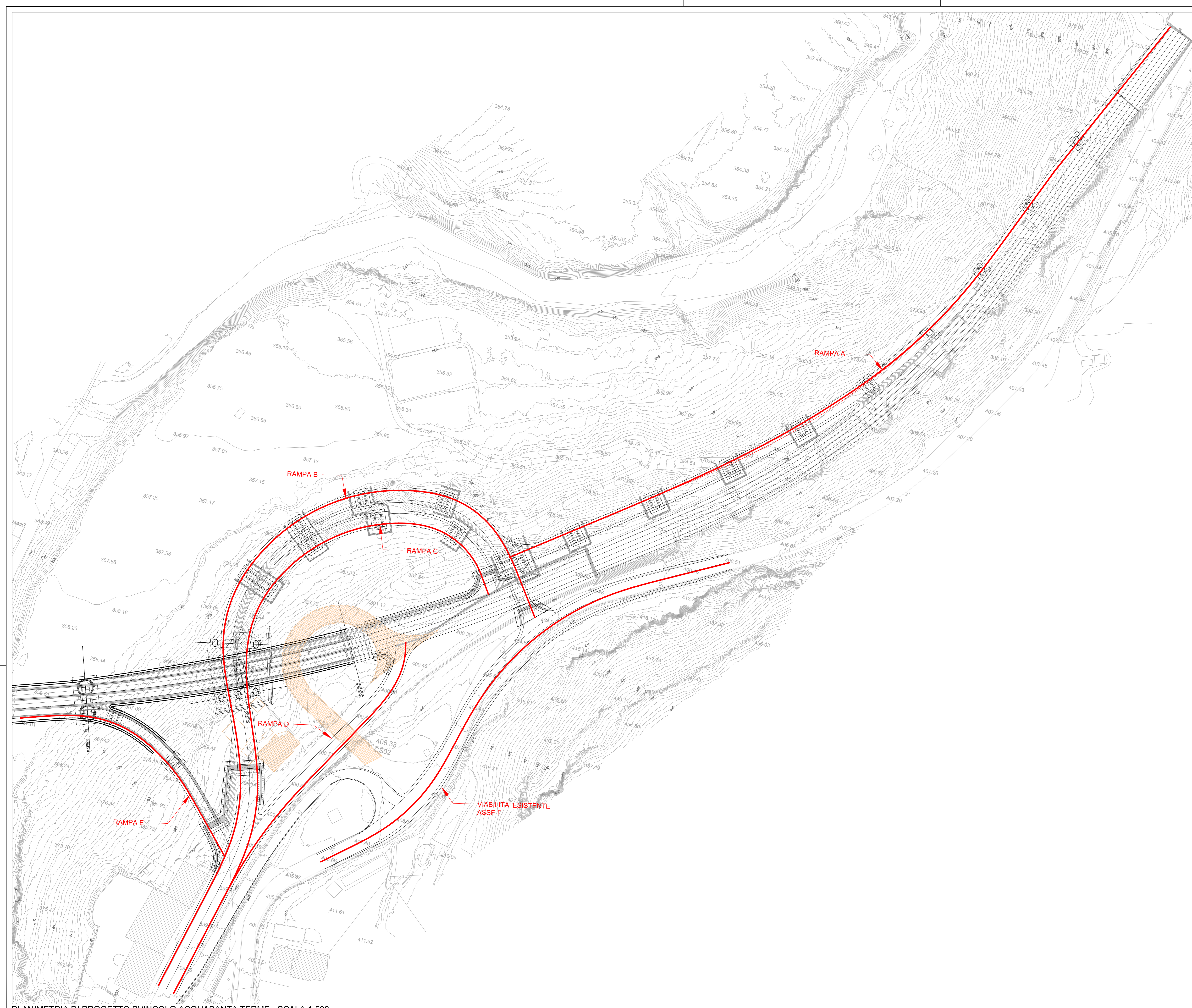
PLANIMETRIA DI PROGETTO SVINCOLO ACQUASANTA TERME - SCALA 1:500
